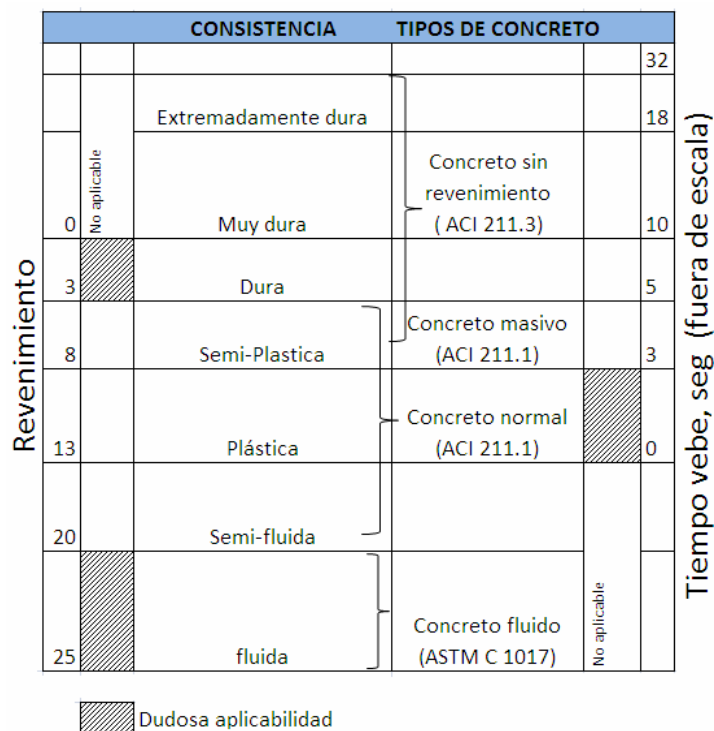
Fig. 4.6 Gráfica de consistencia del concreto
