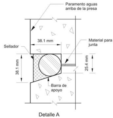
6.10 Sello de junta de contracción en la cara aguas arriba
