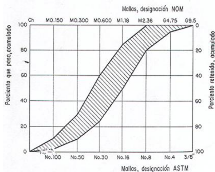
Fig. 2.7 Límites granulométricos especificados para la arena
