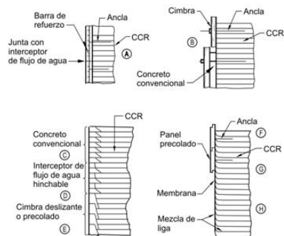
6.11 Opciones para el revestimiento aguas arriba
