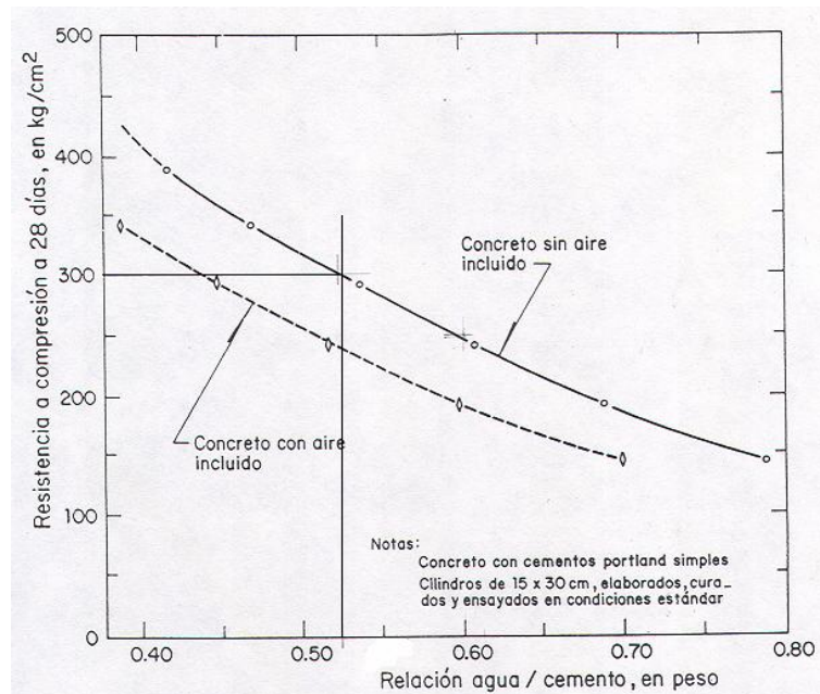
Fig. 4.4 Curva resistencia a compresión predicable en el concreto a 28 días de edad, de acuerdo con la relación agua/cemento en el ACI 211.1.
