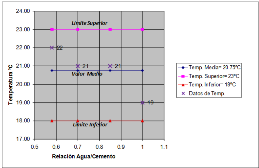
Fig. 5.2 Carta control de temperatura del CCR realizado con cemento CPO 30R.
