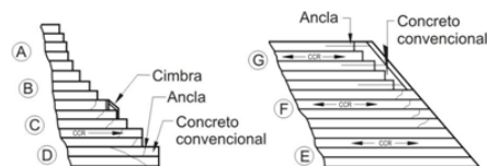
6.12 Opciones para el revestimiento aguas abajo
