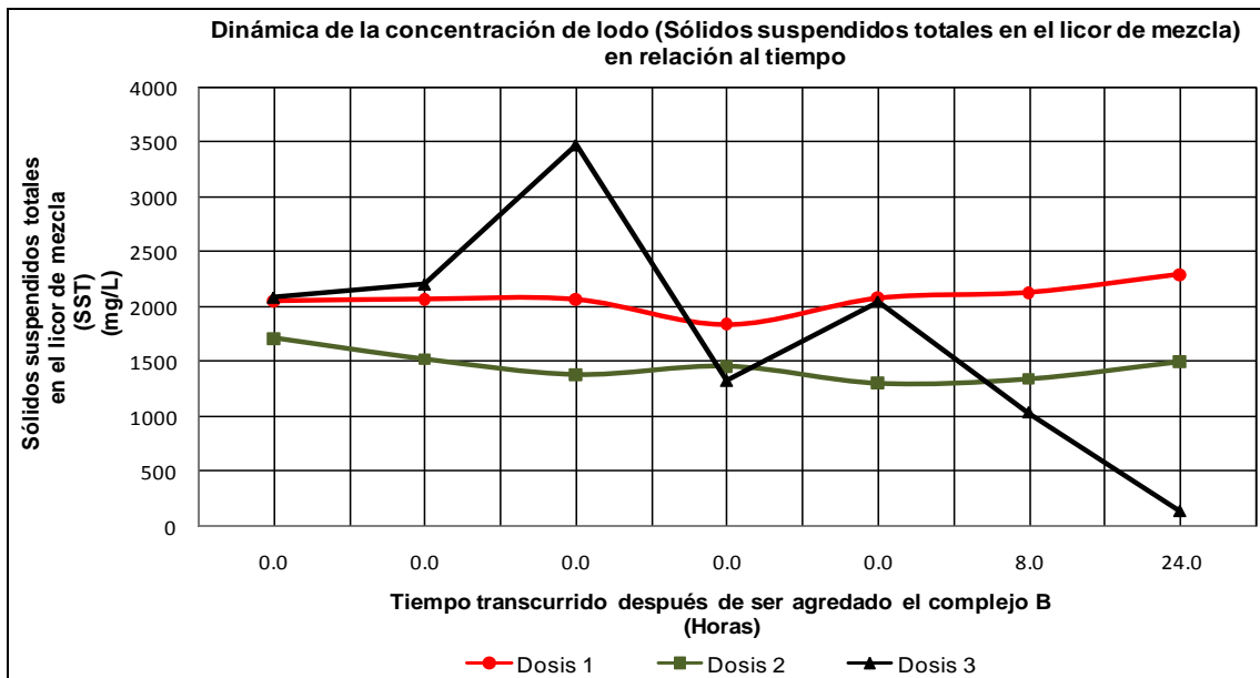
Fig. 5.7 Dinámica de la concentración de lodo, correspondiente a la repetición 1.
