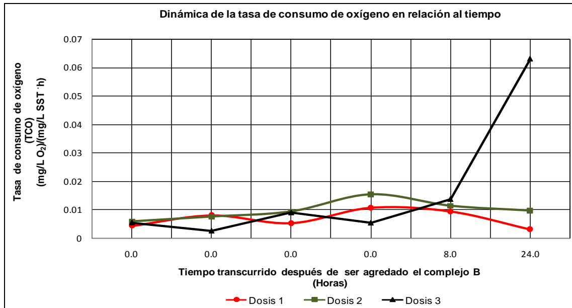
Fig. 5.13 Dinámica de la tasa de consumo de oxígeno correspondiente a la repetición 1.
