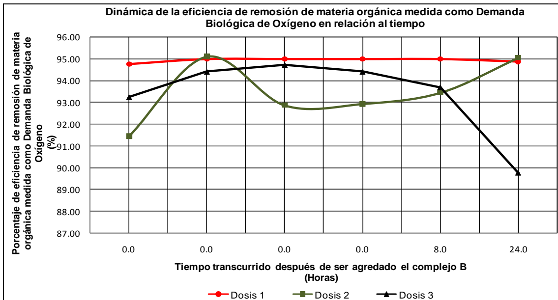
Fig. 5.11 Dinámica de la eficiencia de remoción de materia orgánica medida como demanda biológica de oxígeno, correspondiente a la repetición 1.
