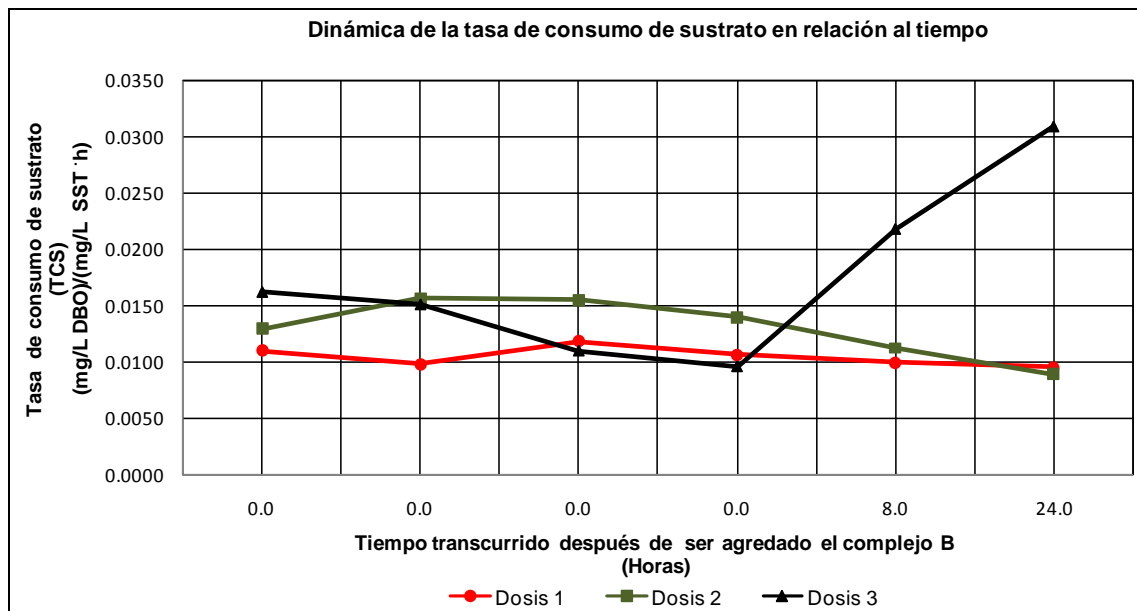
Fig. 5.16 Dinámica de la tasa de consumo de sustrato correspondiente a la repetición 2.
