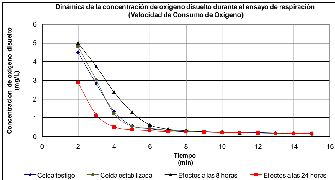
Fig. 5.1 Dinámica de la concentración de oxígeno disuelto durante el ensayo de respiración correspondiente a la dosis 1 de complejo B, repetición 1.
