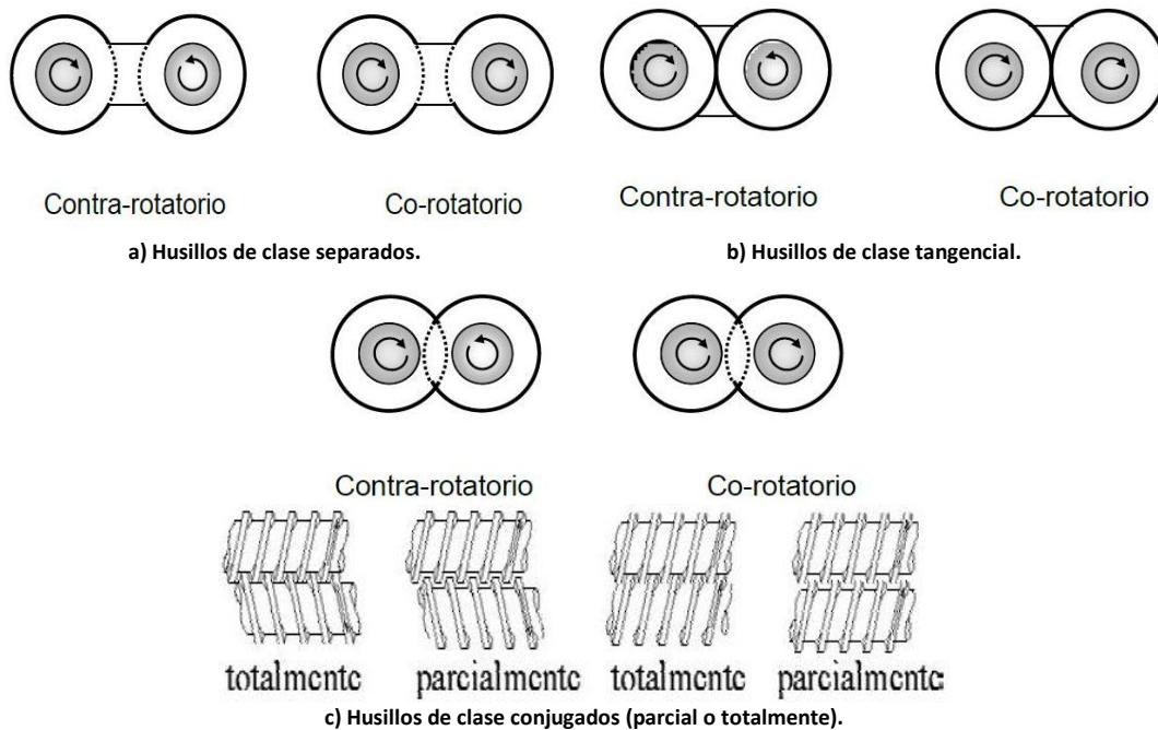
Figura 2.11.2.a. Clasificación de los tornillos de acuerdo al contacto 52 .
