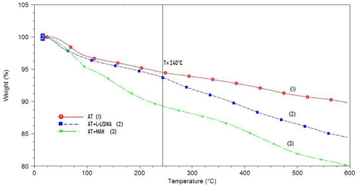
Figura 4.2.1.a. TGA de la arcilla atapulgitica (1) modificada químicamente con MAH (3) y L-lisina (2).
