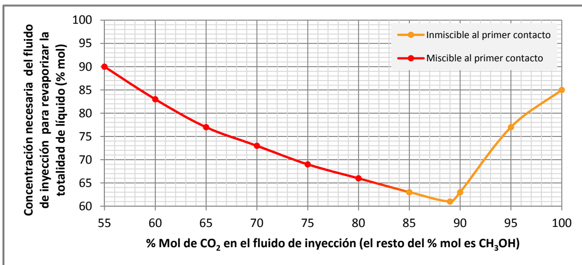
Figura 5.5 Diferentes proporciones de la mezcla de inyección CO 2 +CH 3 OH, y concentraciones necesarias para reevaporizar la totalidad de líquido condensado a 316.38 kg/cm 2 y temperatura de yacimiento (177 °C).
