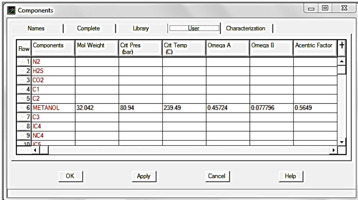
Figura 4.7 Definición del peso molecular, presión crítica, temperatura crítica y factor acéntrico del metanol en el simulador.
