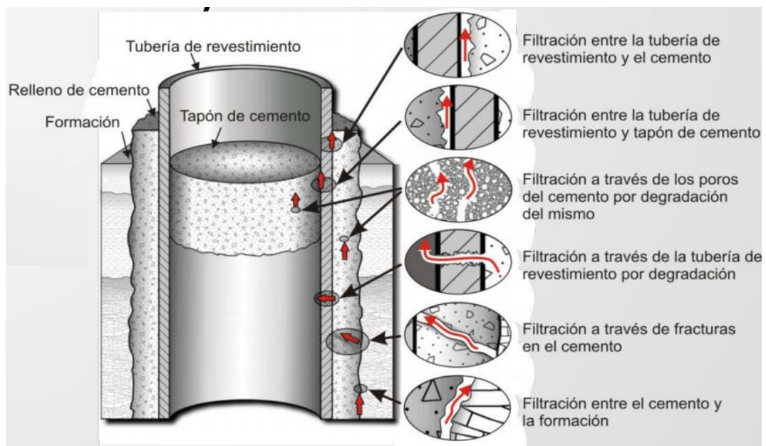
Figura 2. 5 Posibles fugas del fluido fracturante en la tubería de un pozo no convencional (Sánchez, 2012).
