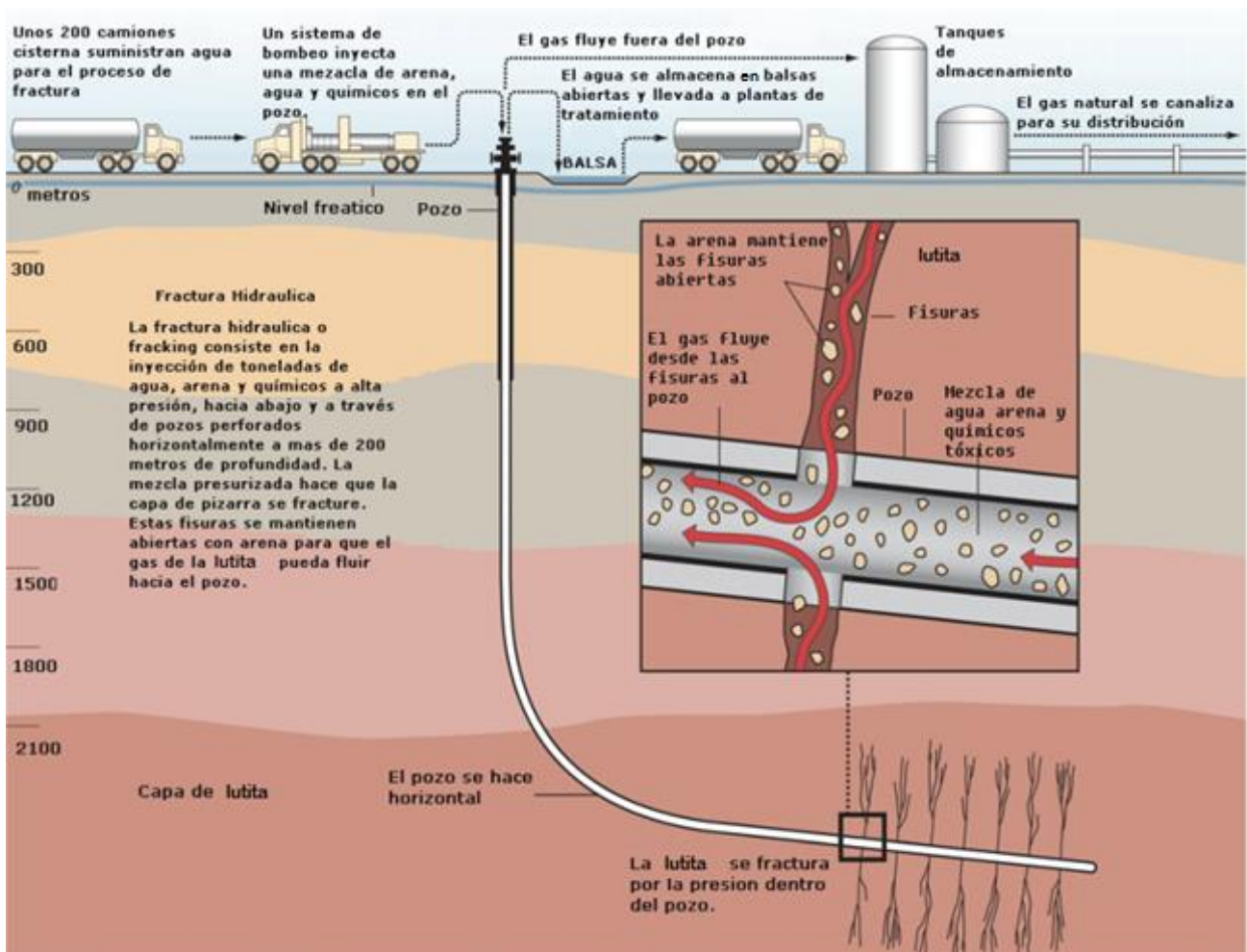
Figura 2. 2 Imagen de los procesos realizados en superficie de un yacimiento de Shale Gas y del movimiento del fluido fracturante en la formación (Asamblea contra la Fractura Hidráulica, 2011).
