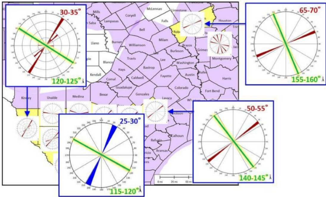
Figura 2. 9 Orientación de la configuración óptima de pozos (mostrada en color verde) para cada una de las tres áreas dentro del play Eagle Ford (Telker, 2013).
