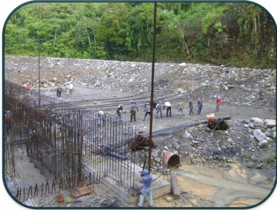
FOTOGRAFIA No.67.-La mayor parte de la colocación de acero se apoyó con la grúa pero en otros elementos no se pudo por el detalle que se entrelazaban parrillas con parrillas.
