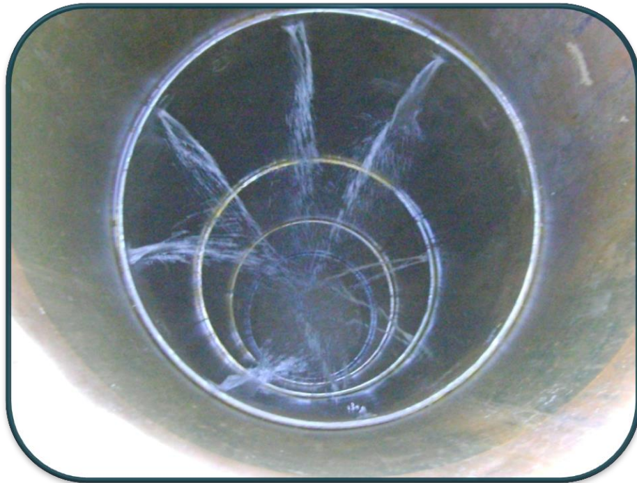
FOTOGRAFIA No.18.-Por el nivel freático la presión de agua se filtraba por las uniones del ademe y eso podría provocar al momento del colado un lavado del concreto y resultaría ineficiente el pilote en estudio.
