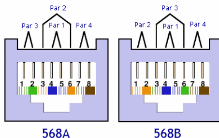
Figura 2.2. Asignación de pines para el conector del cable UTP
