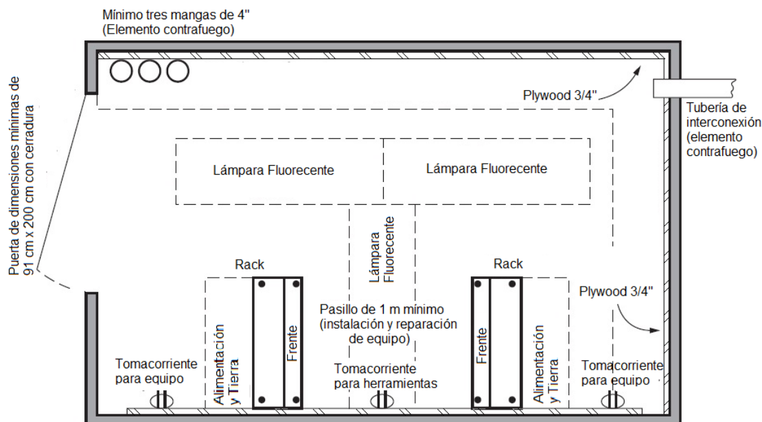
Figura 2.14. Cuarto de telecomunicaciones.
