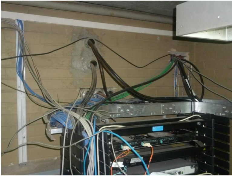
Figura 3.6. Canalizaciones en el SITE.
