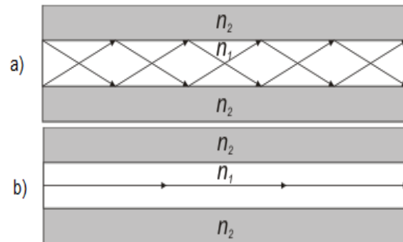
Figura 1.11. a) Modo de propagación de la luz óptica multimodo. b) Modo de propagación de la luz en una fibra óptica monomodo
