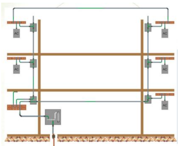
Figura 2.25. Sistema de Puesta a Tierra.
