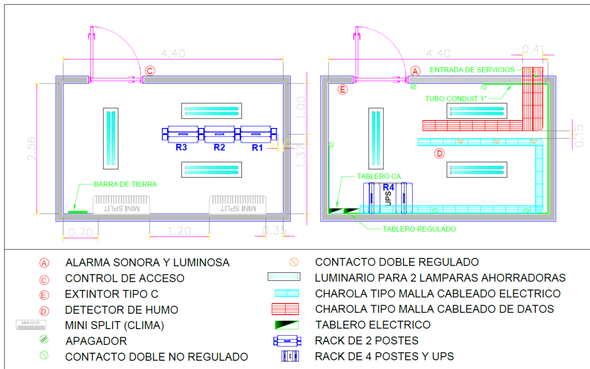
Figura 4.3. Distribución de equipo en el cuarto de telecomunicaciones principal.
