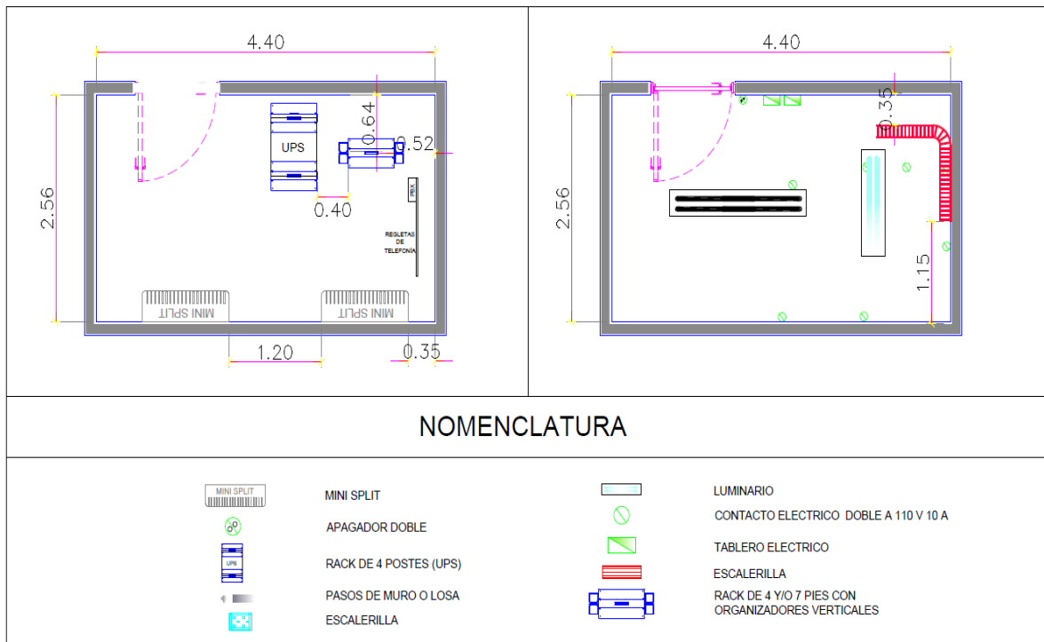
Figura 3.7. Distribución de equipos.
