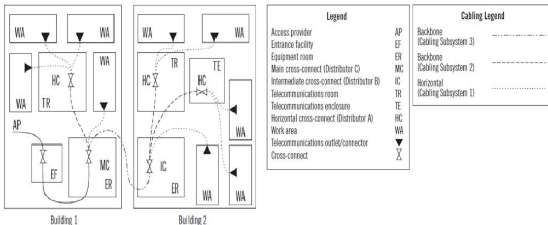
Figura 2.3. Modelo del sistema de cableado de telecomunicaciones en un edificio comercial
