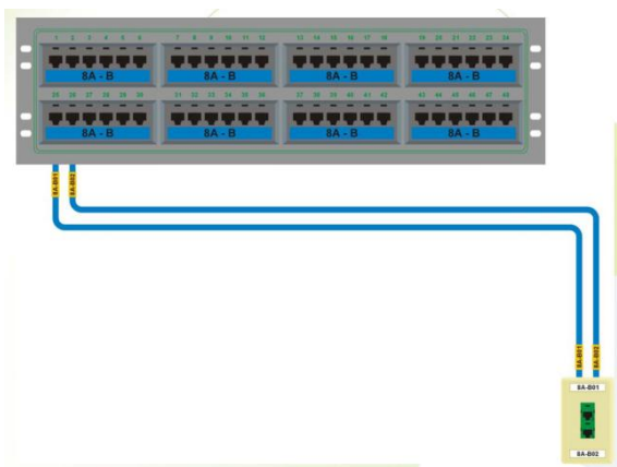
Figura 2.19. Canal de telecomunicaciones.
