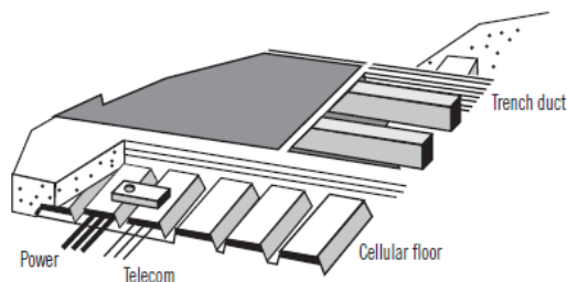
Figura 2.8. Canalización bajo piso.
