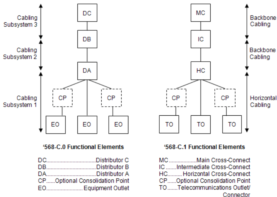
Figura 2.1. Comparación de la terminología de los elementos funcionales para 568-C.0 y 568-C.1
