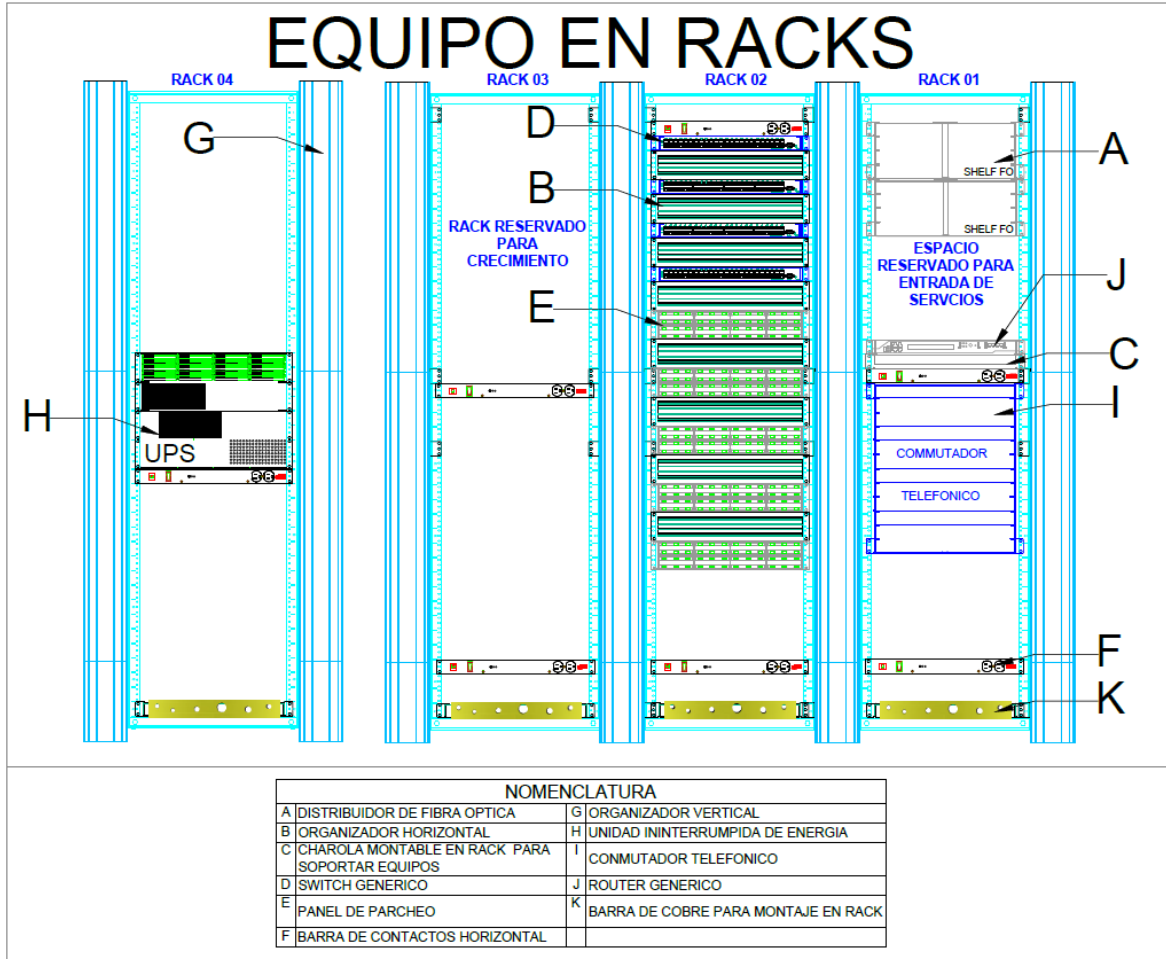
Figura 4.4. Frentes de rack's del SITE.
