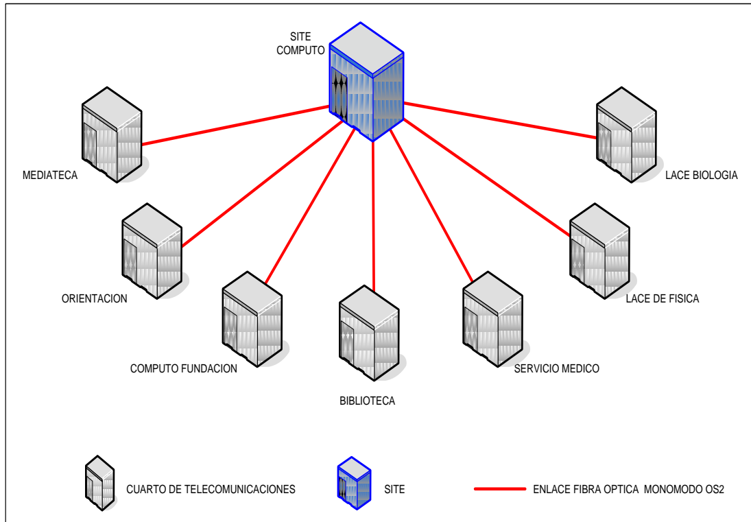
Figura 4.7. Enlaces de cableado de backbone o vertical.
