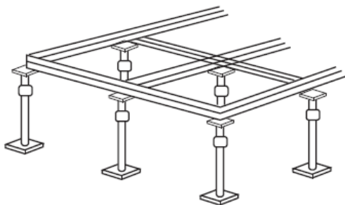
Figura 2.9. Canalización bajo piso elevado.
