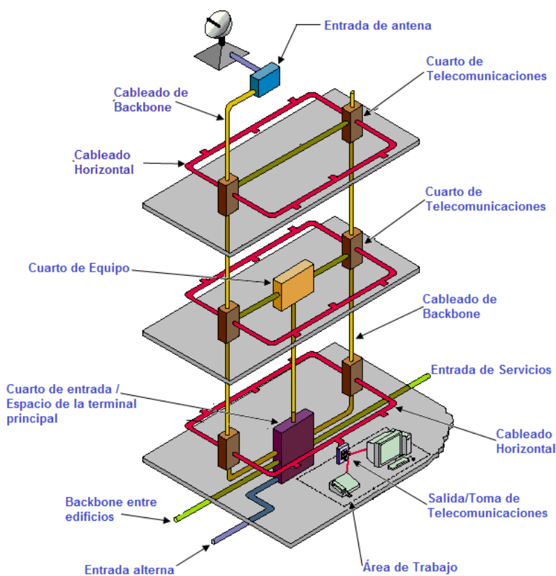
Figura 2.4. Modelo del sistema de cableado de telecomunicaciones en un edificio comercial
