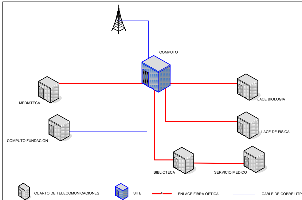
Figura 3.14. Distribución del cableado de backbone en ENP plantel No. 6.
