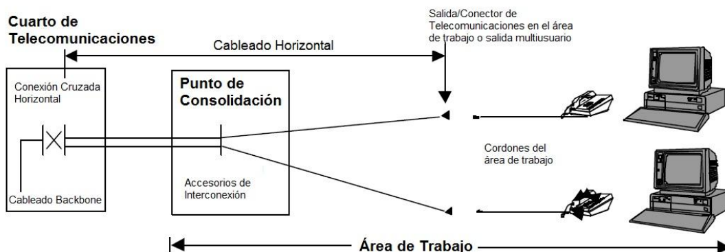
Figura 2.6. Punto de consolidación.
