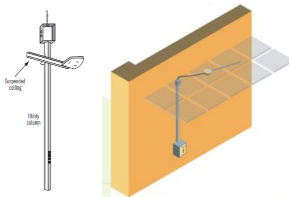
Figura 2.11. Cableado sobre techo falso.
