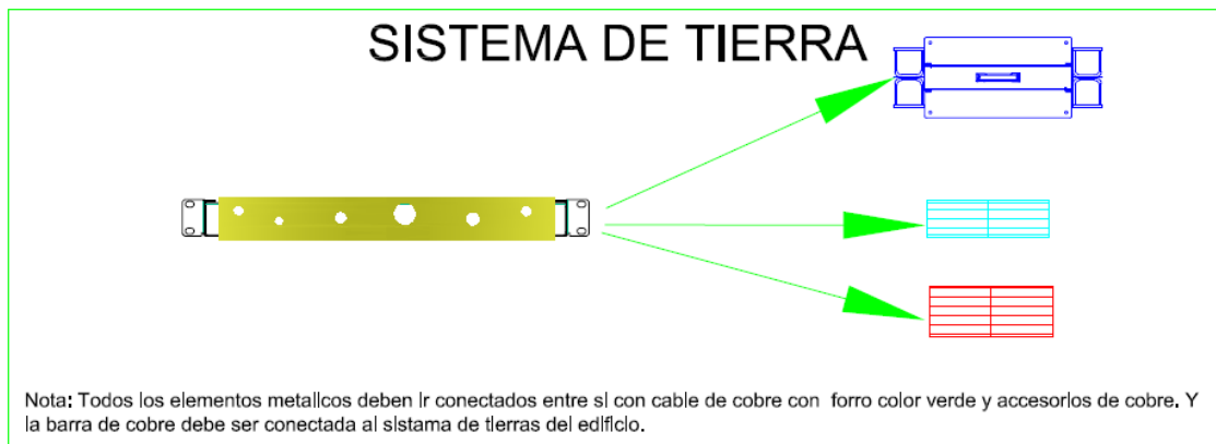
Figura 4.2. Sistema de tierra.
