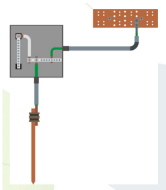
Figura 2.23. Unión de la TMGB con la tierra del Sistema de Potencia.
