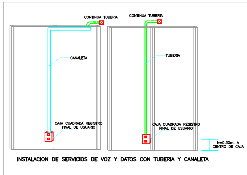
Figura 4.6. Salidas en Área de Trabajo.
