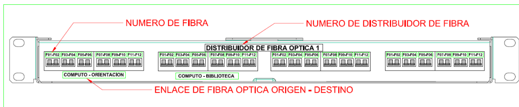
Figura 4.10. Etiqueta para distribuidor de fibra óptica.
