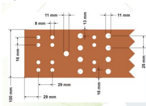
Figura 2.24. Dimensiones típicas de una barra de Cobre para Telecomunicaciones.
