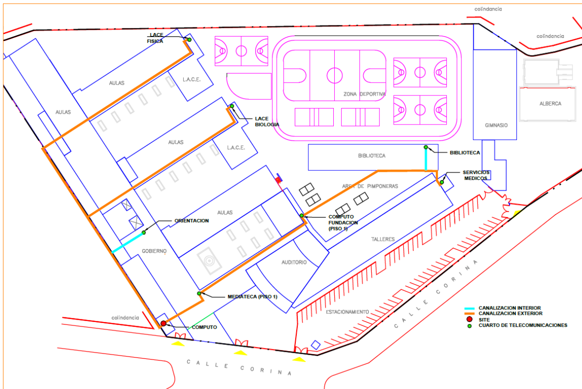
Figura 4.5. Ubicación de cuartos de telecomunicaciones.
