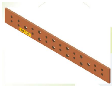
Figura 2.22. La TMGB debe de ir etiquetada.
