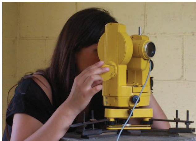
Figura. 3.1.27. Teodolito DI-FLUX ZEISS A-20 cuasi-nivelado con el sensor Fluxgate en dirección hacia-abajo.
