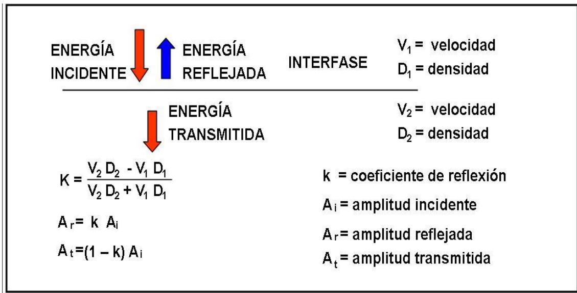
Fig. 5.5 Relación de incidencia, onda reflejada y transmitida a través de una interfase
