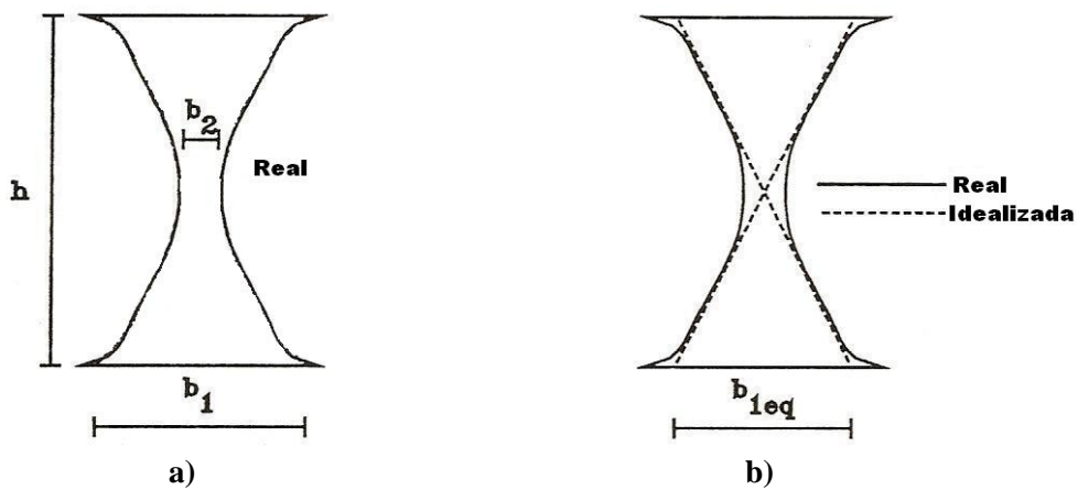
a) b) Figuras 3.3. Geometría real e idealizada de los dispositivos ADAS
