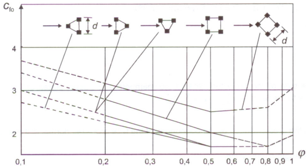
Figura 5.15. Coeficiente de fuerza C_{f,0} para una estructura con celosías espaciales con miembros angulares, en función del factor de solidez \varphi (Referencia 5).
