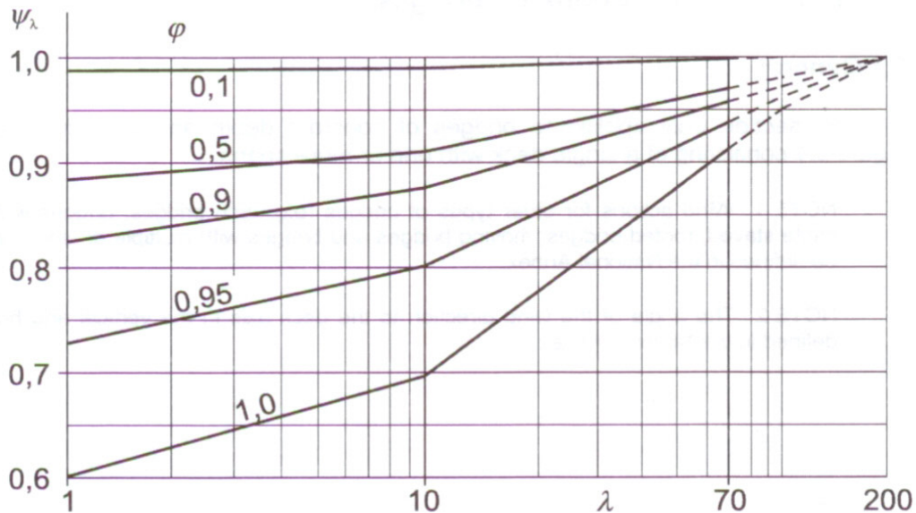
Figura 5.16. Valor indicativo del factor de efecto de fondo \psi_\lambda , en función del factor de solidez \phi contra la esbeltez \lambda (Referencia 5).
