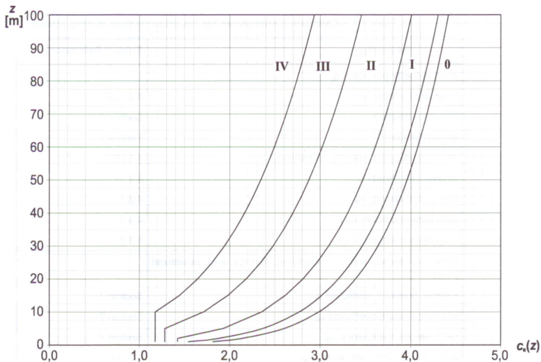
Figura 5.12. Factor de exposición C_e(Z) para C_o = 1.00 y k_r = 1.00 (Referencia 5).
