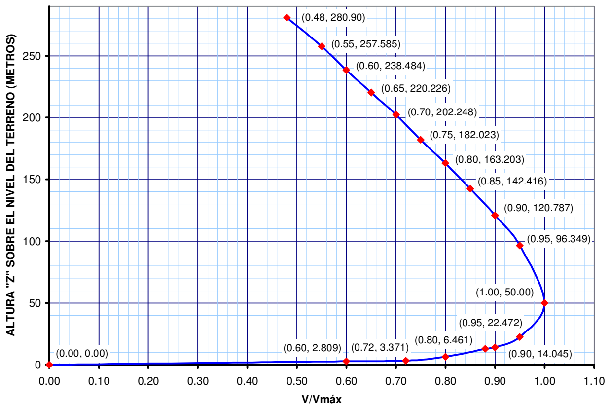
Figura 3.2. Perfil promedio de variación de la velocidad del viento con la altura durante una tormenta severa o vaguada (Referencia 15).
