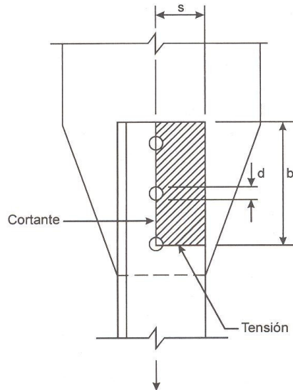
Figura 6.4. Superficies de falla por cortante y tensión combinados (Referencia 4).
