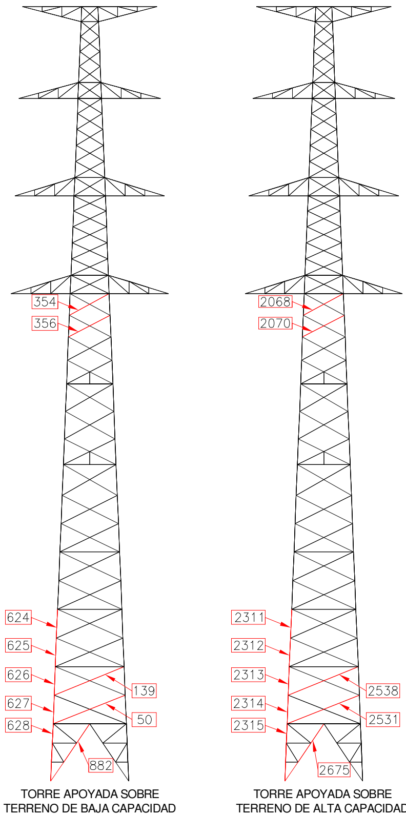
Figura 8.1. Elementos revisados para cada una de las torres de soporte.
