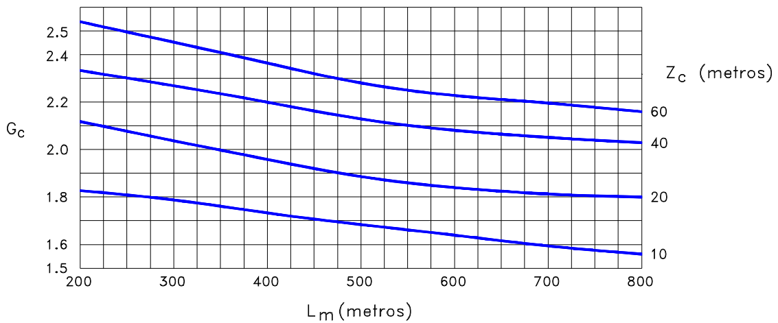
Figura 5.8. Factor de ráfaga para conductores, terreno de rugosidad B (Referencia 2).
