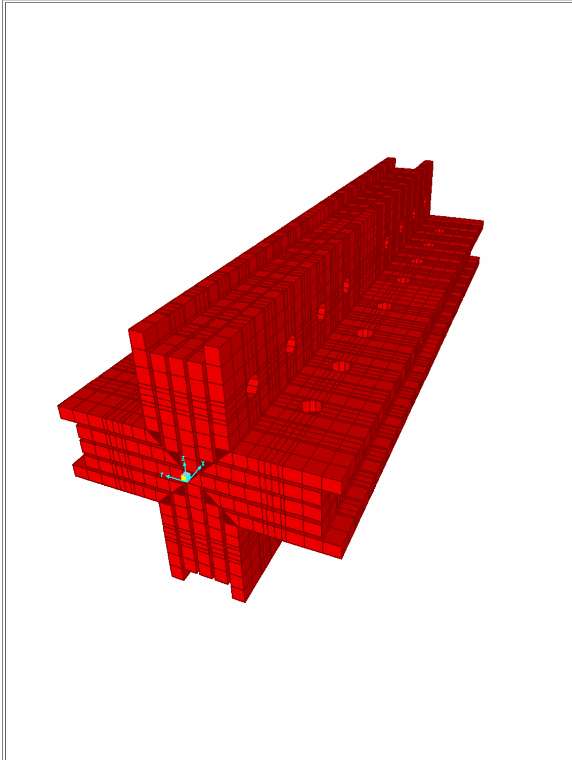
Figura A.3. Modelo completo con elementos finitos sólidos de la conexión en estudio.
