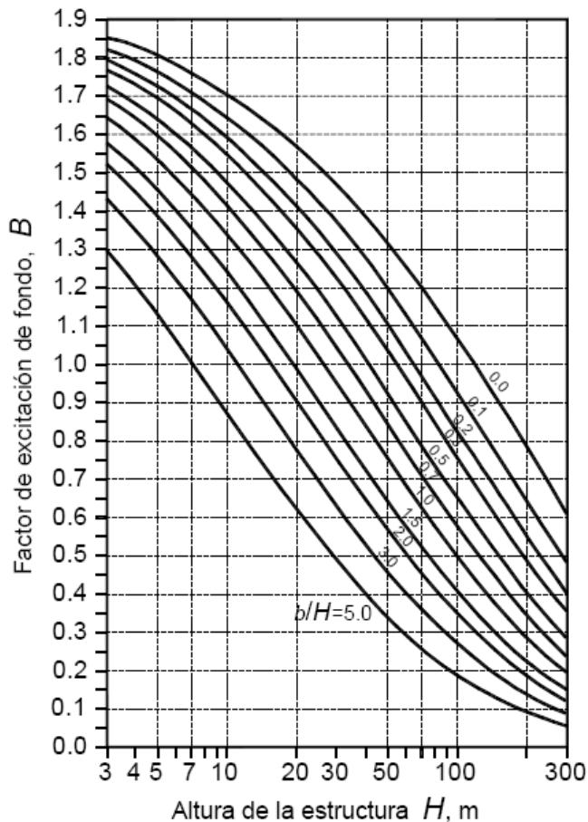
Figura 5.2. Factor de excitación de fondo (Referencia 1).
