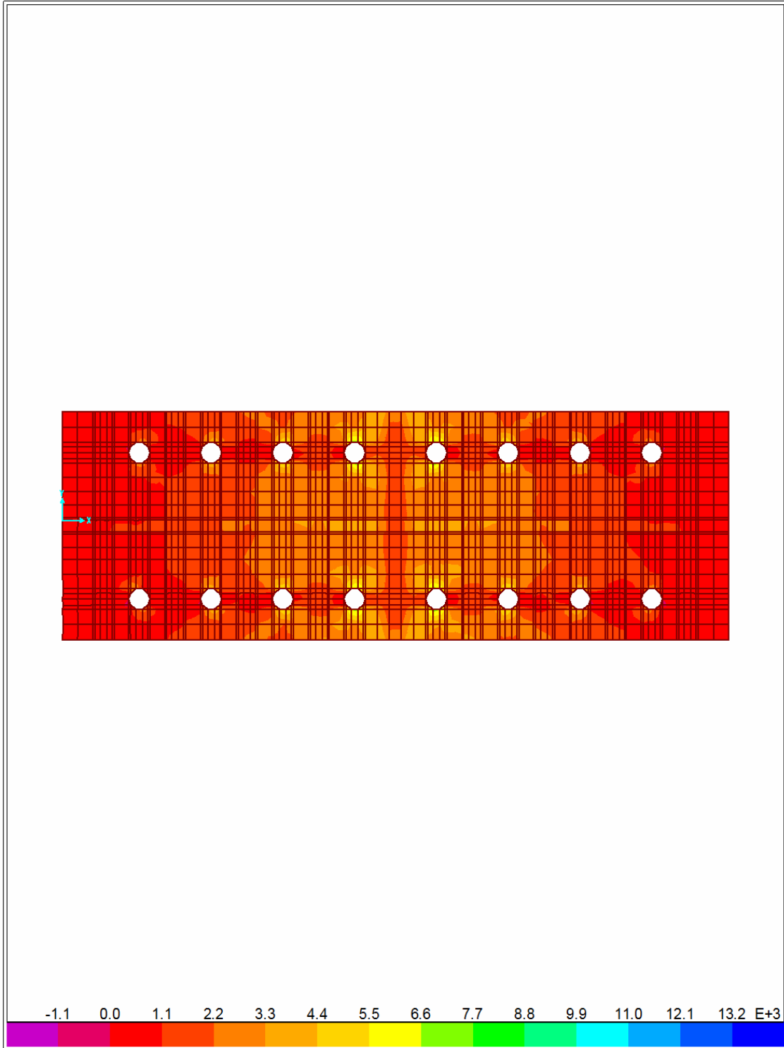
Figura A.4. Resultado del análisis: Esfuerzos máximos de tensión que se generan sobre las placas de conexión.
