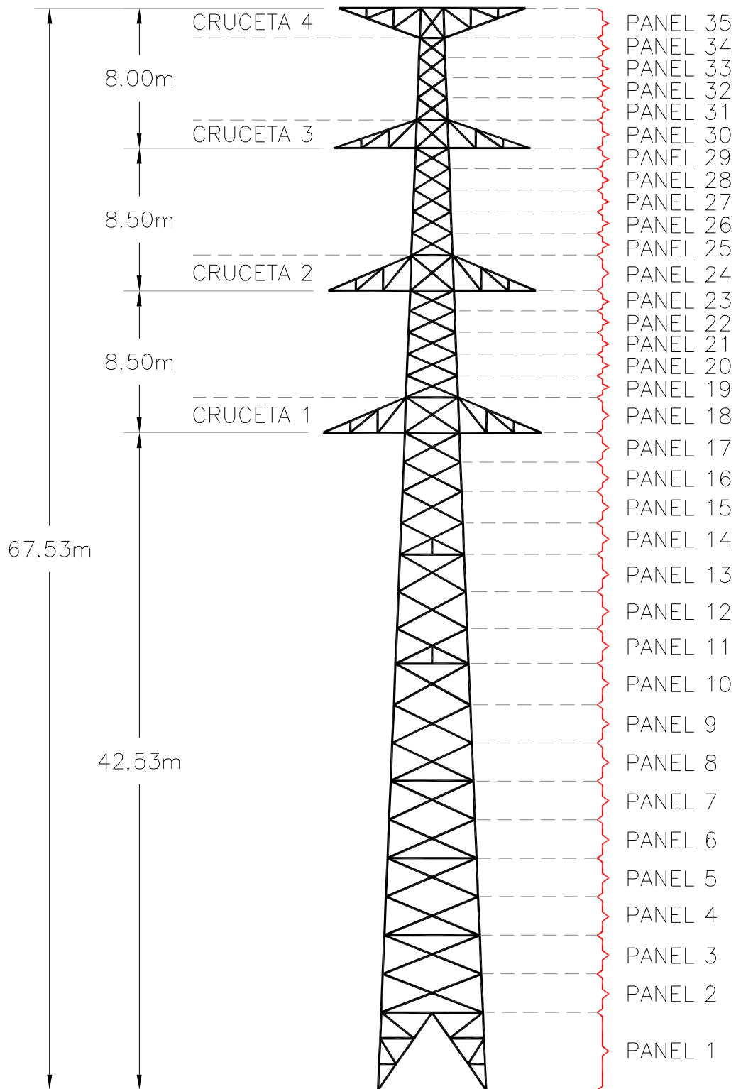
Figura 7.2. Paneles en que están divididas las torres de soporte.
