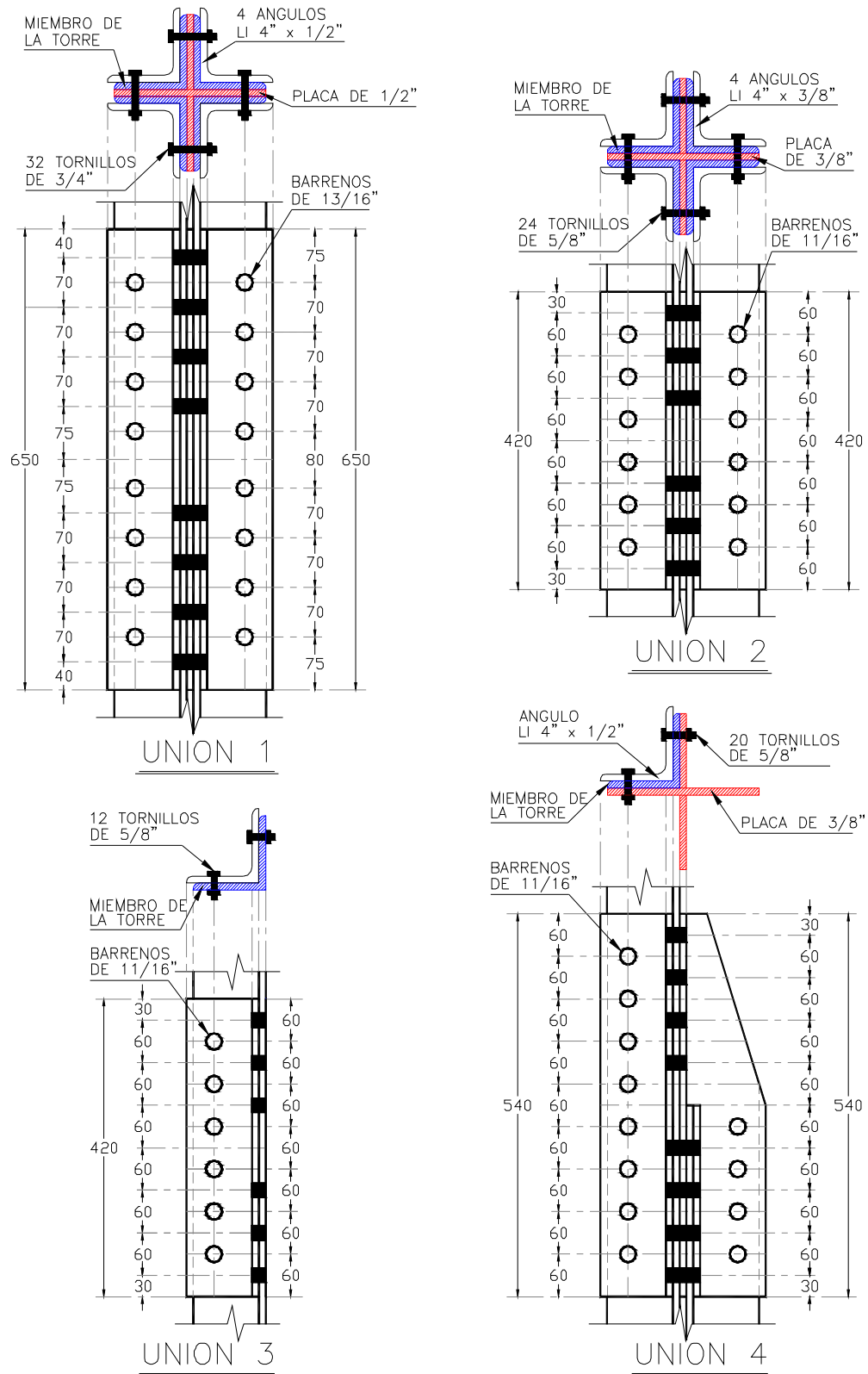
Figura 8.32. Conexiones tomadas del proyecto original (parte 1).
