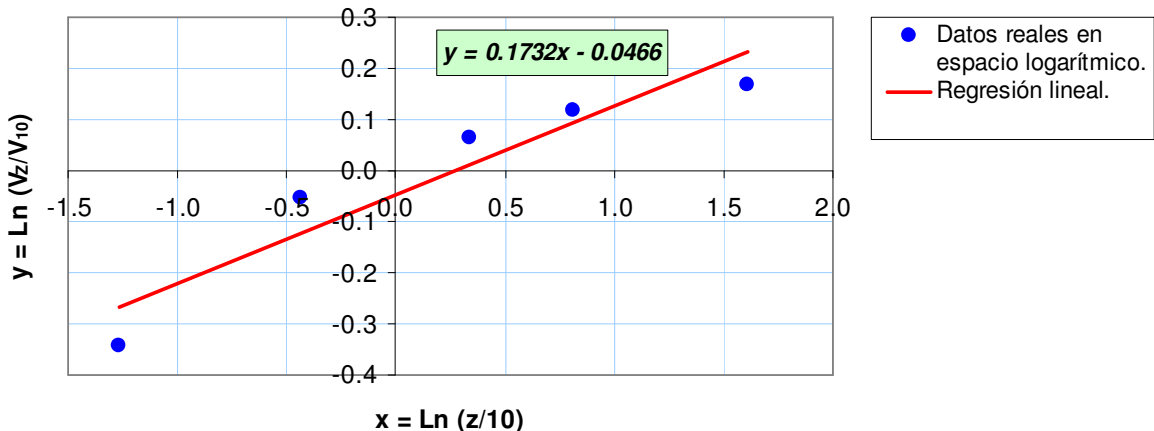
Figura 3.3. Parámetro “ \alpha ” para alturas 10\text{ m} \leq Z \leq 50\text{ m} .
