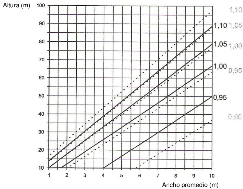
Figura 5.13. Factor estructural para torres con celosías, C_s C_d (Referencia 5).
