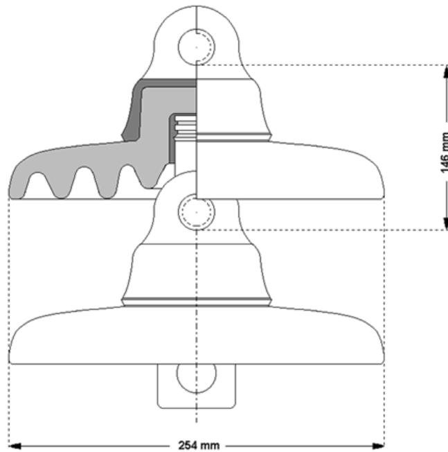
Figura 2.3. Aislador de suspensión, cementado, tipo de charnela (Referencia 6).
