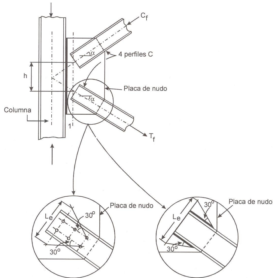
Figura 6.6. Ancho efectivo, L_e ; hipótesis de Whitmore (Referencia 4).
