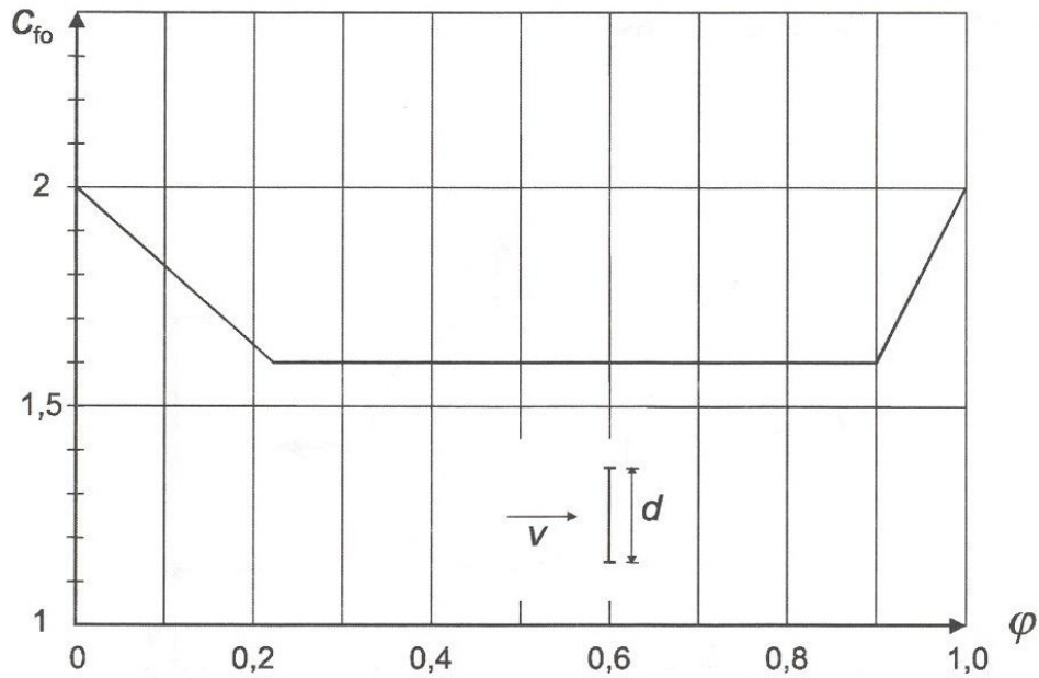
Figura 5.14. Coeficiente de fuerza C_{f,0} para una estructura con celosías plana con miembros angulares, en función del factor de solidez \varphi (Referencia 5).
