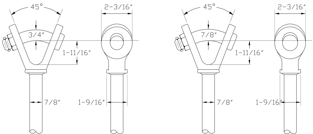
Figura A.7. Secciones de los ganchos "Y" analizados (Referencia 23).
