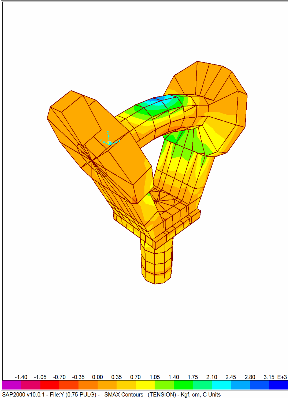
Figura A.8. Resultados del análisis del gancho “Y” de 3/4” de diámetro (Esfuerzos Máximos).
