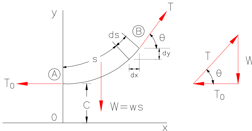
Figura 7.4. Tensiones que define una curva catenaria (Referencia 12).
