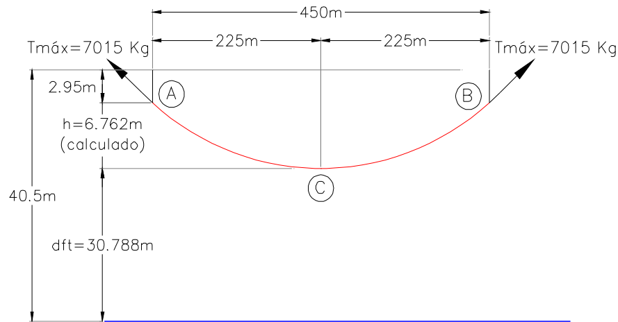
Figura 7.5. Configuración de los cables conductores más próximos al nivel del terreno.
