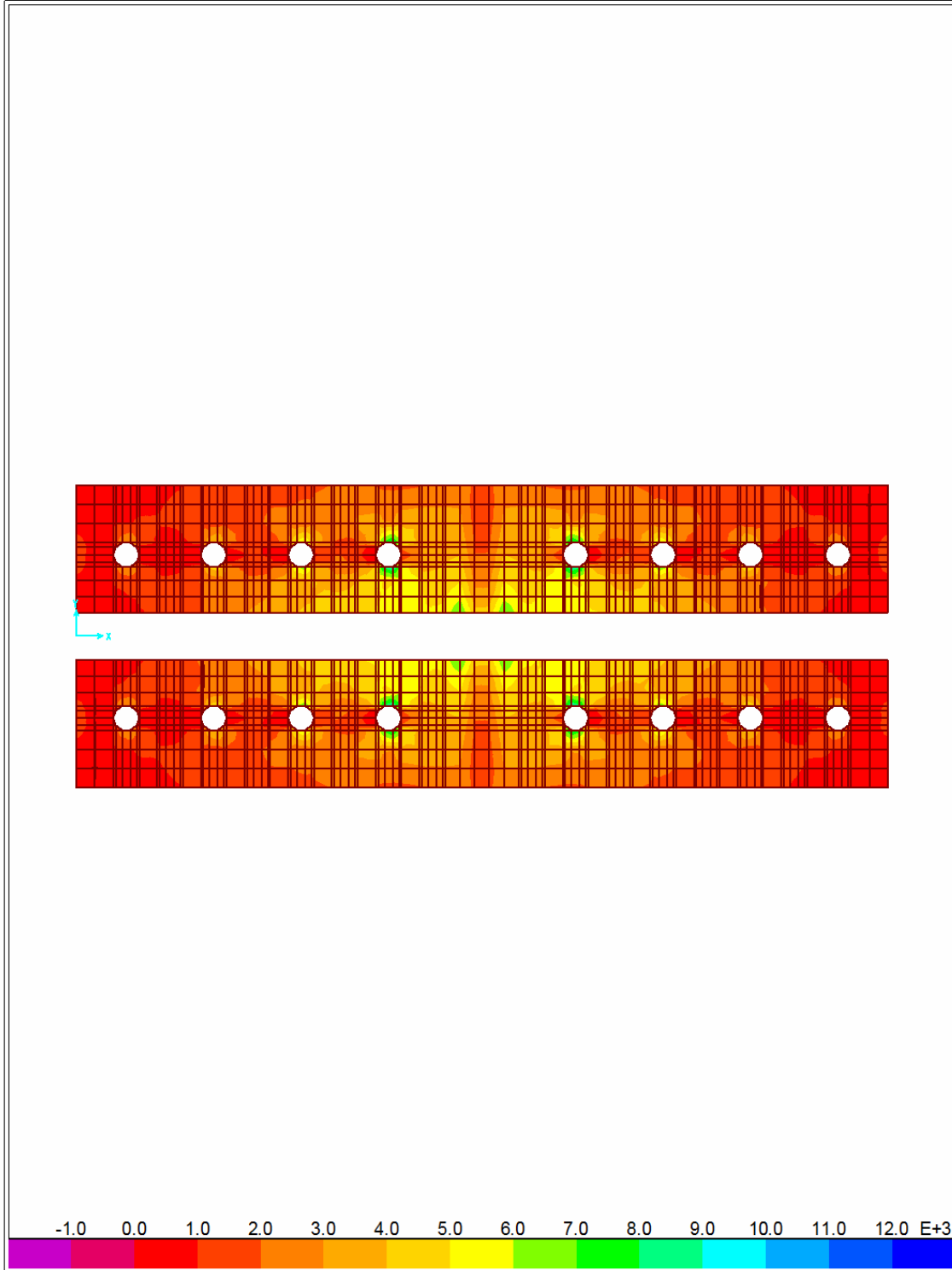
Figura A.5. Resultado del análisis: Esfuerzos máximos de tensión que se generan sobre los ángulos de conexión.
