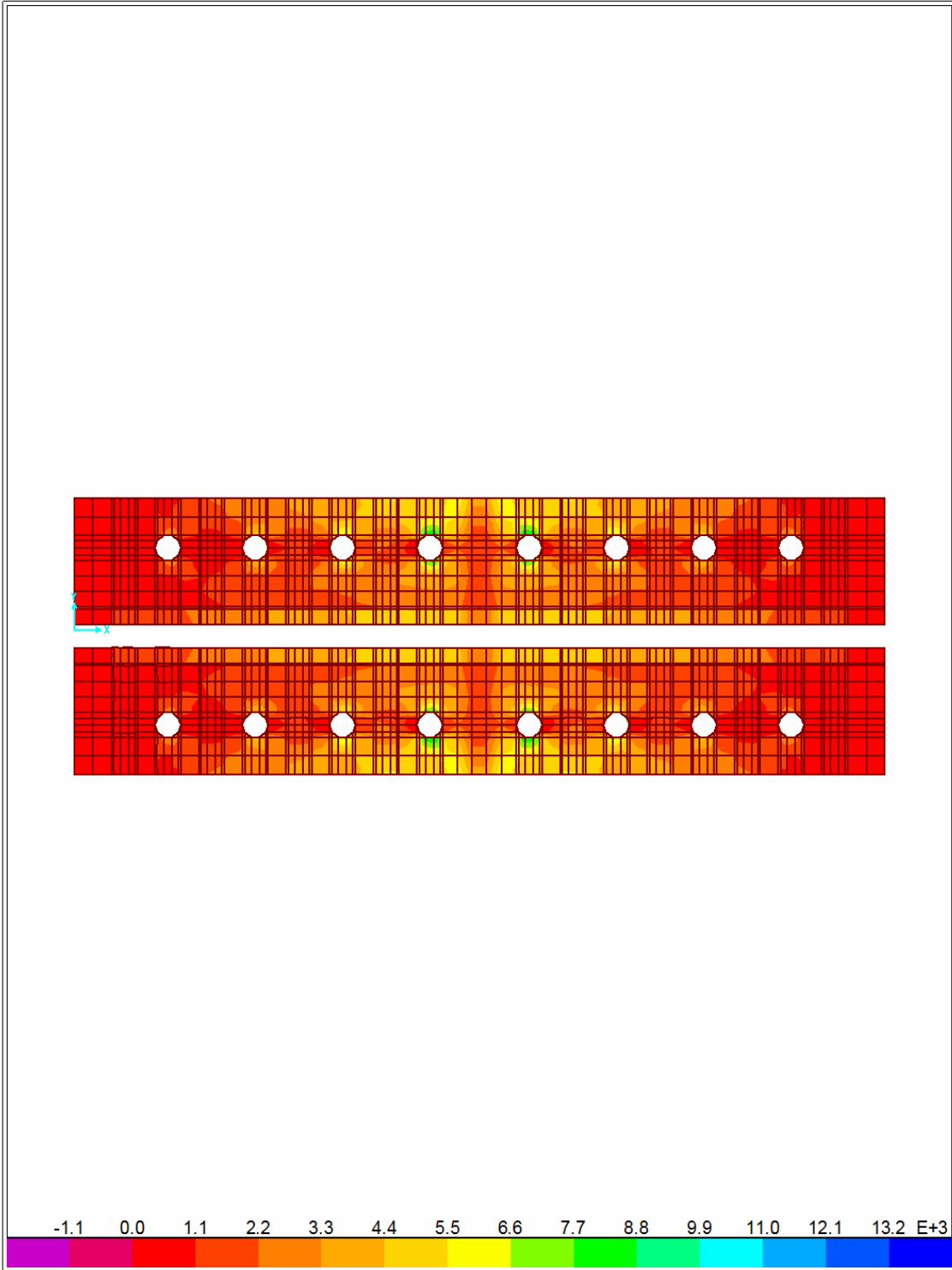
Figura A.6. Resultado del análisis: Esfuerzos máximos de tensión que se generan sobre los miembros de las torres.
