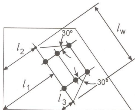
Figura 6.5. Dimensiones para determinar la resistencia a pandeo de una placa de nudo (Referencia 4).
