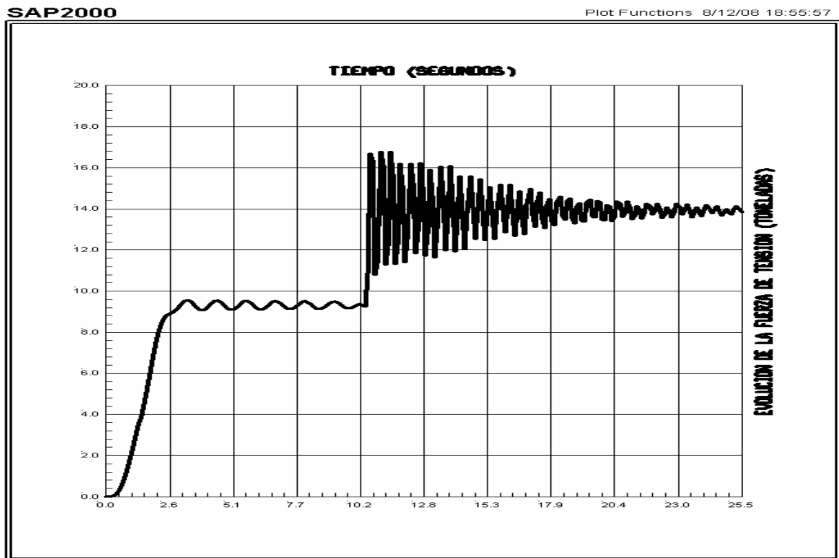
Figura 8.2. Historia de cargas de un miembro diagonal del panel 1.
