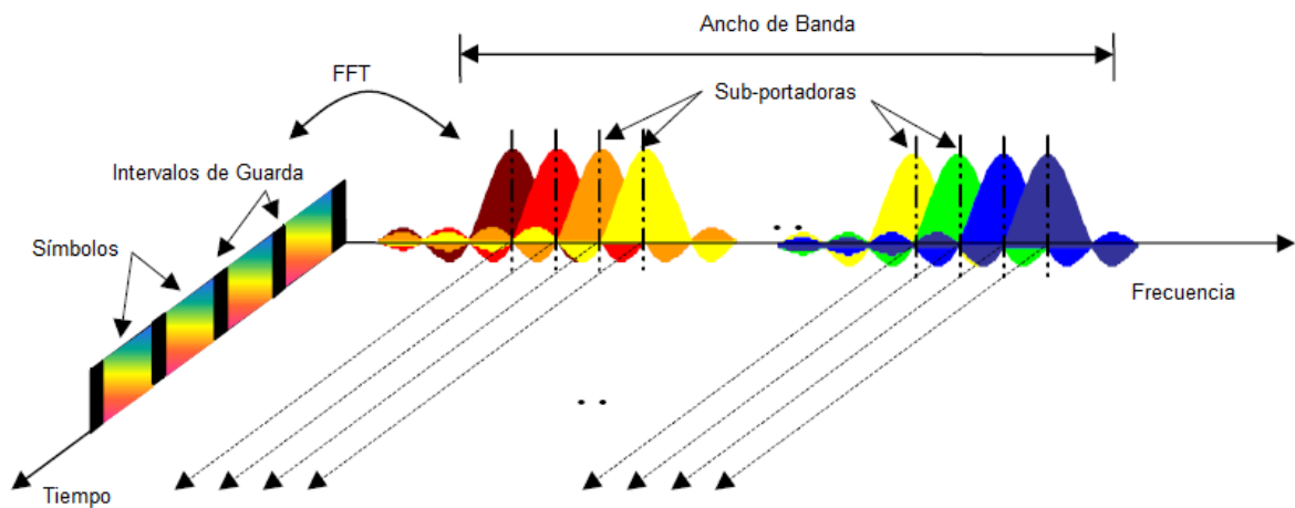
Figura 4.12 Representación del esquema OFDM
