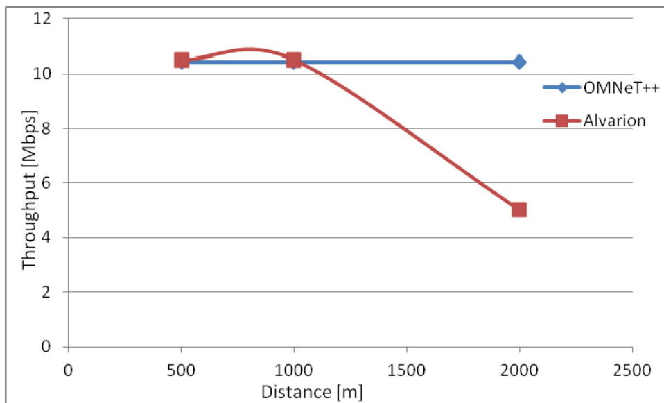
Figura 5.23 Comparación del throughput para QAM64
