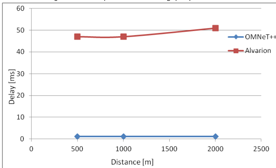
Figura 5.24 Comparación del delay para QAM64
