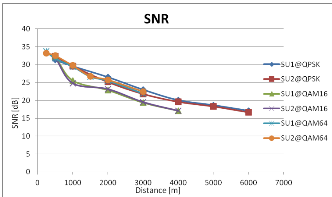
Figura 5.11 SNR en las diferentes modulaciones para los dos suscriptores
