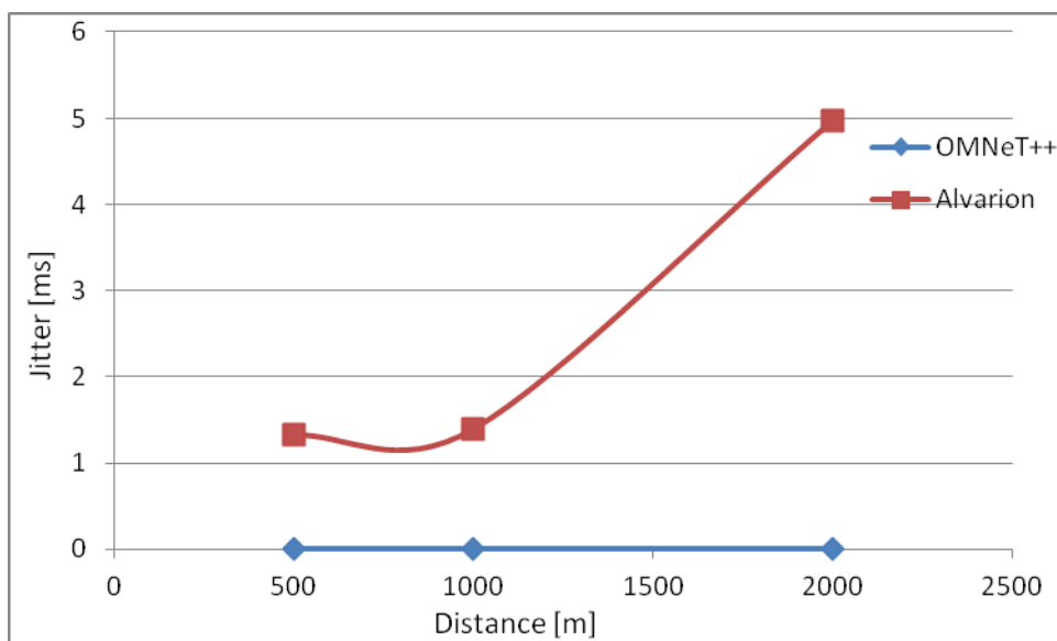
Figura 5.25 Comparación del jitter para QAM64
