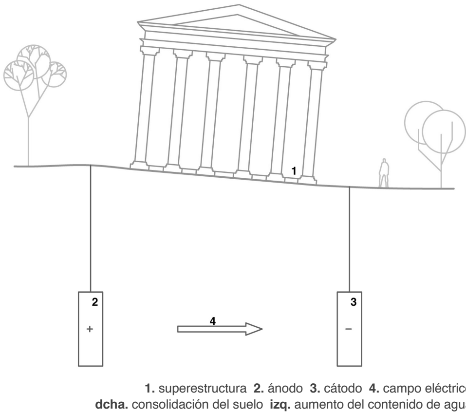
Figura 3.14. Principio de la electro-osmosis.
