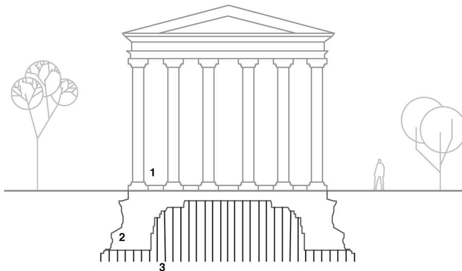
1. superestructura 2. cimentación preservada 3. cimentación desmantelada
