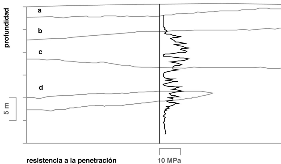
Figura 4.23. Perfil de suelo con base en los resultados de sondeos y pruebas de piezocono.
