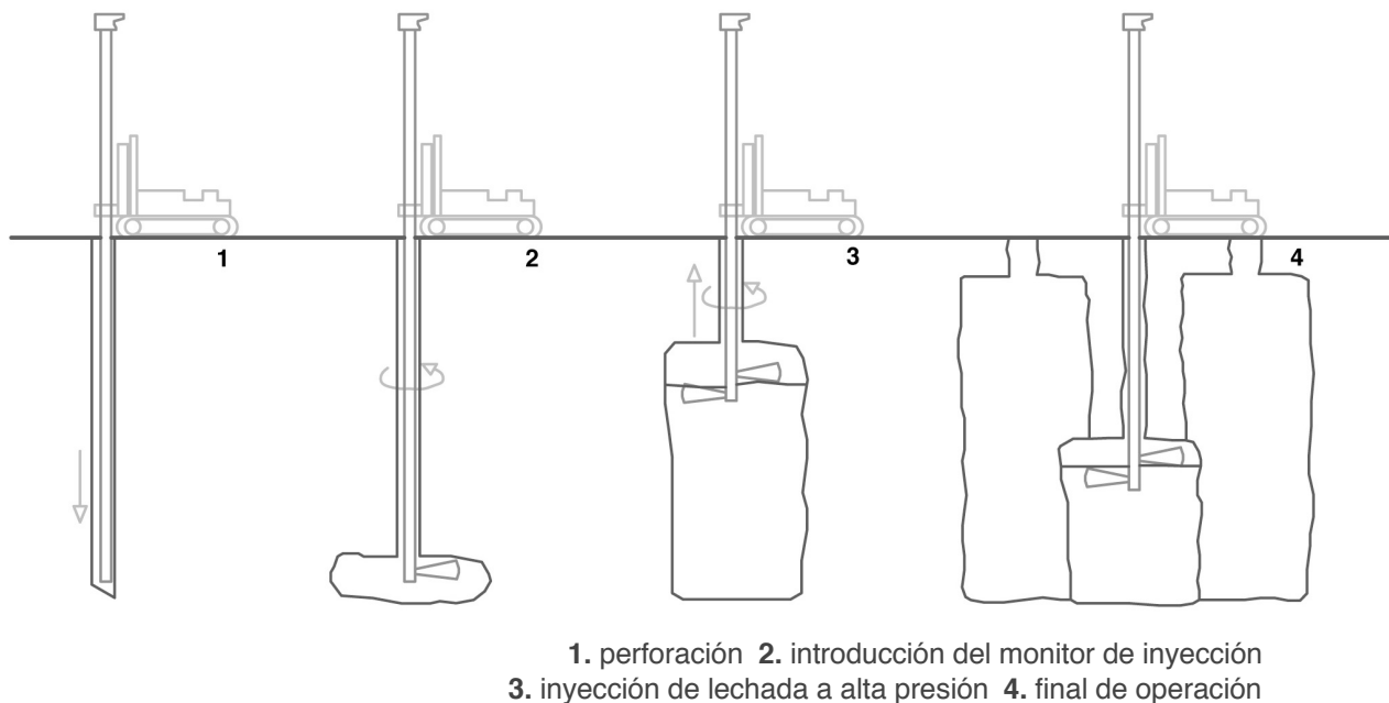
Figura 3.17. Procedimiento constructivo del Get-Grout y Deep-Mixing.
