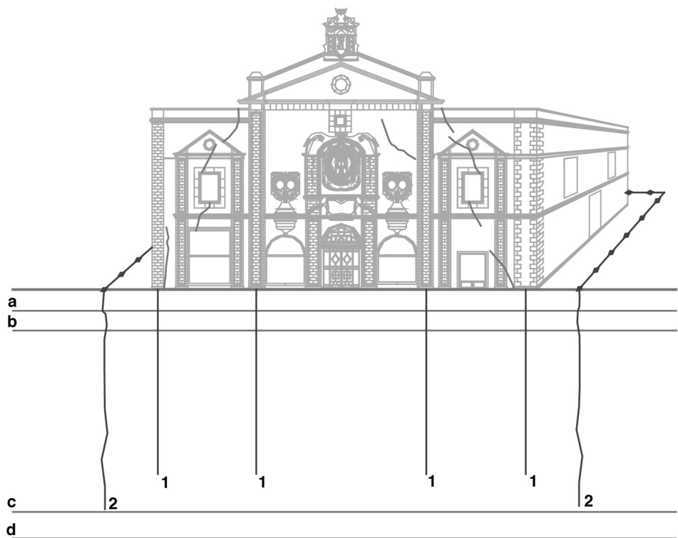
1. micropilote 2. fisura inducida a, b, c, d. estratos como descritos en la tabla 4.1
