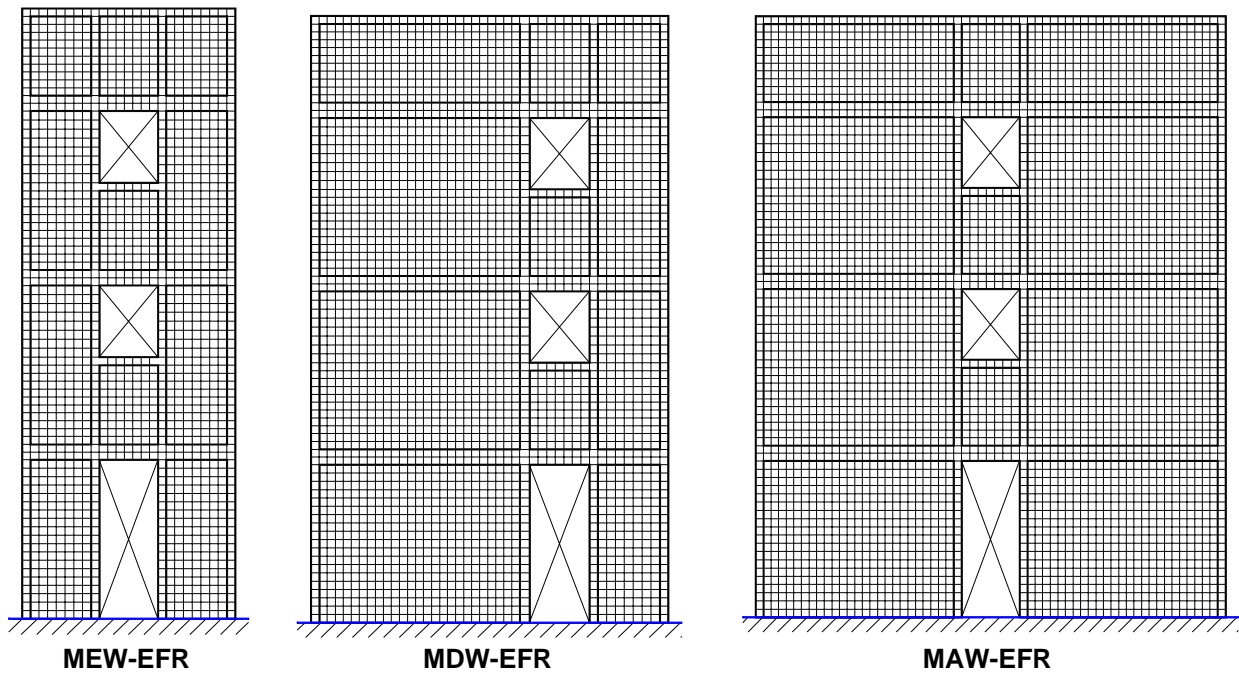
Fig. 4.32 Modelos de referencia serie WWW: muros acoplados por pretil
