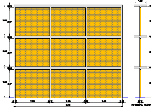
Fig. 4.17 Dimensiones modelo marco M3
