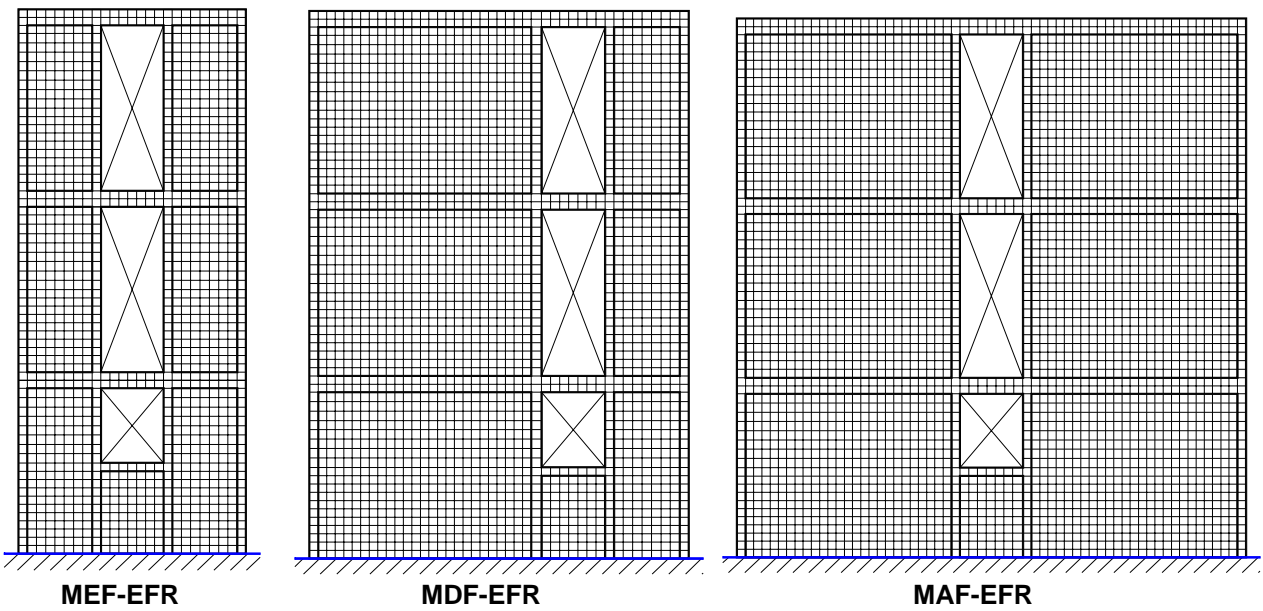
Fig. 4.33 Modelos de referencia serie WFW: muros con pretil inferior
