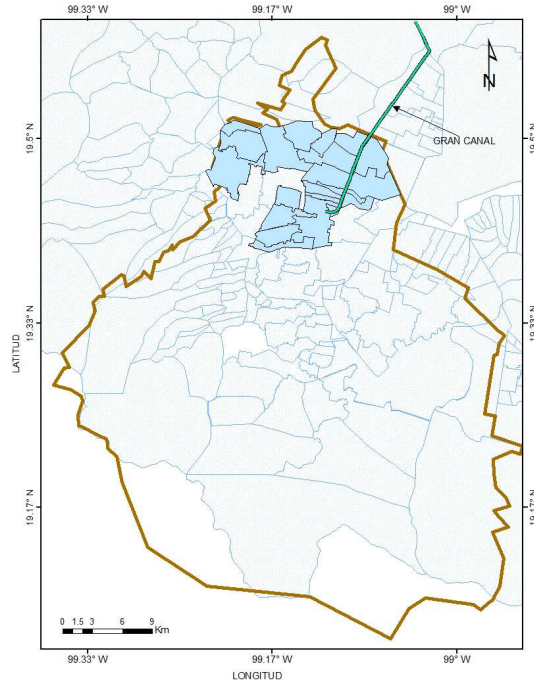
Figura 4.23. Escenario de inundación 4
