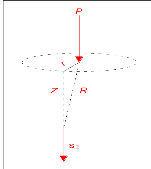
Figura 28, Distribución de Presiones de una Carga Concentrada
