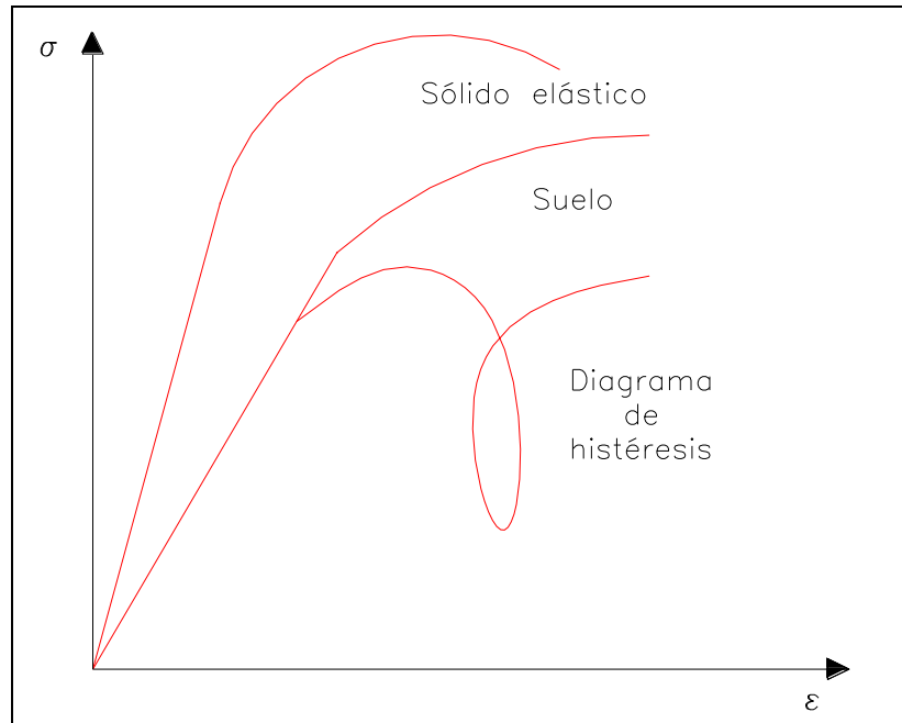
Figura 48, Diagrama de Esfuerzos de Distintos Materiales
