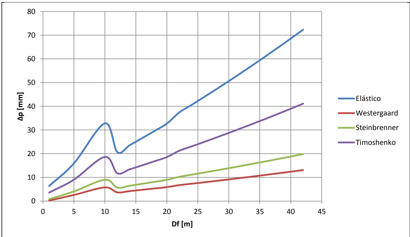
Figura 70, Comparación Asentamientos Timoshenko (D=1.00 m)
