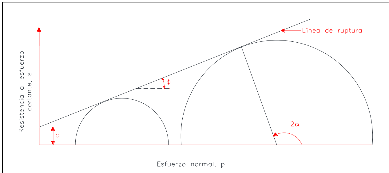
Figura 259, Diagrama de Ruptura de Mohr
