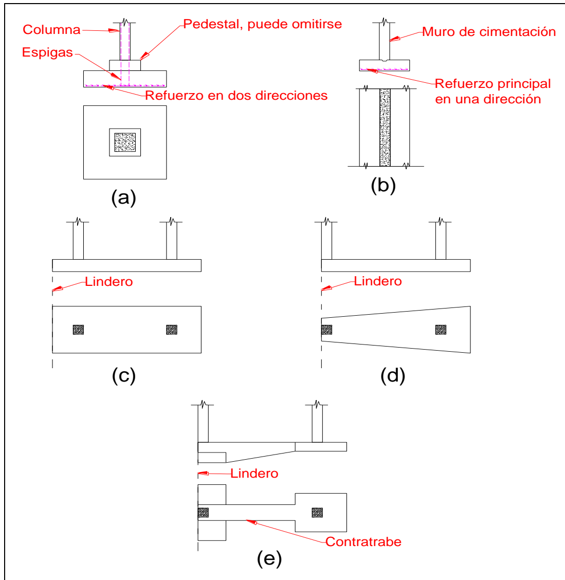
Figura 26, Tipos de Zapatas, a) Zapata Individual para Columna, b) Zapata para Muro, c) y d) Zapatas Combinadas, e) Zapata en Cantiliver
