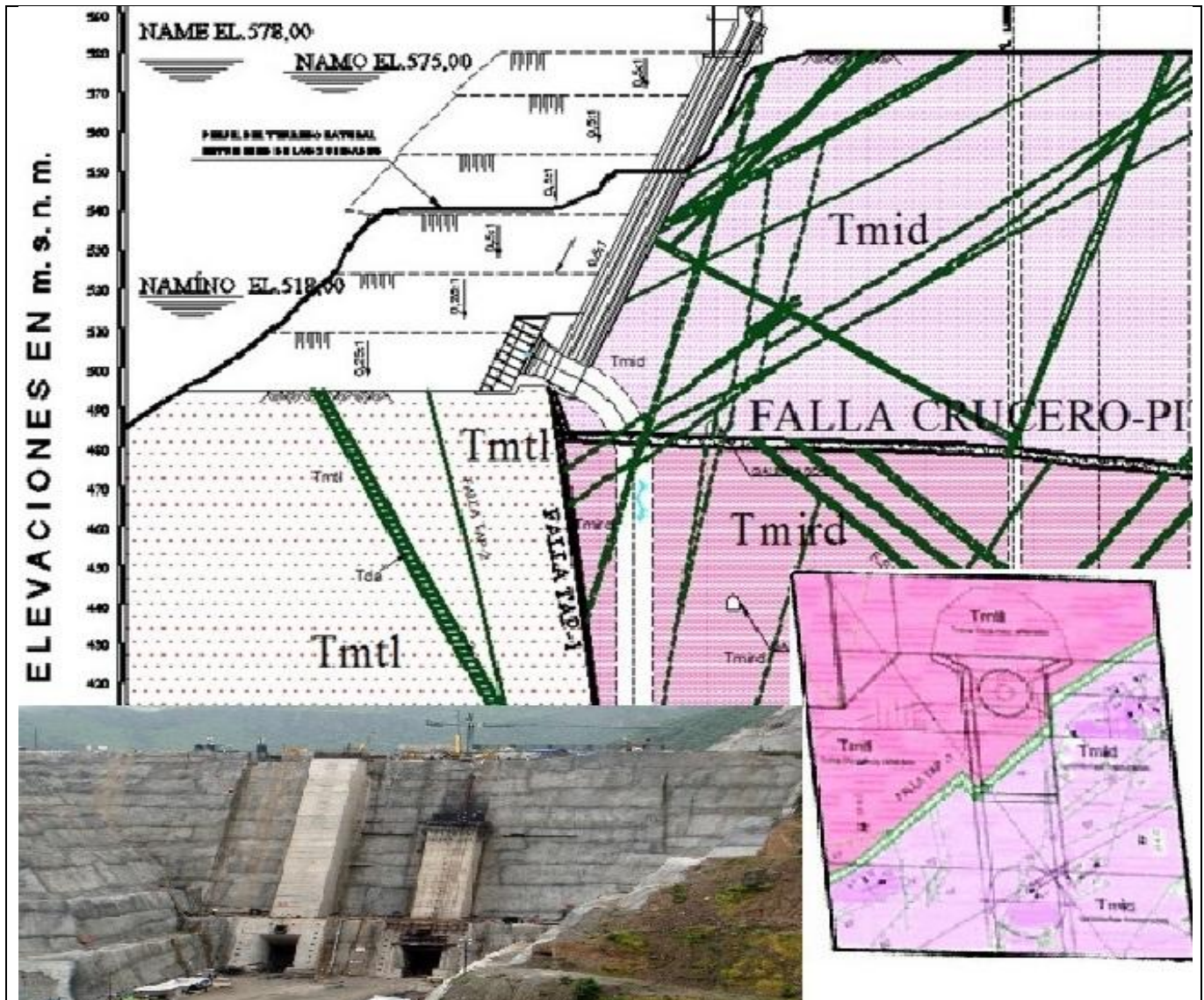
Figura 57, Geología de la Obra de Toma
