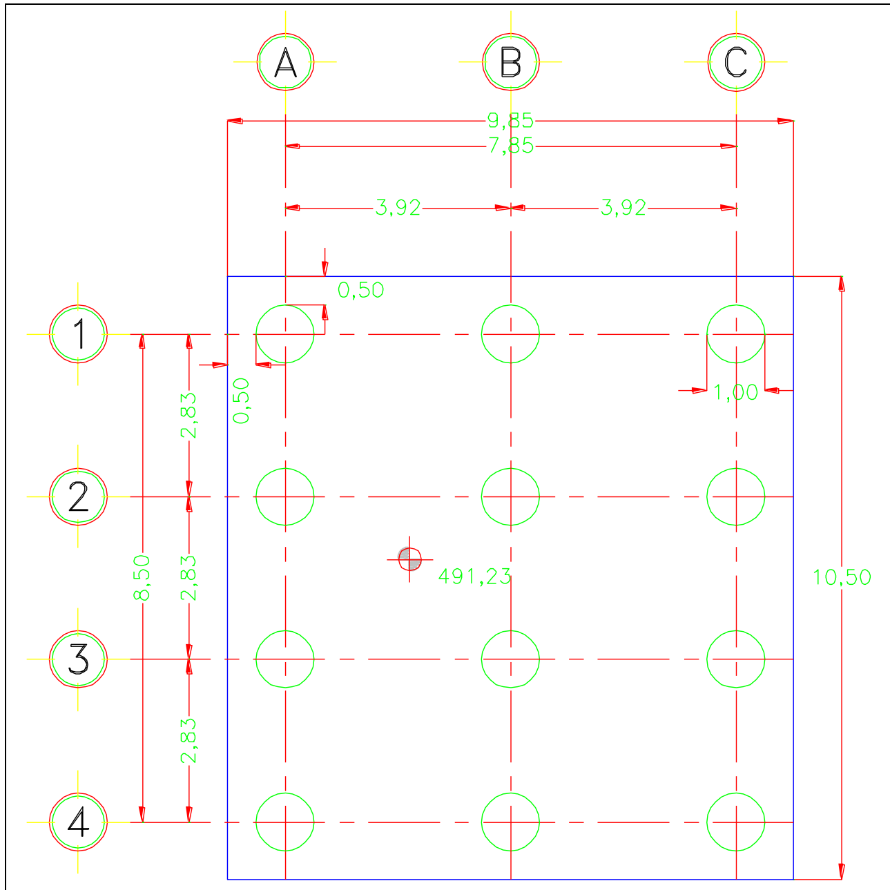
Fuente: Elaboración propia. Figura 74, Planta de Cimentación
