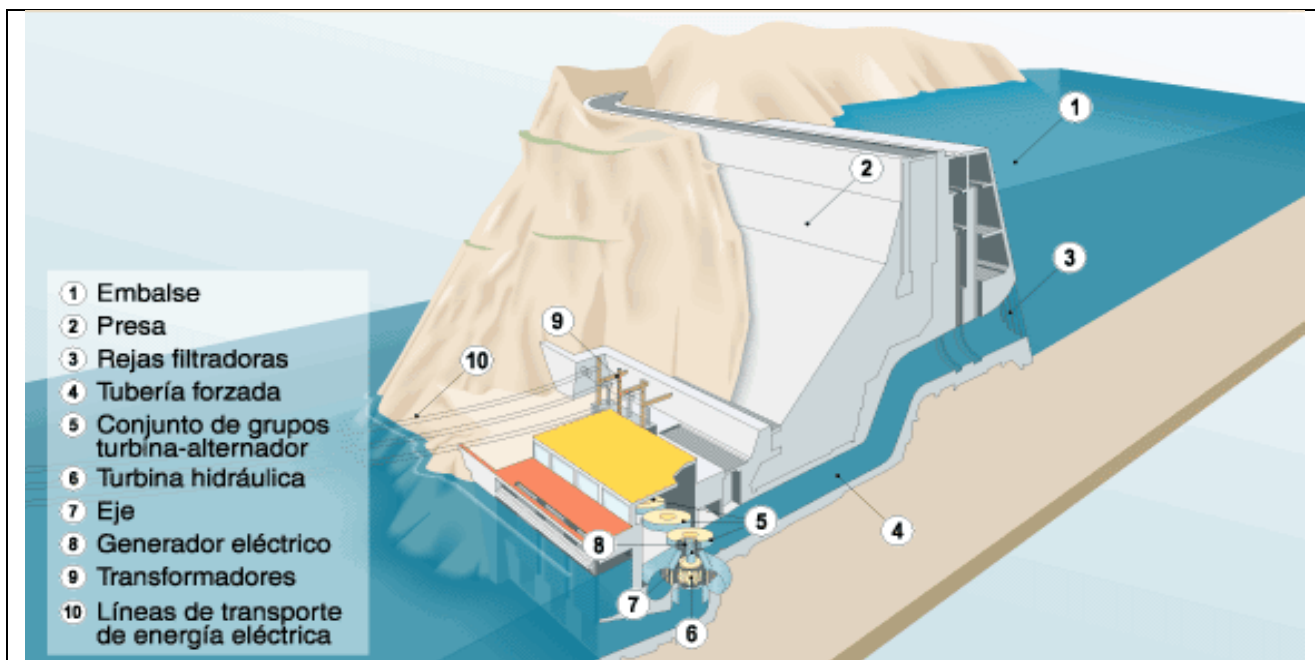
Figura 12, Partes de una Central Hidroeléctrica
