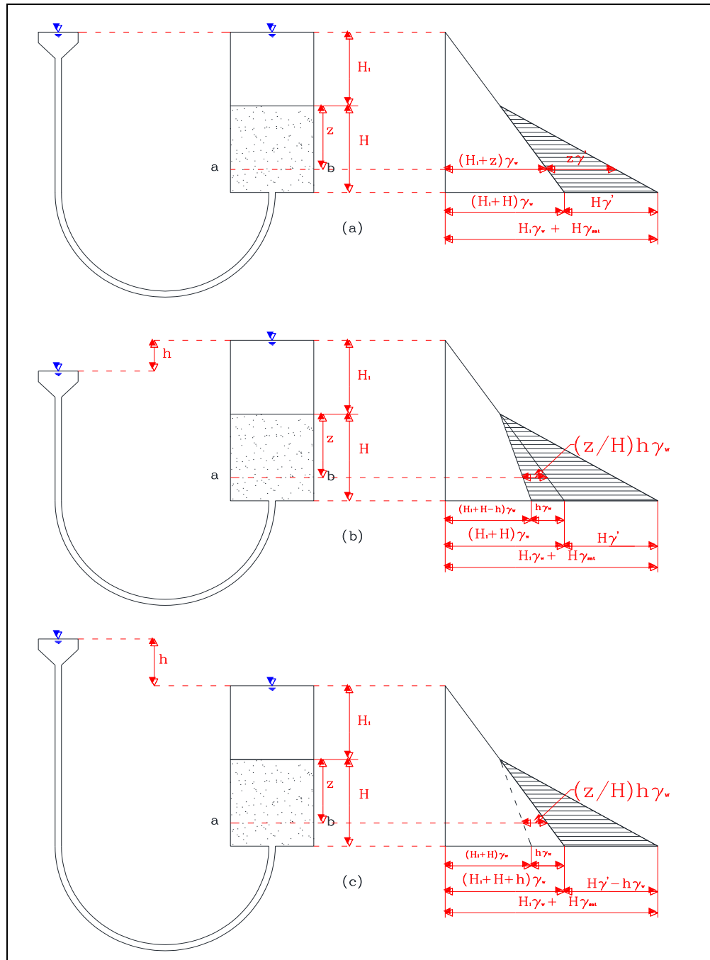
Figura 22, Diagrama de Presión Rfectiva y Presion de Poro
