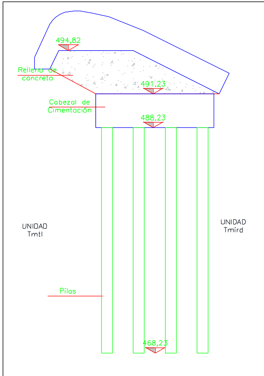
Figura 79 Cimentación Obra de Toma U2.
