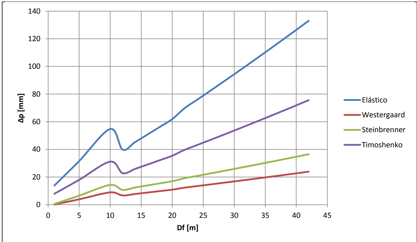
Figura 73, Comparación Asentamientos Timoshenko (D=1.90 m)
