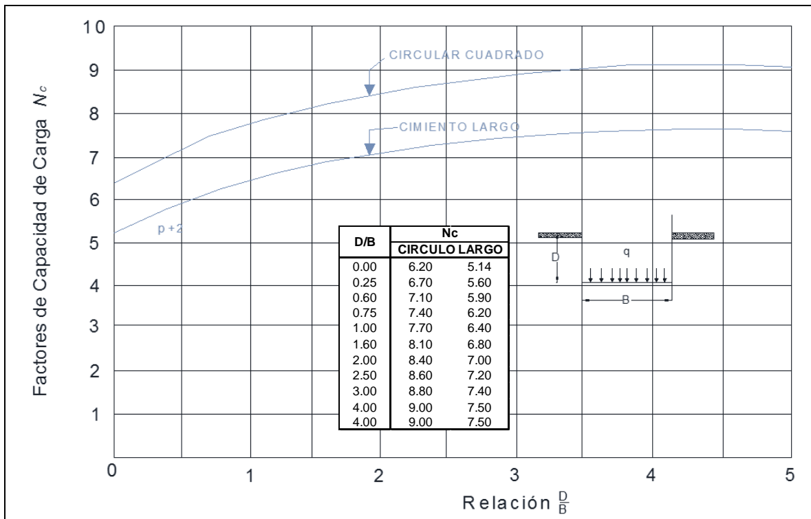
Figura 36, Valores de N_c según Skempton, para Suelos Cohesivos
