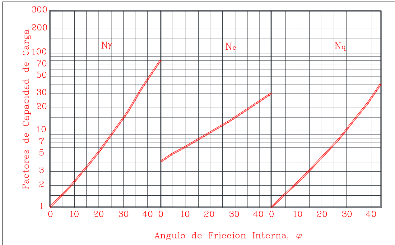
Figura 37, Factores de Capacidad de Carga, según Bell
