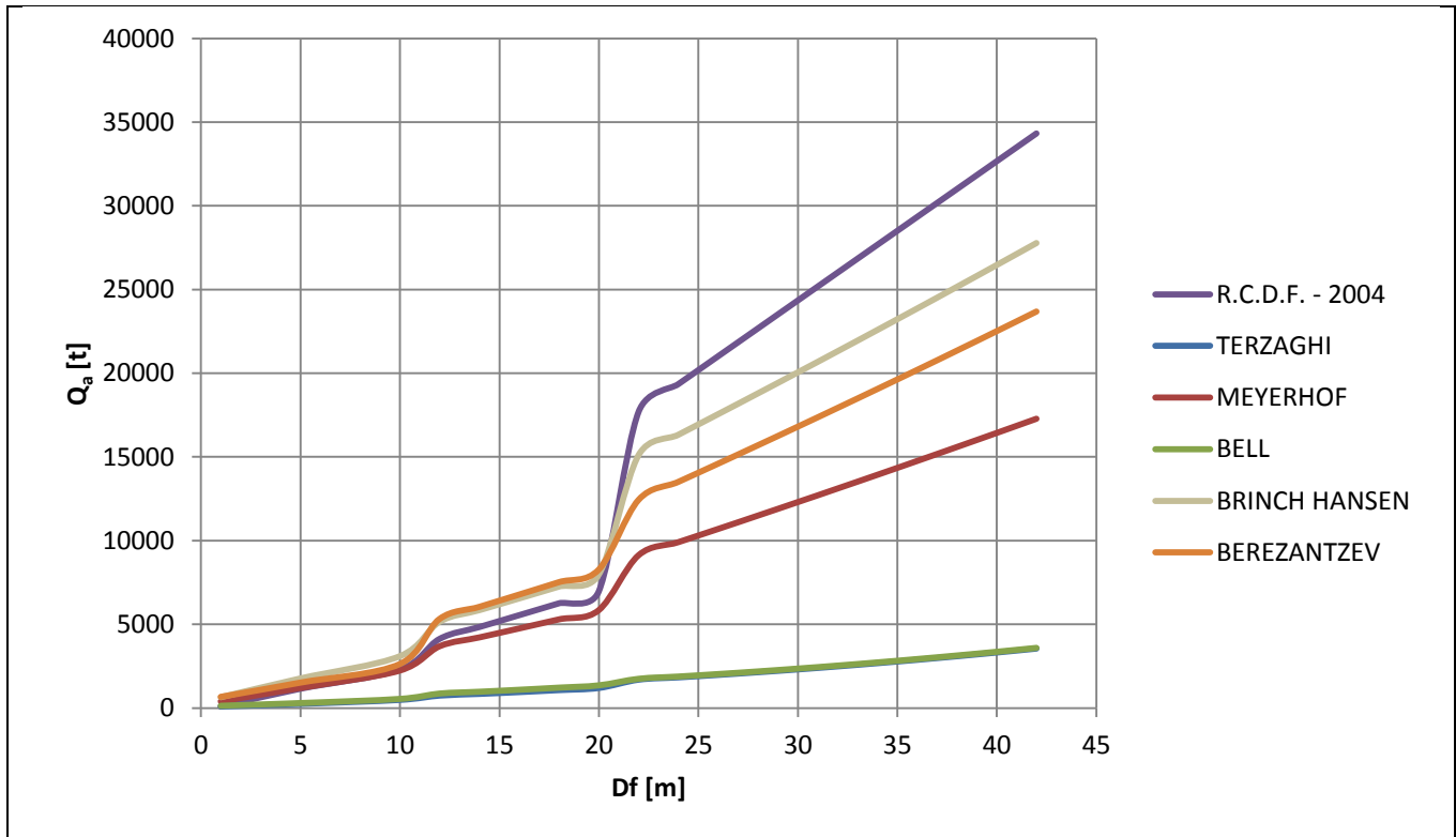
Figura 65, Comparación Teorías Capacidad de Carga (D=1.90 m)
