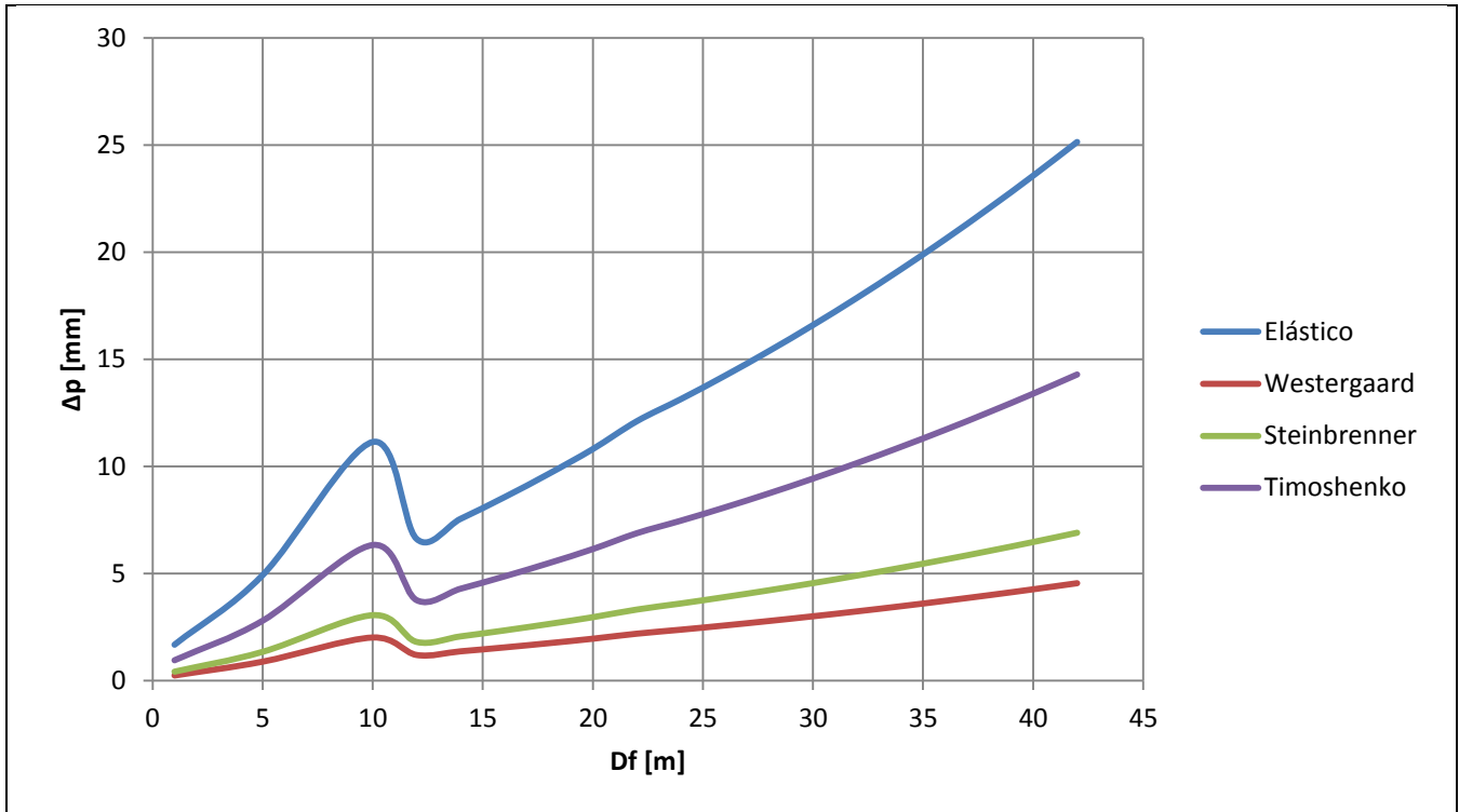
Figura 66, Comparación Asentamientos Timoshenko (D=0.30 m)
