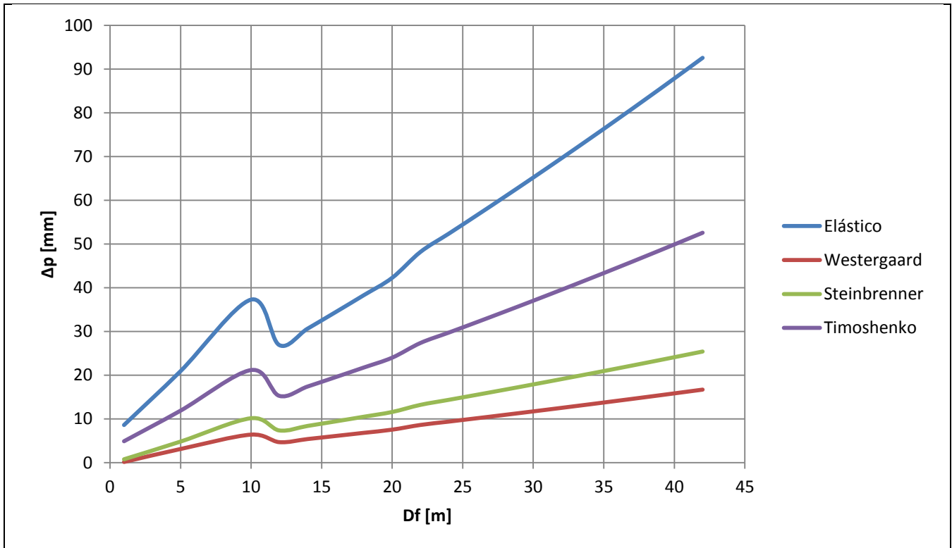
Figura 71, Comparación Asentamientos Timoshenko (D=1.30 m)
