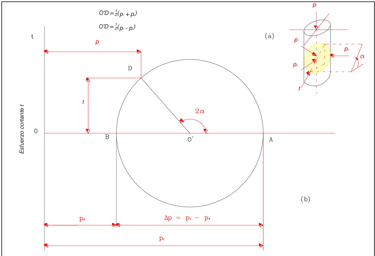
Figura 24, a) Esfuerzos en Espécimen Probado en la Cámara Triaxial e Inclinación \alpha del Plano de Falla con la Horizontal, b) Círculo de Esfuerzos de Mohr
