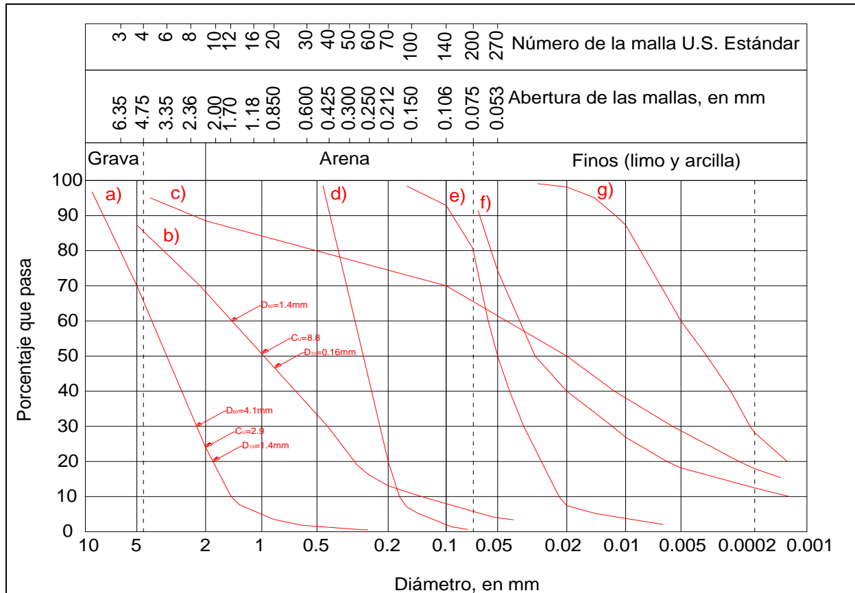
Fuente: Crespo, 2008. Figura 17, Curvas Típicas de Distribución Granulométrica de Algunos Suelos Naturales.
