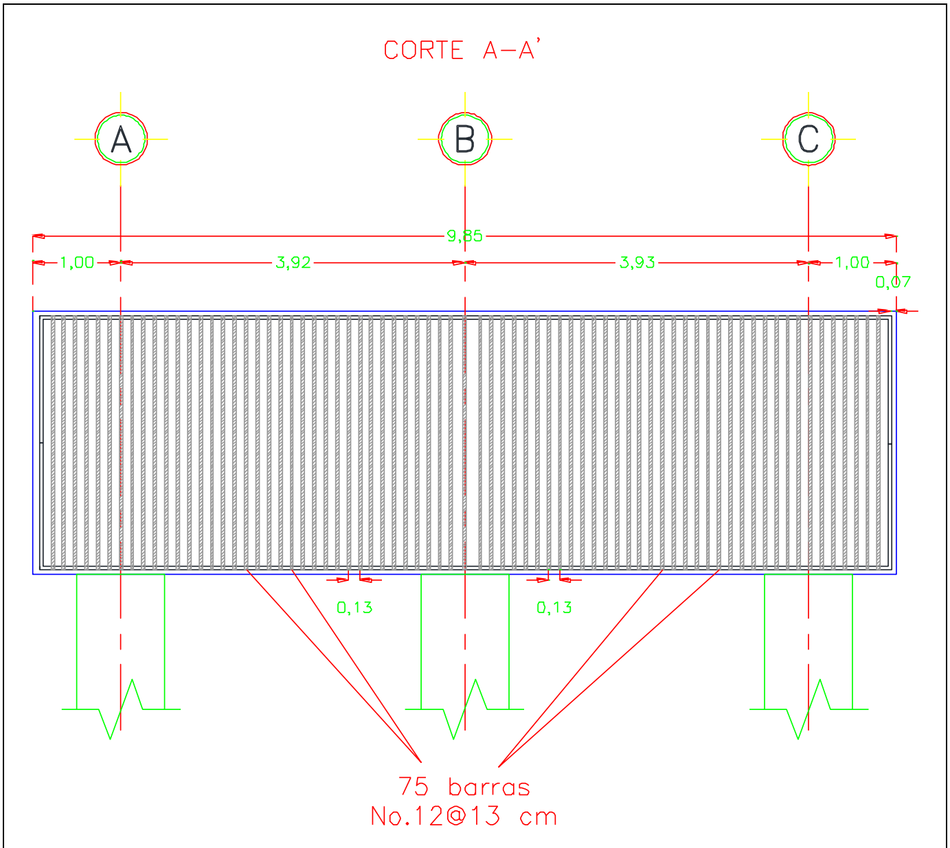
Figura 77, Acero de Refuerzo en Cabezal
