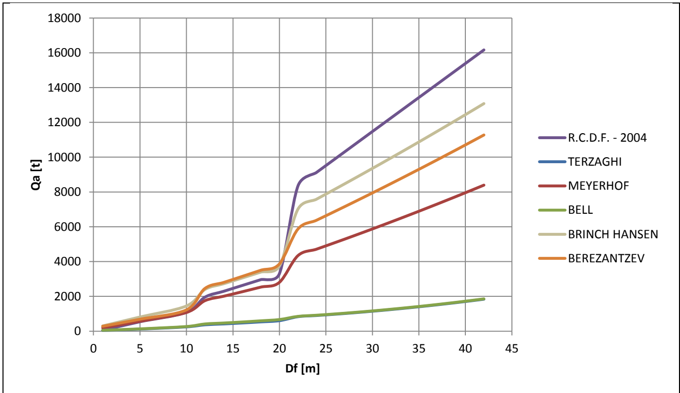
Figura 63, Comparación Teorías Capacidad de Carga (D=1.50 m)
