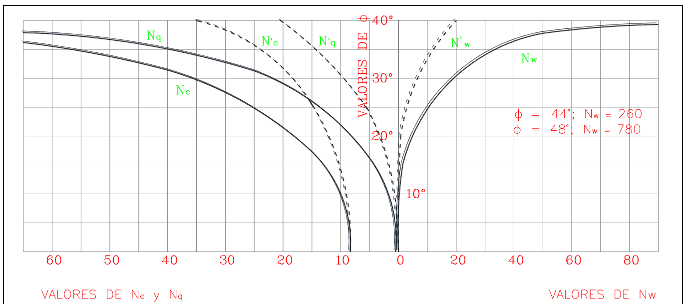
Figura 32, Factores de Capacidad de Carga según Terzaghi
