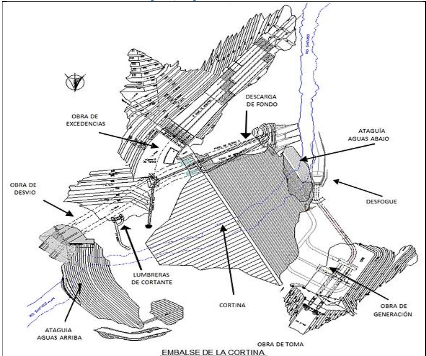
Figura 16, Arreglo General del P.H. La Yesca
