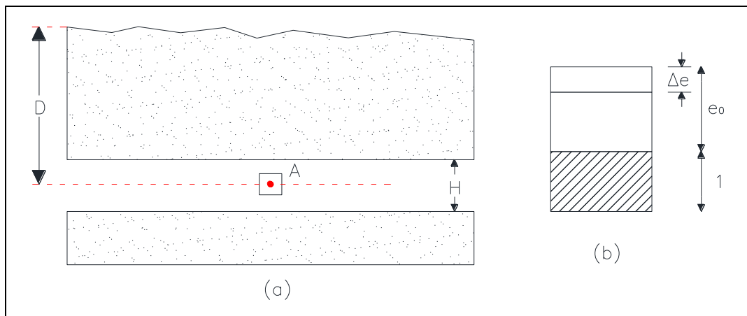
Figura 23, a) Sección a Través de un Manto de Arcilla Compresible, b) Compresión de un Elemento del Manto
