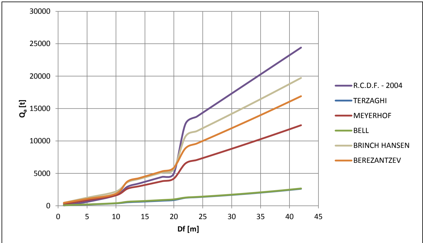
Figura 64, Comparación Teorías Capacidad de Carga (D=1.60 m)
