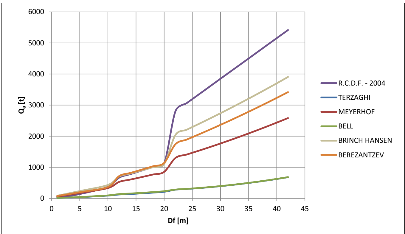
Figura 60, Comparación Teorías Capacidad de Carga (D=0.70 m)
