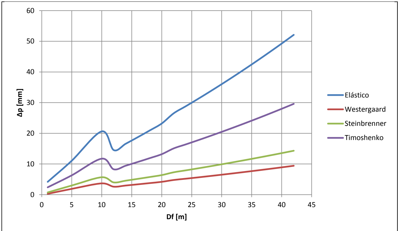
Figura 68, Comparación Asentamientos Timoshenko (D=0.70 m)
