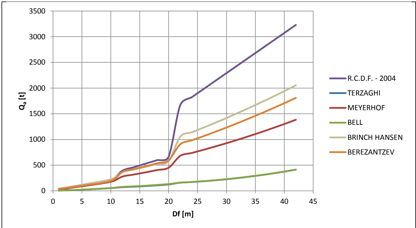
Figura 59, Comparación Teorías Capacidad de Carga (D=0.50 m)
