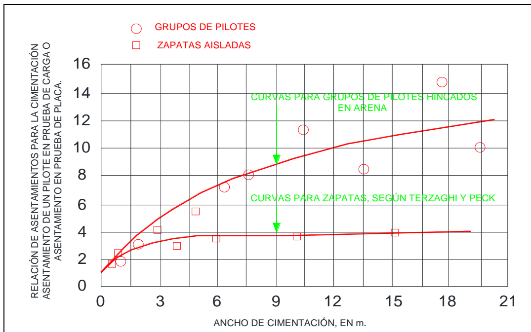
Figura 43, Curva Empírica para Calcular Asentamientos de Grupos de Pilotes en Arenas
