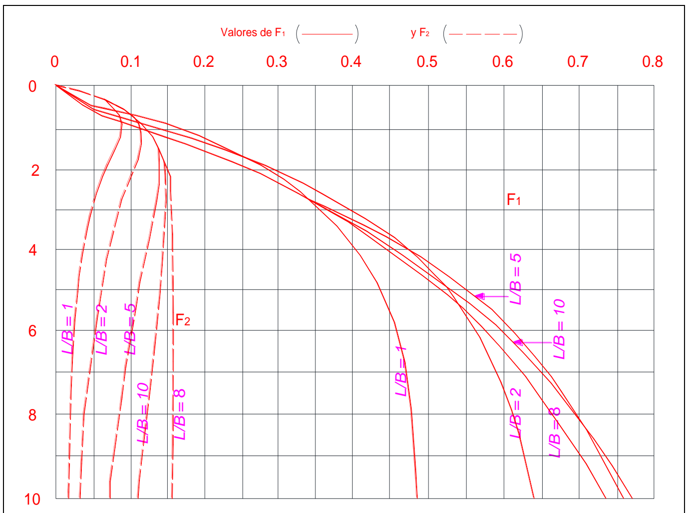
Figura 52, Factores de Influencia F_1 y F_2 de Steinbrenner
