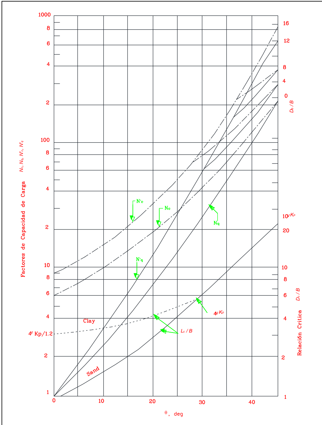
Figura 35, Factores de Capacidad de Carga según Meyerhof
