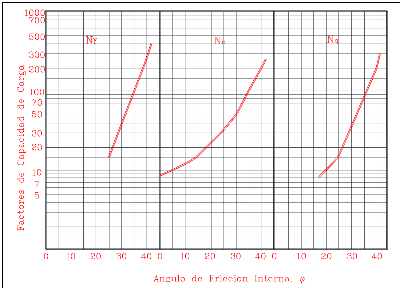
Figura 38, Factores de Capacidad de Carga, según Berezantzev
