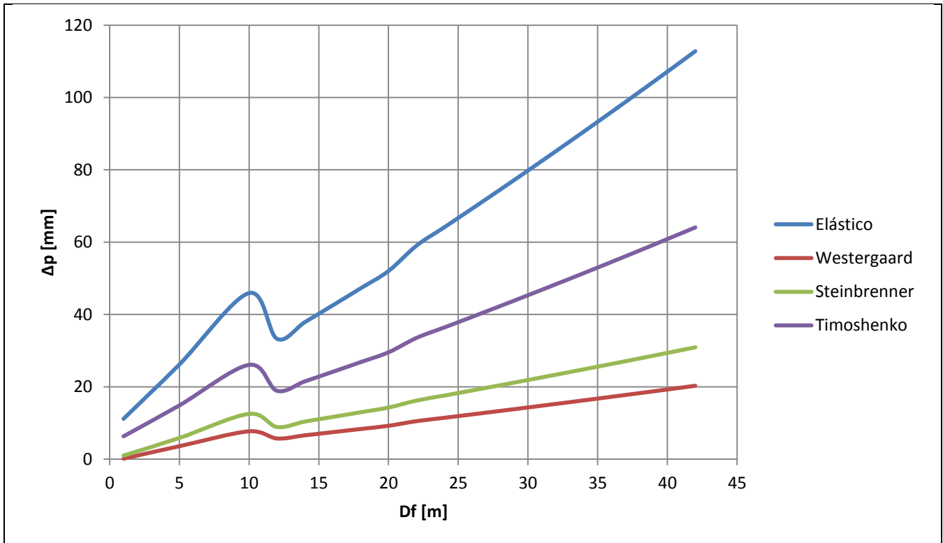
Figura 72, Comparación Asentamientos Timoshenko (D=1.60 m)
