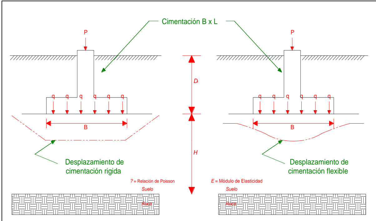
Figura 51, Asentamientos Elásticos y la Flexibilidad de la Cimentación
