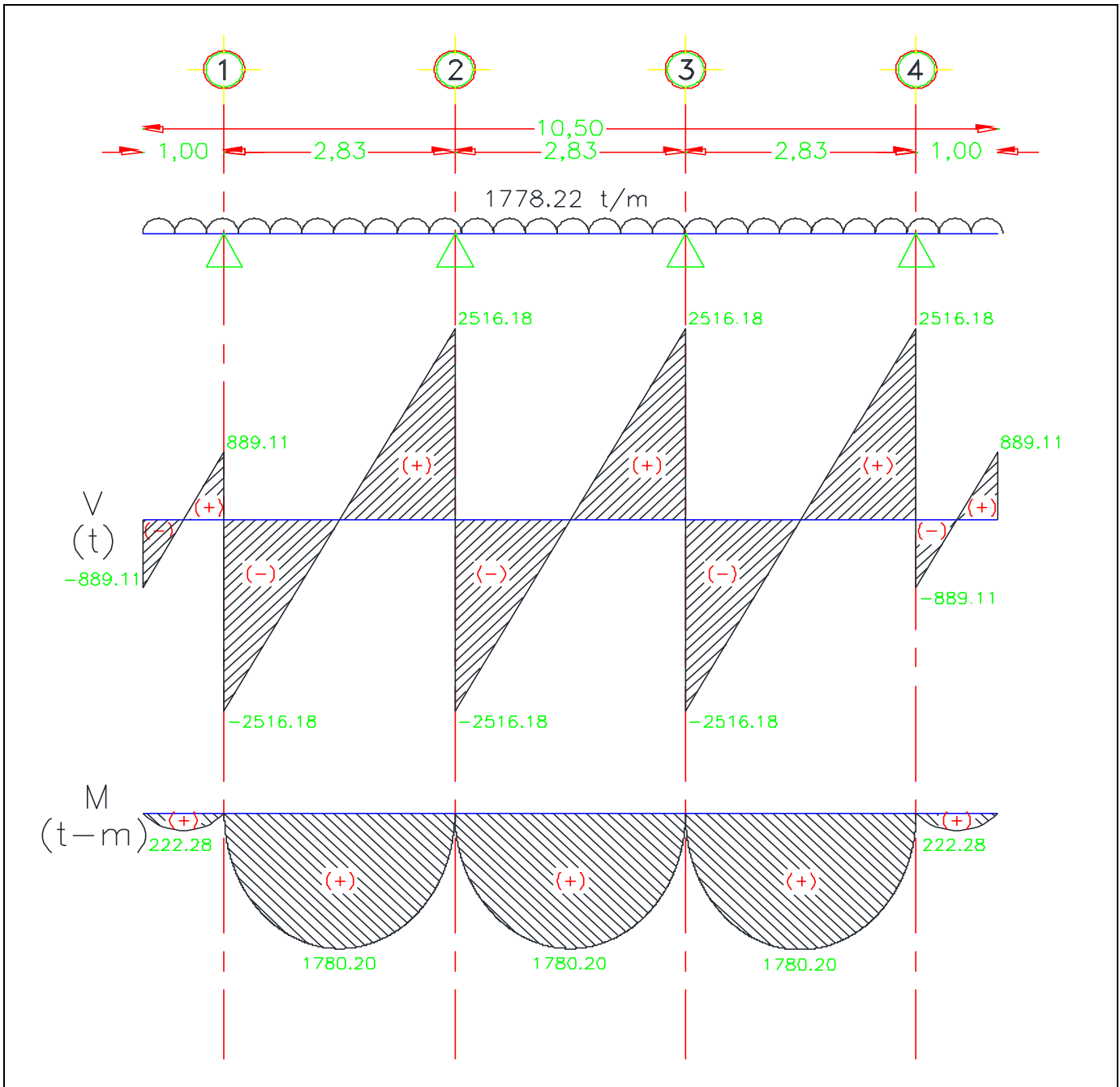
Figura 76, Diagrama de Elementos Mecánicos
