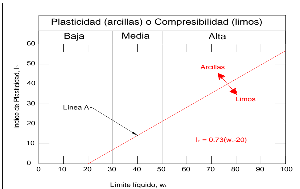
Figura 19, Carta de Plasticidad (A. Casagrande, 1948)
