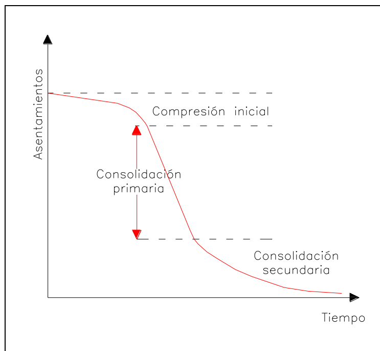
Figura 49, Asentamientos Respecto al Tiempo
