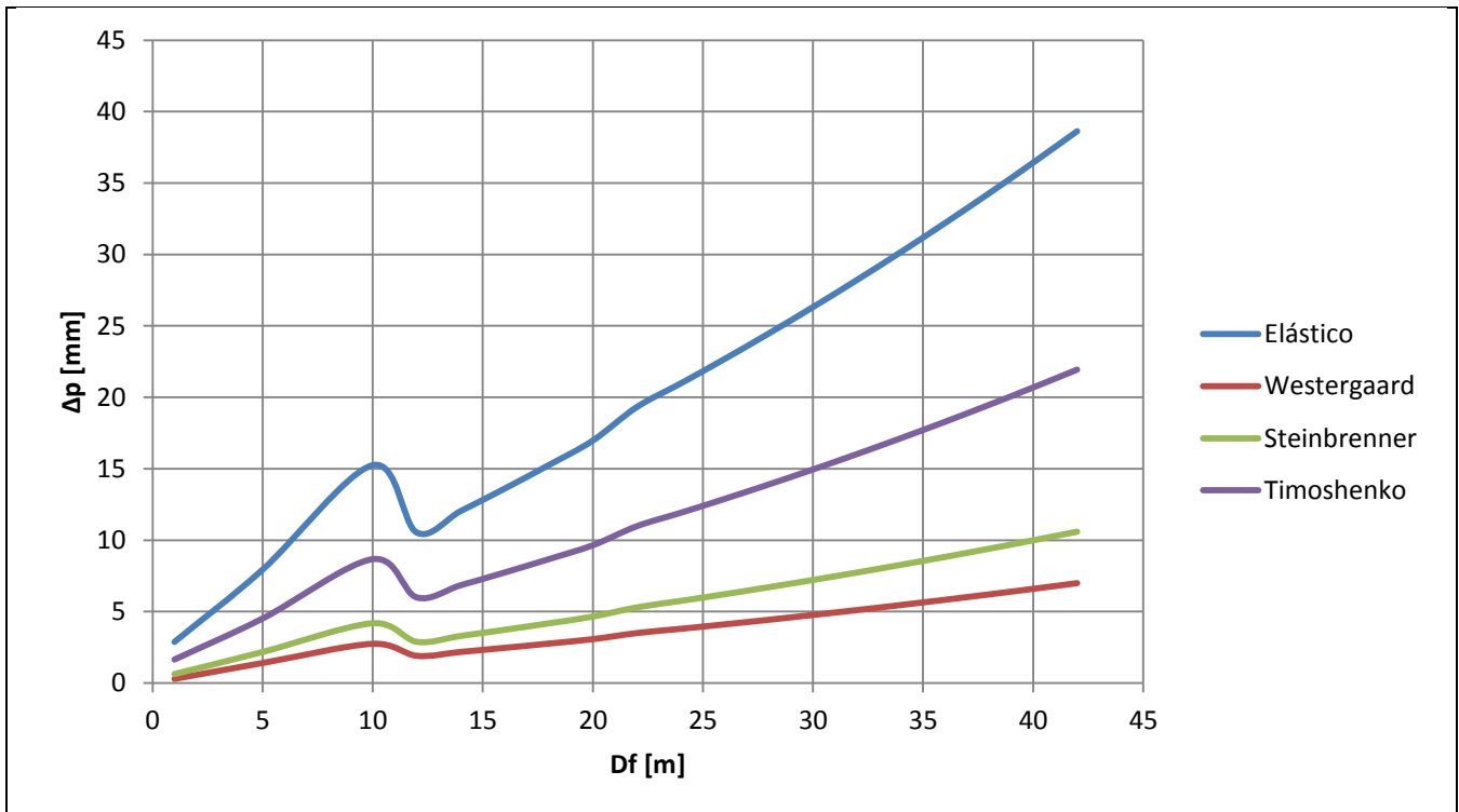
Figura 67, Comparación Asentamientos Timoshenko (D=0.50 m)
