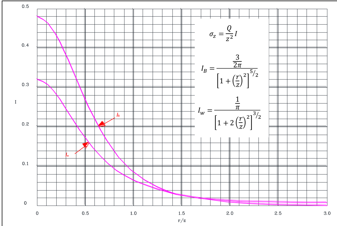
Figura 50, Grafica para Determinar los Esfuerzos Verticales por Medio de los Factores de Influencia de Boussinesq y Westergaard
