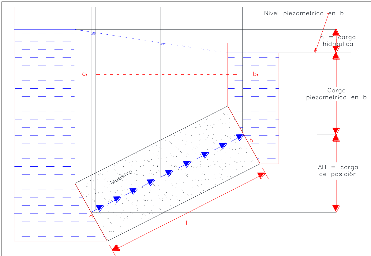
Figura 21, Diagrama que ilustra la Carga Hidráulica, Carga Piezométrica y Carga de Posición
