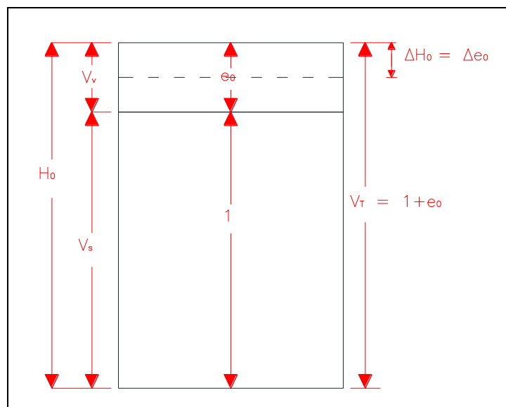
Figura 44, Relación de Vacíos de un Espécimen
