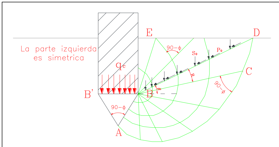
Figura 33, Mecanismos de Falla Meyerhof a Poca Profundidad
