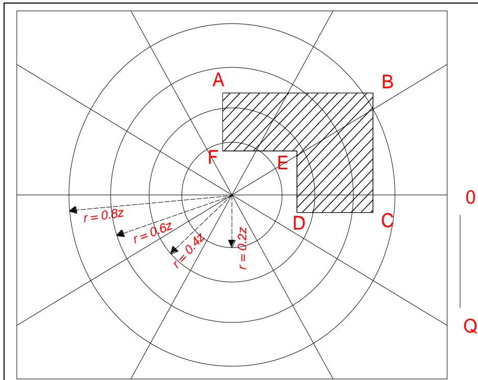
Fuente: Crespo, 2008. Figura 29, Ejemplo Carta de Newmark
