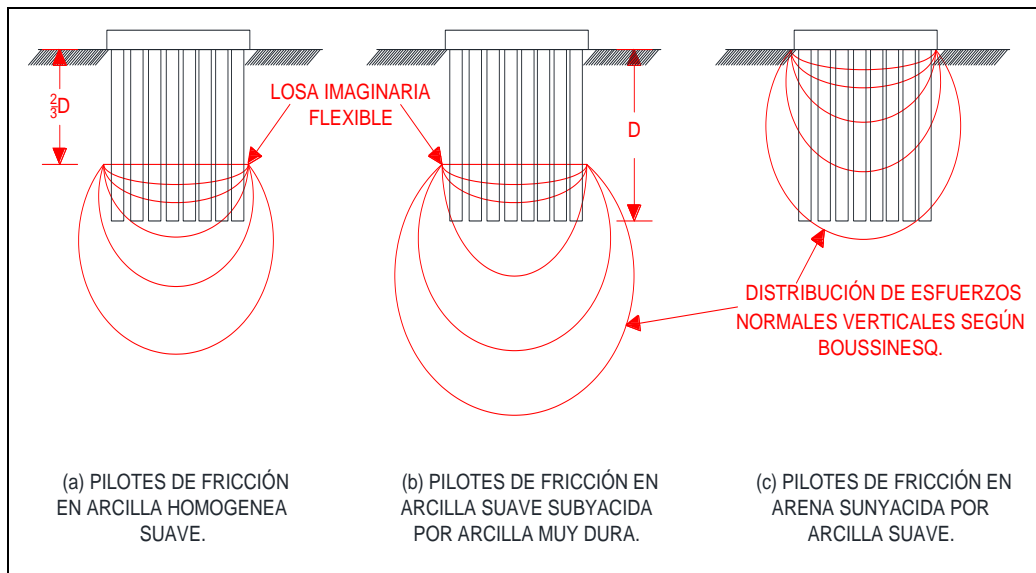
Figura 42, Hipótesis para Calcular la Distribución de Esfuerzos Bajo Grupos de Pilotes de Fricción
