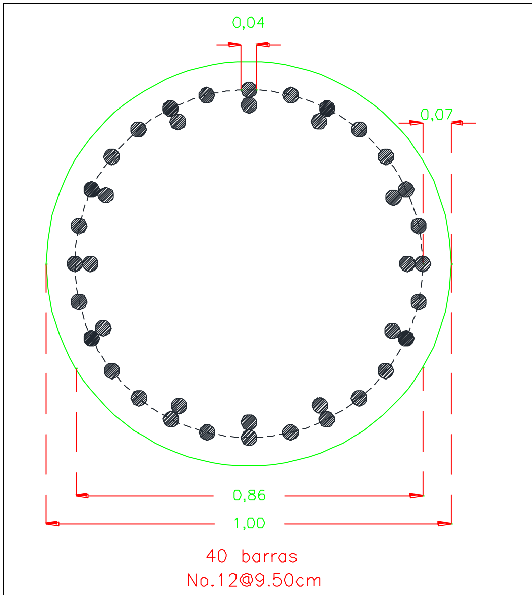
Figura 75, Acero de Refuerzo en Pilas
