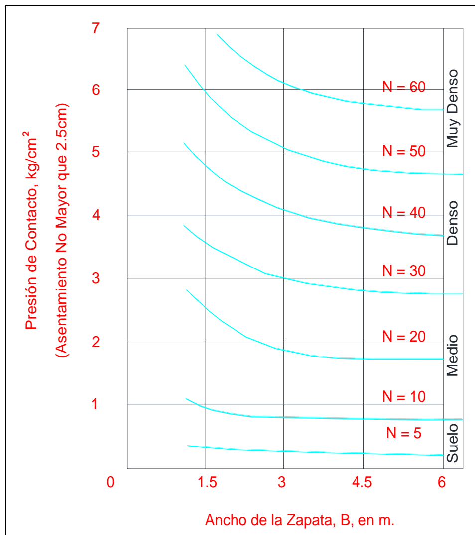
Figura 40, Presión de Contacto Correspondiente a Asentamientos de 1" para Zapatas en Arena
