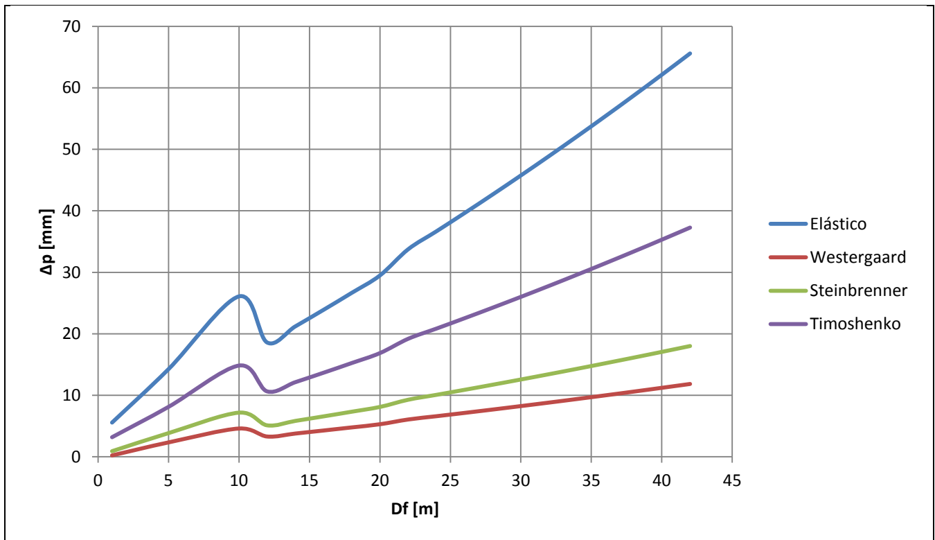
Figura 69, Comparación Asentamientos Timoshenko (D=0.90 m)
