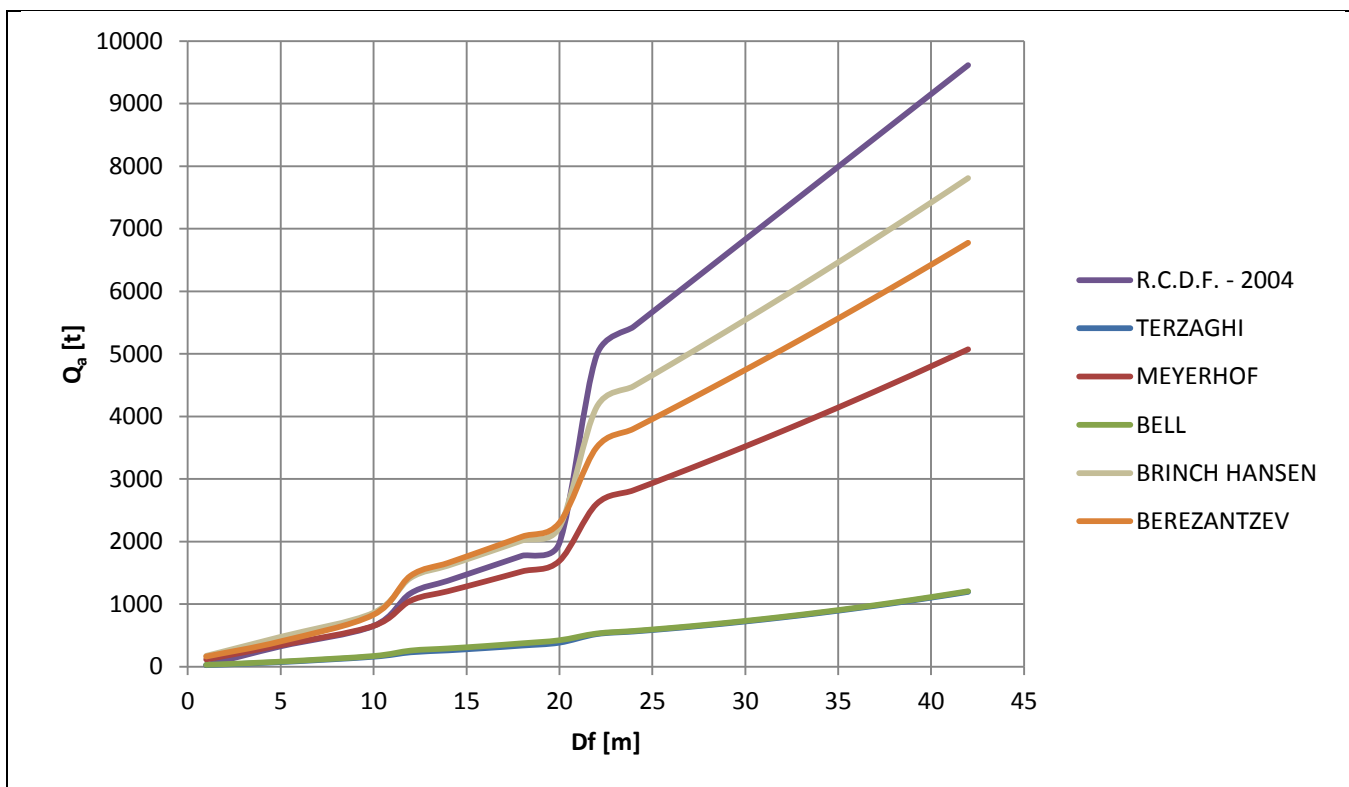
Figura 62, Comparación Teorías Capacidad de Carga (D=1.00 m)
