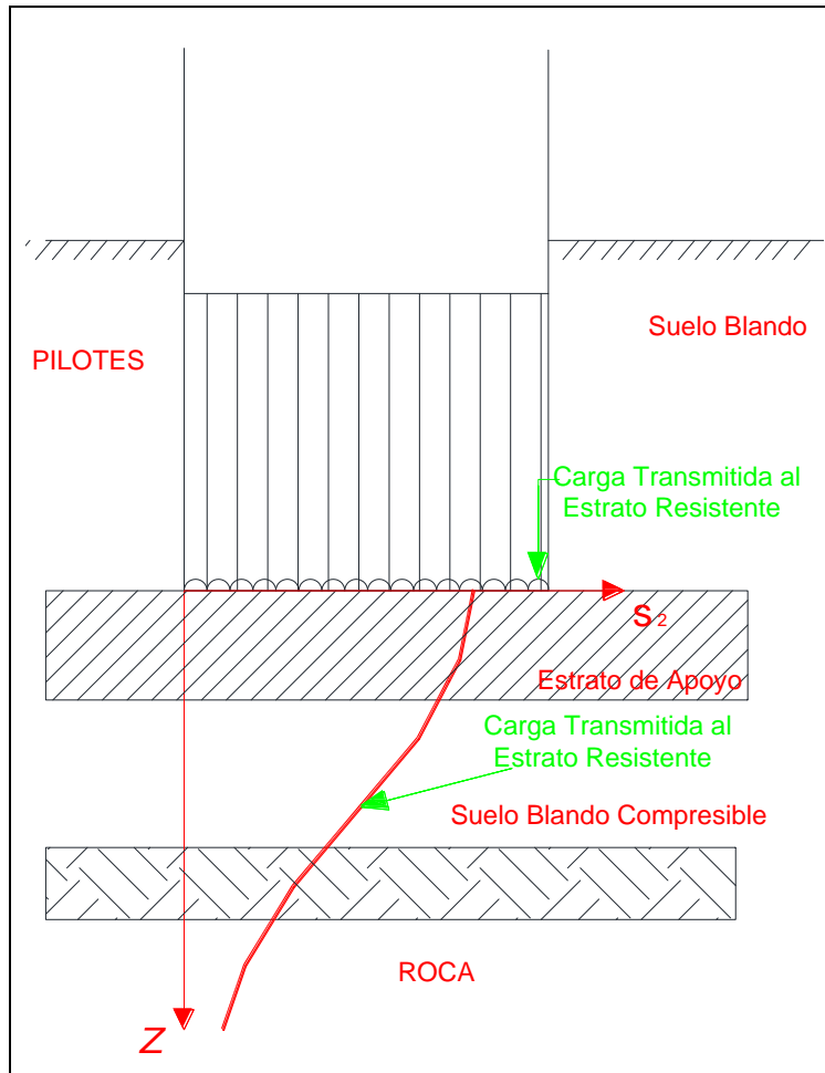
Figura 41, Distribución de Esfuerzos Según Boussinesq para Cimentaciones Profundas
