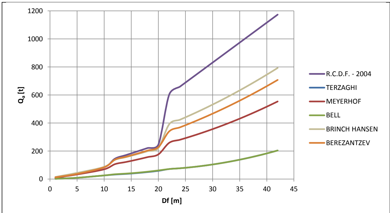
Figura 58, Comparación Teorías Capacidad de Carga (D=0.30 m)
