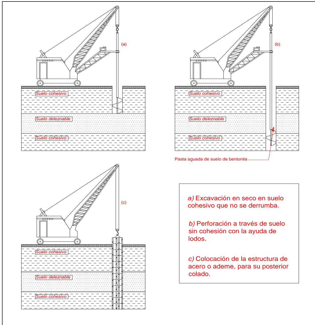
Figura 27, Etapas en la Construcción de una Pila
