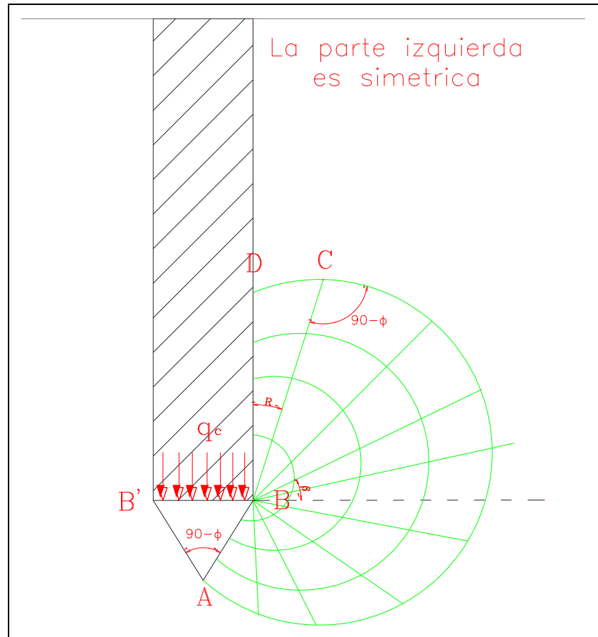
Figura 34, Mecanismos de Falla Meyerhof a Gran Profundidad
