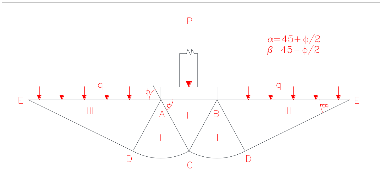
Fuente: Juárez y Rico, 2011. Figura 31, Esquema de las Zonas de Terzaghi
