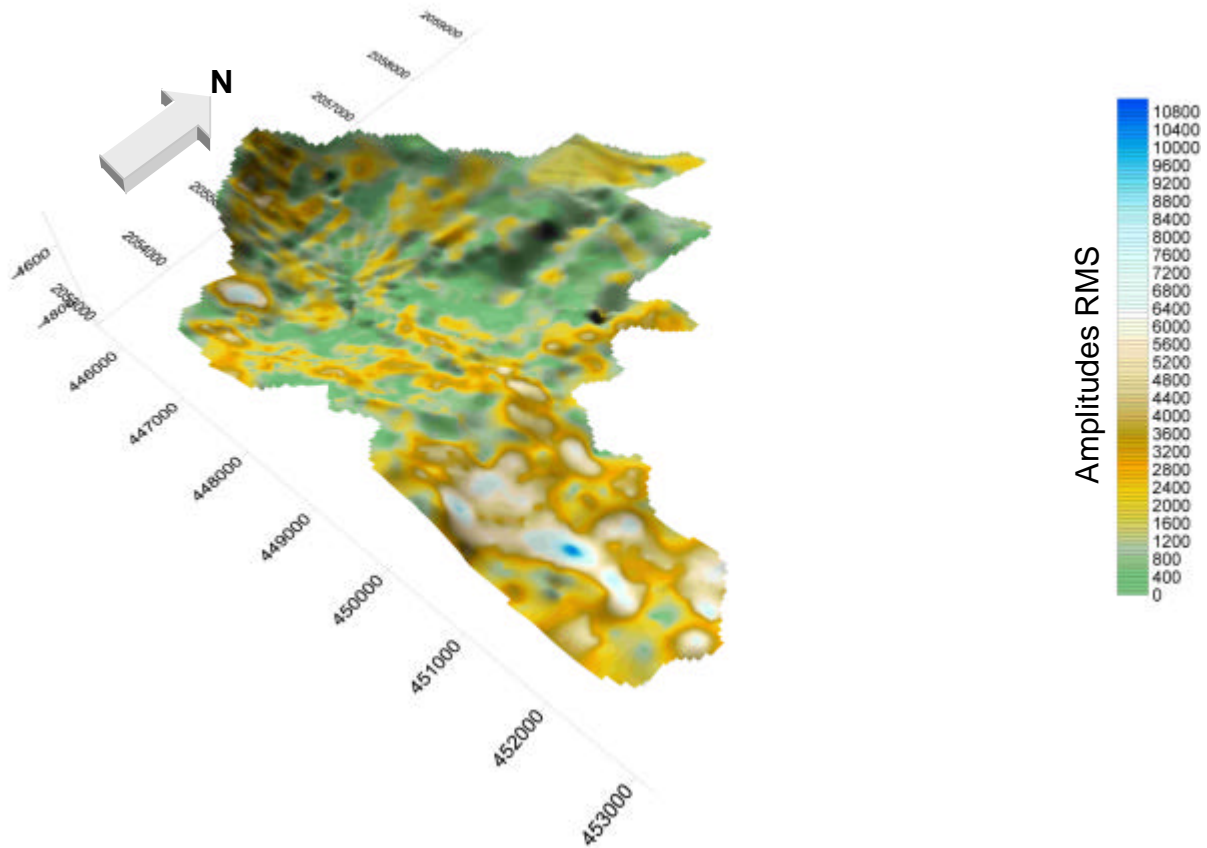
Figura 127. Posición en tiempo de la cima de la facies sísmica asociada a la facies sedimentaria de Flujo de escombros carbonatados A4 montada con los contornos de amplitud RMS asociados a la misma cima. Software SURFER V8.
