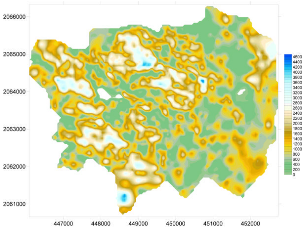
Figura 107. Despliegue de mapa de configuración de Amplitudes RMS de facies sísmicas asociadas a posibles facies sedimentarias de Aprones del rasgo A6 en detalle . Software SURFER V8.
