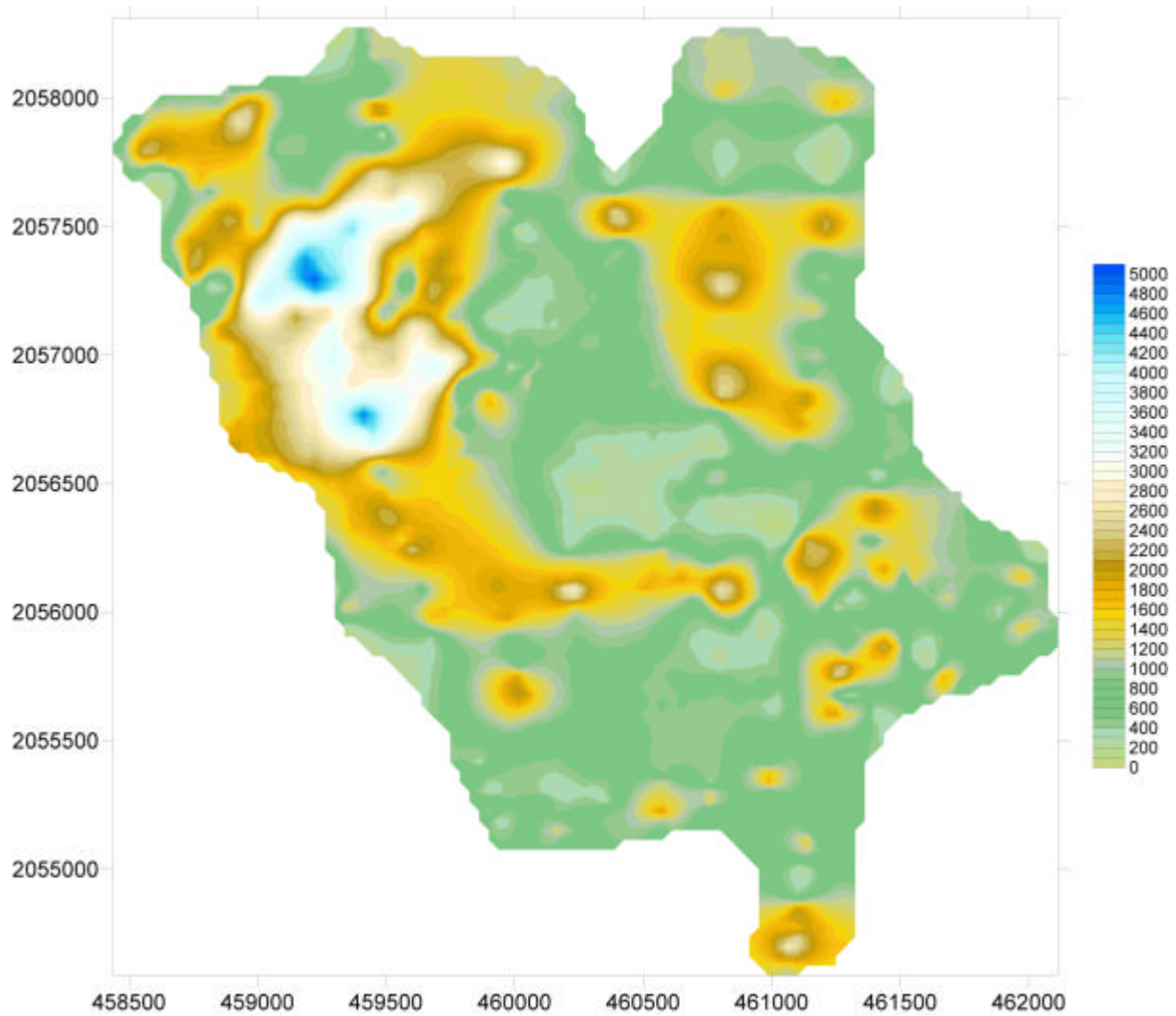
Figura 108. Despliegue de mapa de configuración de Amplitudes RMS de facies sísmicas asociadas a posibles facies sedimentarias de aprones del rasgo A7 en detalle. Software SURFER V8.
