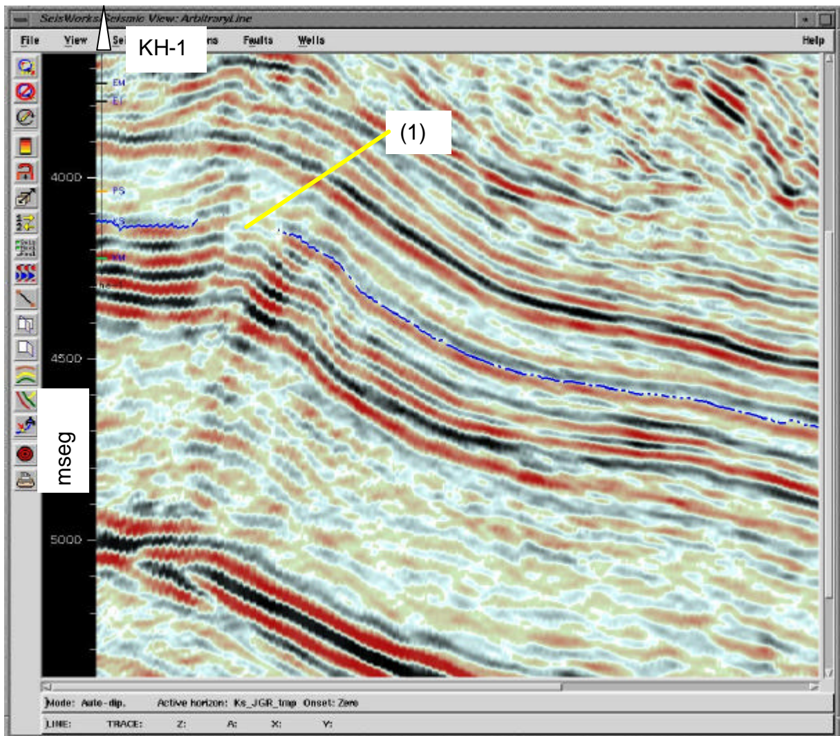
Figura 79. Sección arbitraria que muestra las facies sísmicas con reflexiones discontinuas sobre la superficie picada del Ks. Se indica con el numero (1) la perdida de continuidad en el borde norte de la terraza No. 5. Software Landmark – SeisWorks de Halliburton V2003.
