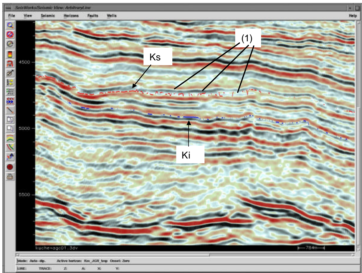
Figura 69. Línea arbitraria, donde se señala para la cima del Ks (rojo) los patrones de reflexión asociables e flujos de escombros indicados con el numero (1). Estos horizontes están calibrados al pozo KH-1 pero el plano de la sección no pasa por el. Software Landmark – SeisWorks de Halliburton V2003.
