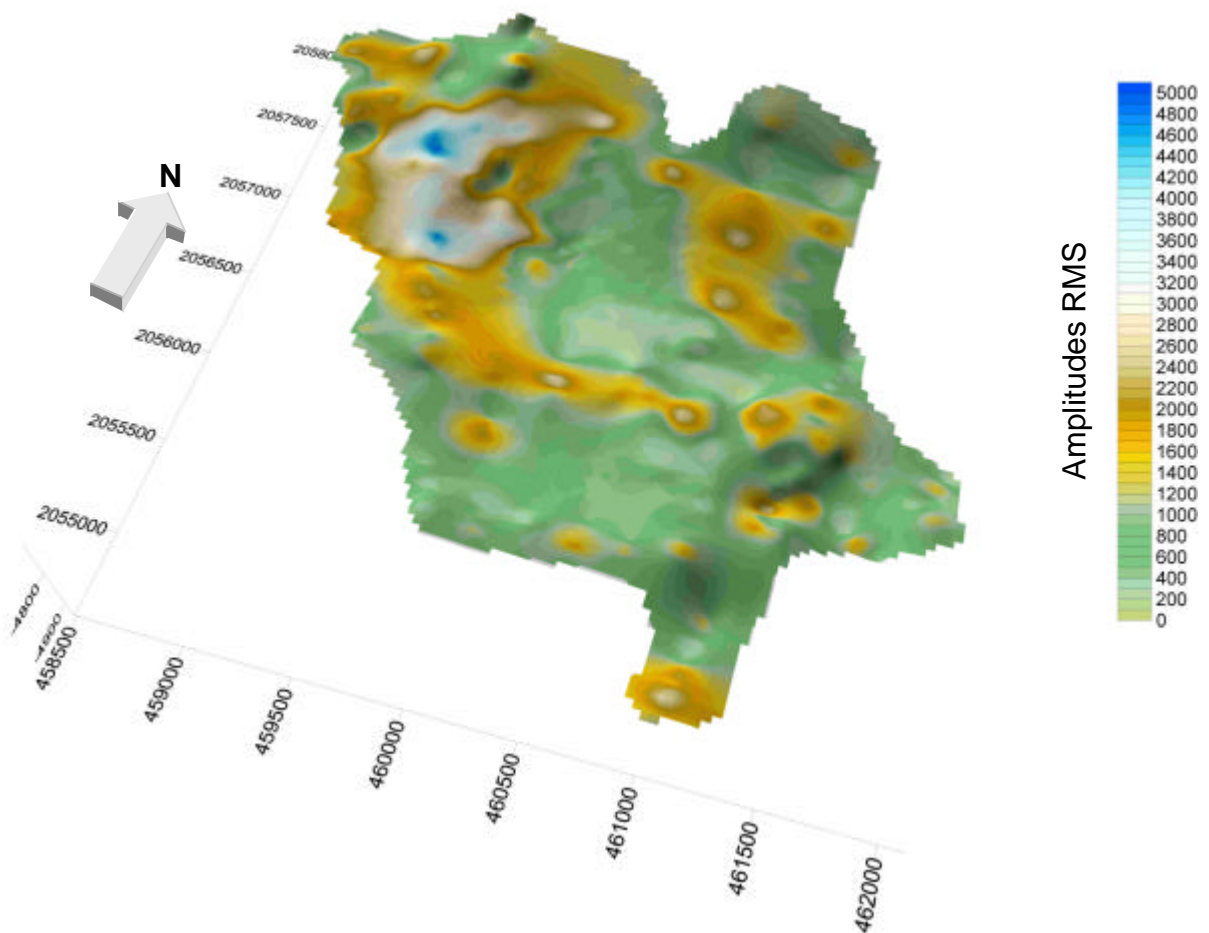
Figura 130. Posición en tiempo de la cima de la facies sísmica asociada a la facies sedimentaria de Flujo de escombros carbonatados A7 montada con los contornos de amplitud RMS asociados a la misma cima. Software SURFER V8.
