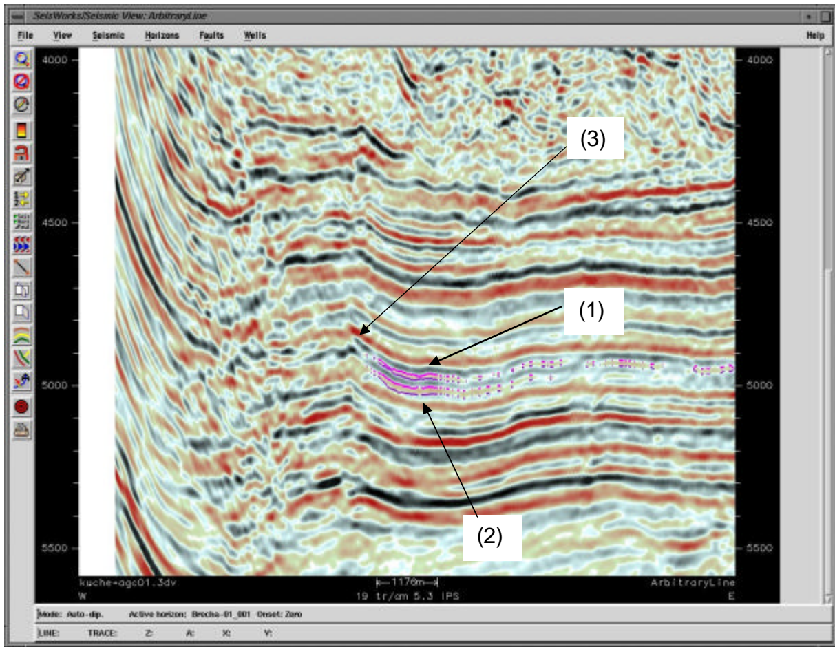
Figura 84. Sección arbitraria que muestra los 2 flujos de escombros con los números (1) y (2) provenientes de lo que podría ser un perfil depositacional sismoestratigráfico asociable a un margen de borde de plataforma en la parte NW del área y que esta cerca de la zona de afectación de la falla inversa al NW de la zona de estudio, mas sin embargo, la sección demuestra la existencia de un borde de perfil de deposito que origina los colapsos descritos (3). Software Landmark – SeisWorks de Halliburton V2003.
