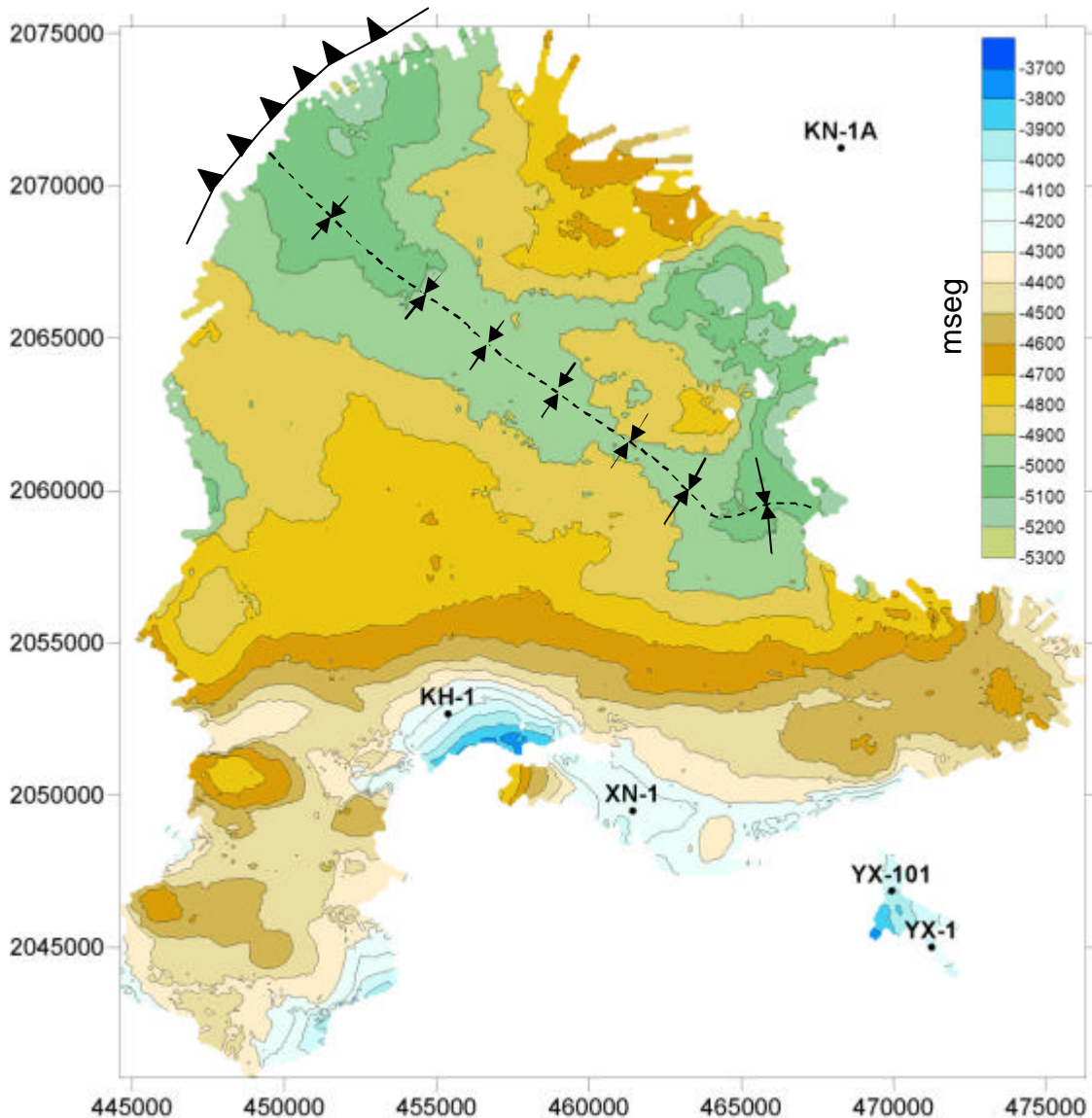
Figura 55. Mapa de contornos del Ks. producto de la aplicación de Krigging en una malla de 80 por 80m y un radio de búsqueda de 200m. Se denota el eje del pequeño bajo sinclinal. Software SURFER V8.
