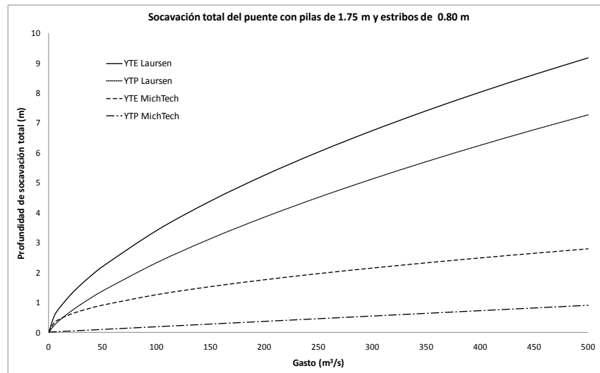
Figura 67. Socavación total para puente tipo 6
