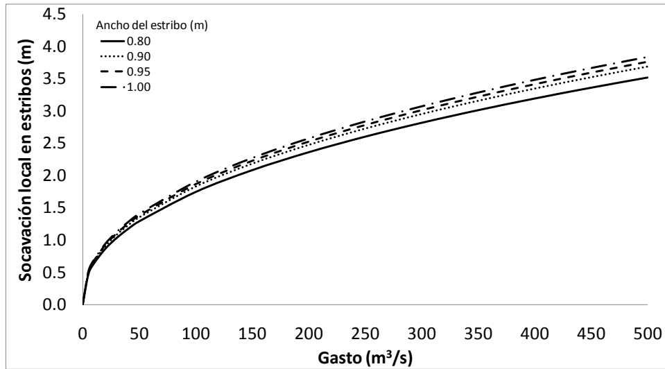
Figura 46. Socavación local en estribos puente tipo 1
