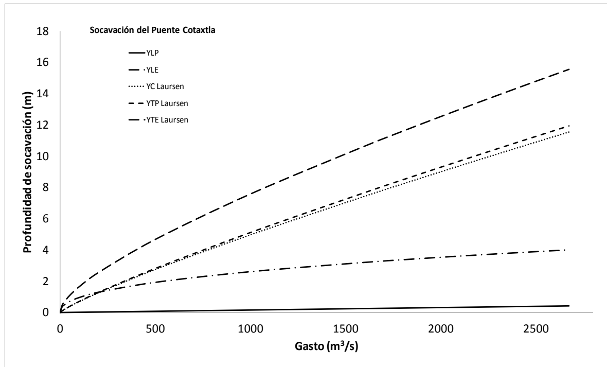
Figura 77. Socavación puente Cotaxtla (Laursen)
