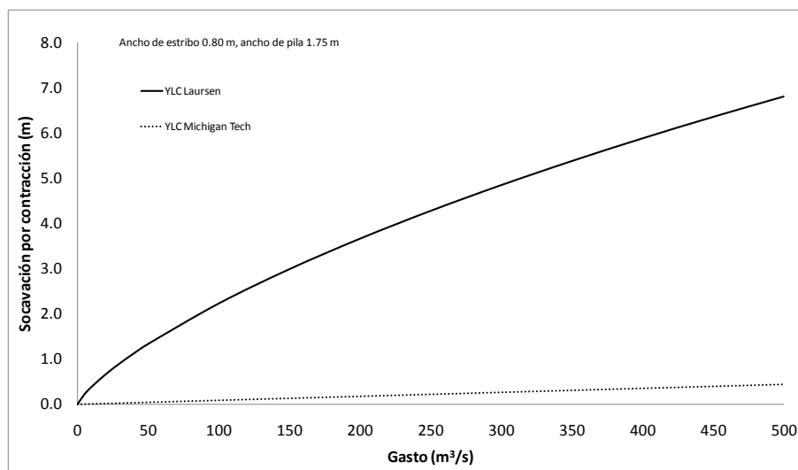
Figura 66. Socavación por contracción de puente tipo 6
