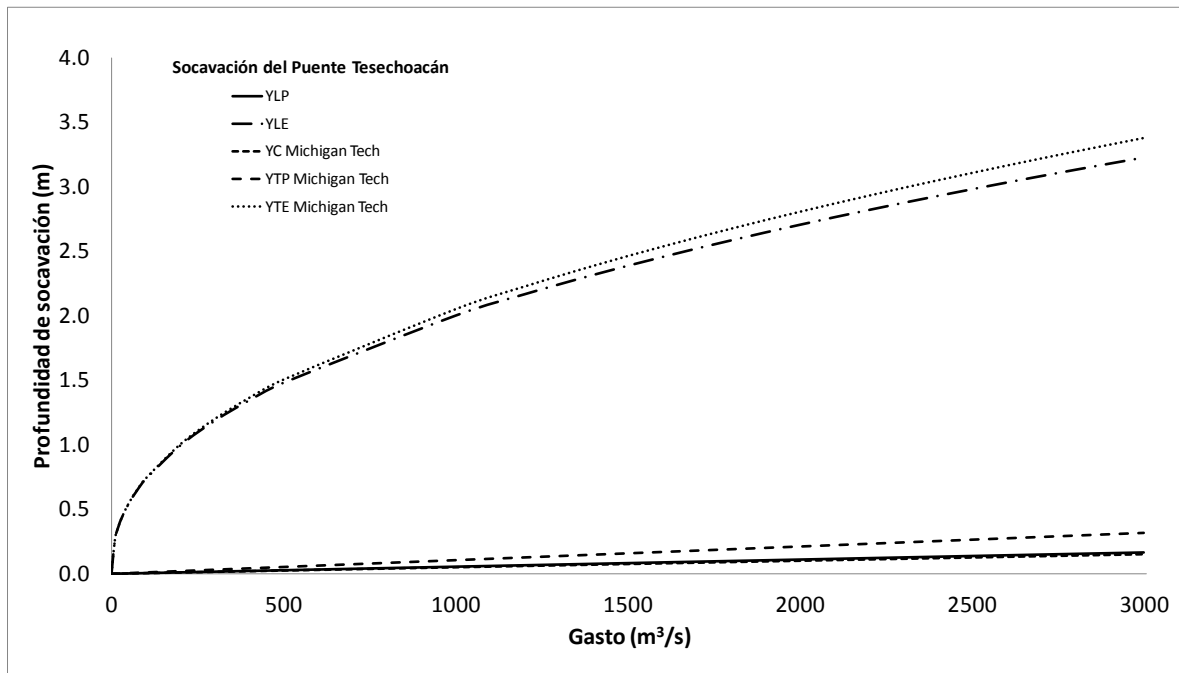
Figura 84. Socavación del puente Tesechoacán (Michigan Tech)
