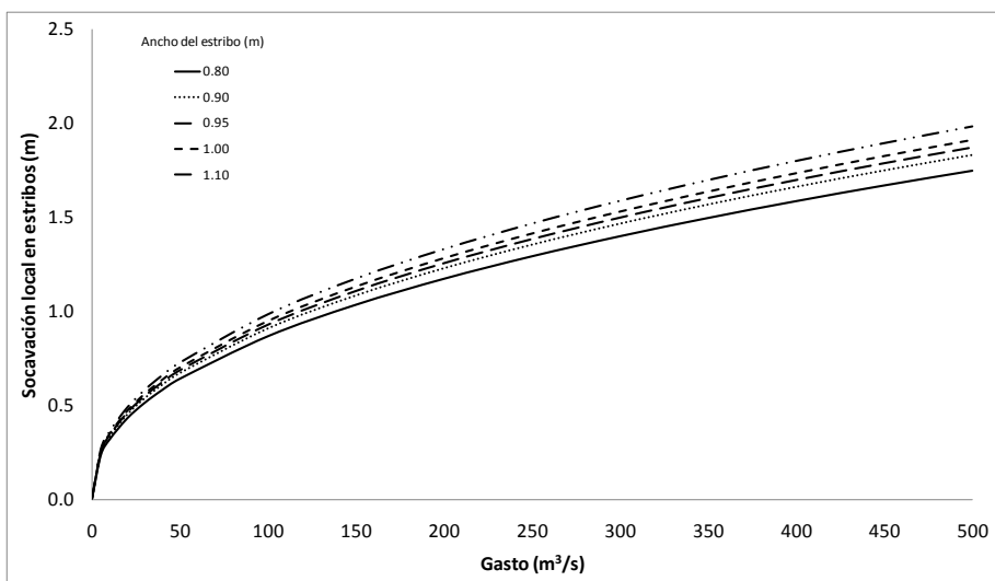
Figura 72. Socavación local en estribos para puente de 50m
