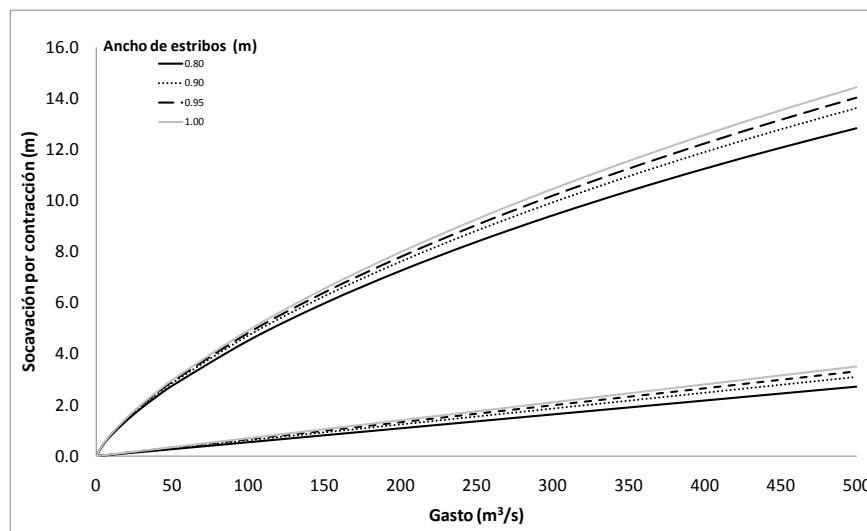
Figura 49. Comparación de socavación por contracción de las dos expresiones empleadas para puente tipo 1
