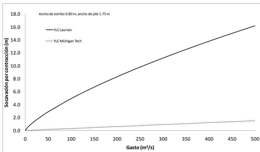
Figura 62. Socavación por contracción (Laursen y Michigan Tech) para puente tipo 4
