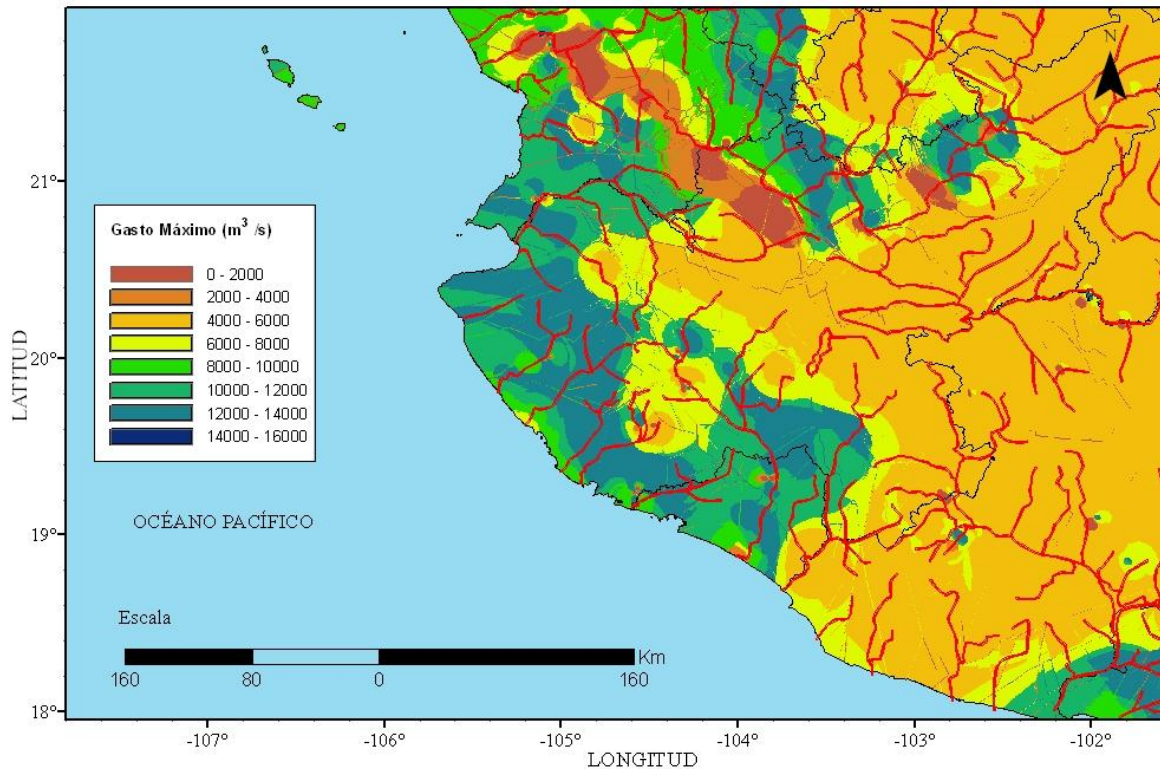
Figura 31. Variación del gasto ( m^3/s )
