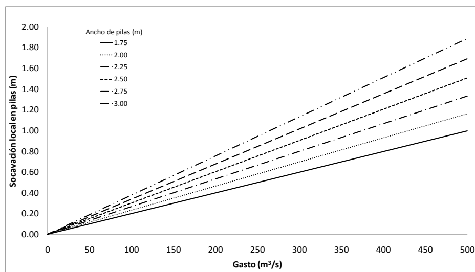
Figura 68. Socavación local en pilas para puente de 25m, apoyado en 2 pilas
