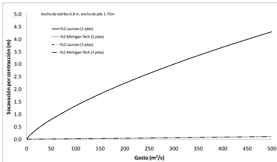
Figura 75. Socavación por contracción para puente de 50m
