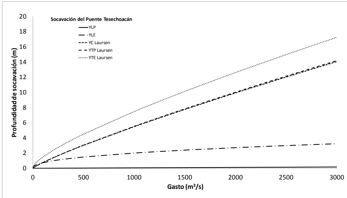
Figura 83. Socavación del puente Tesechoacán (Laursen)
