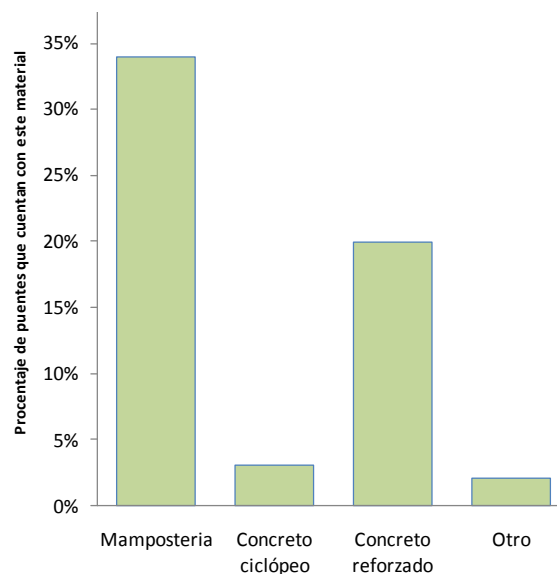
Figura 40. Clasificación de los puentes de acuerdo al material en las pilas
