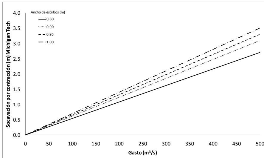
Figura 48. Socavación por contracción (Michigan Tech) para puente tipo 1
