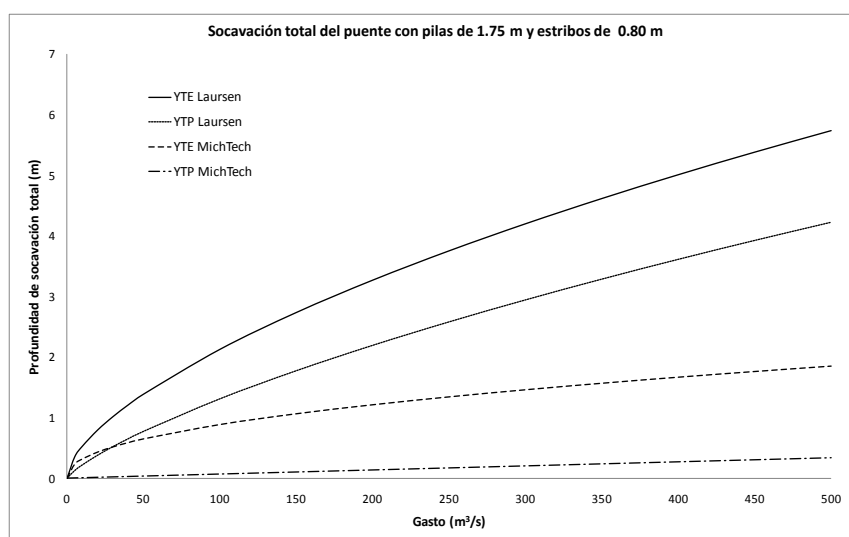
Figura 76. Socavación total para puente de 50m, apoyado en 2 pilas
