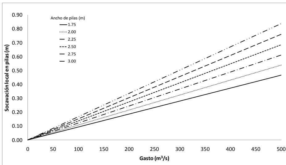
Figura 64. Socavación local en pilas de puente tipo 6
