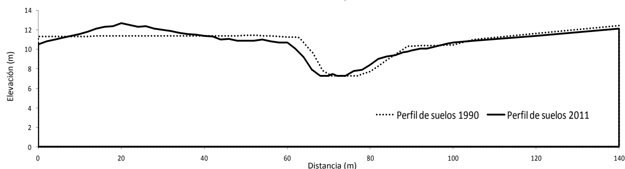
Figura 82. Croquis de los perfiles de suelos del puente Poposoca
