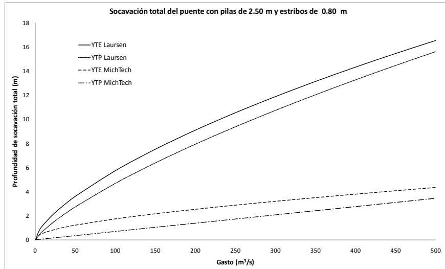
Figura 59. Socavación total puente tipo 2 con estribos de 0.8m y pila de 2.5m
