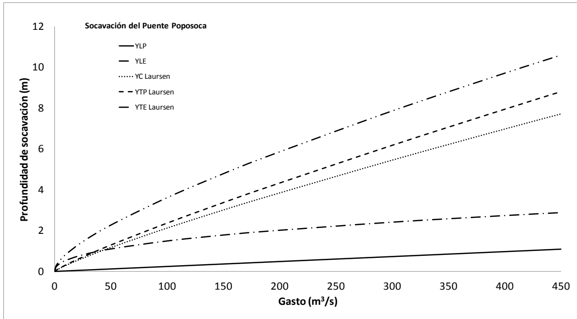
Figura 80. Socavación del puente Poposoca (Expresión de Laursen)
