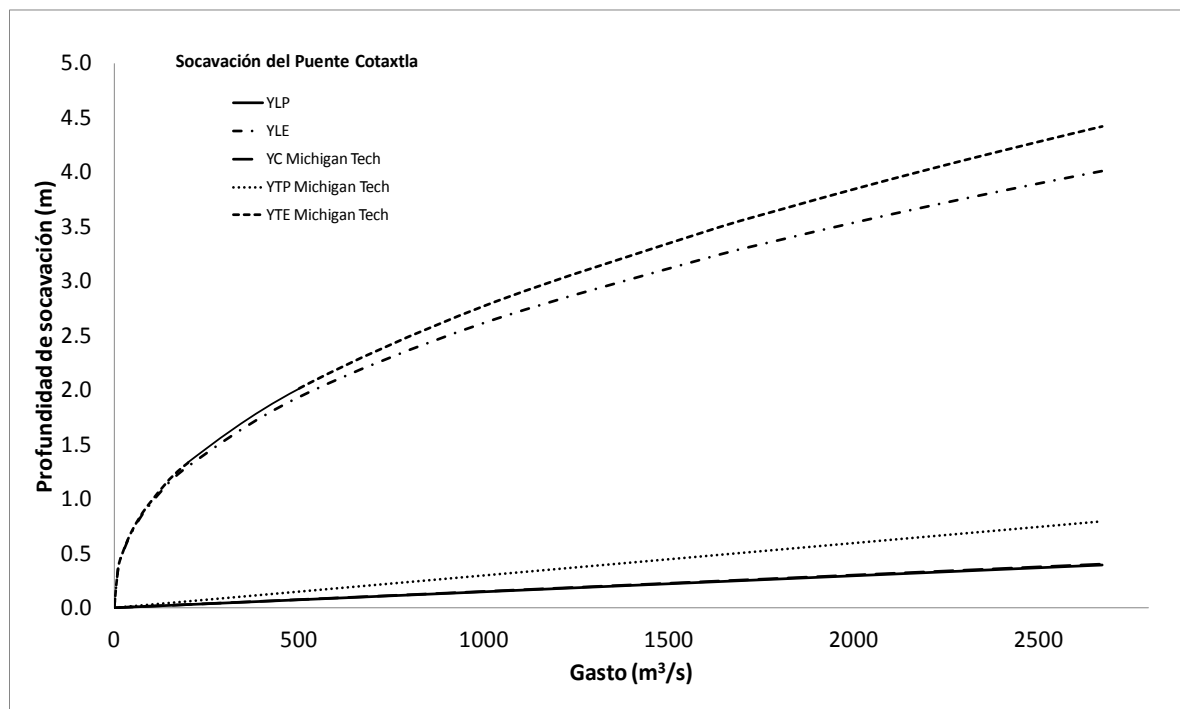
Figura 78. Socavación puente Cotaxtla (Michigan Tech)
