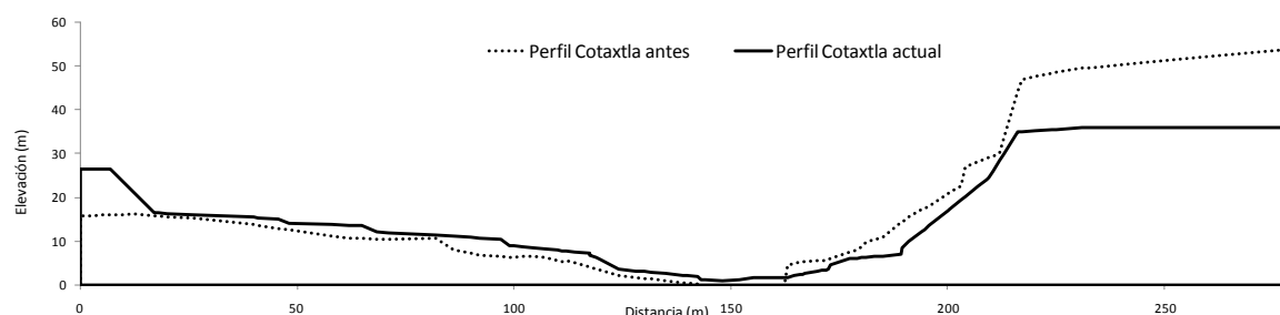
Figura 79. Croquis de los perfiles del puente Cotaxtla
