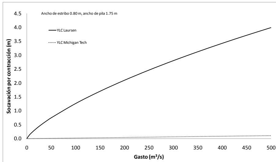
Figura 73. Socavación por contracción para puente de 50m, apoyado en 2 pilas
