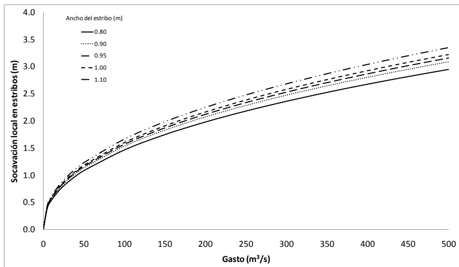
Figura 61. Socavación local en estribos para puente tipo 4
