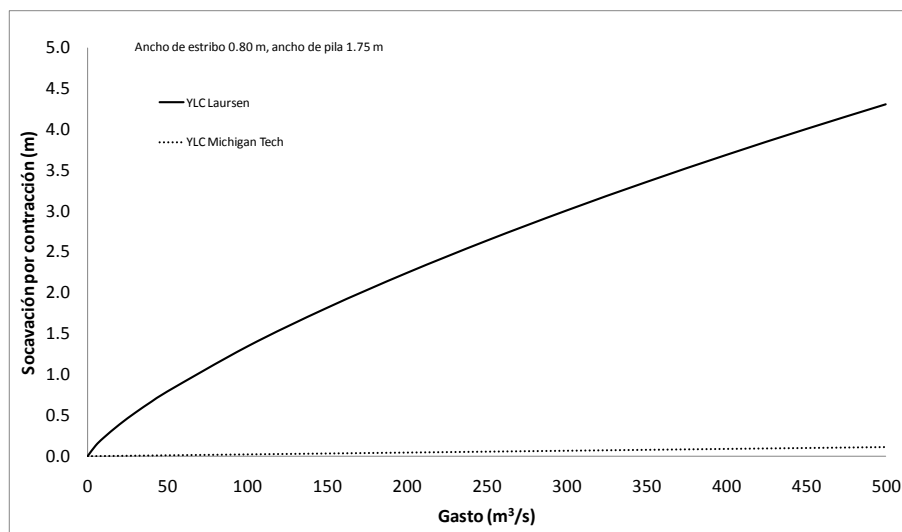
Figura 74. Socavación por contracción para puente de 50m, apoyado en 3 pilas
