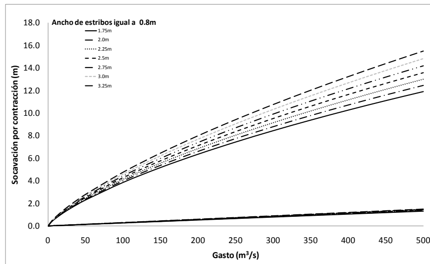
Figura 57. Socavación por contracción, Laursen y Michigan Tech
