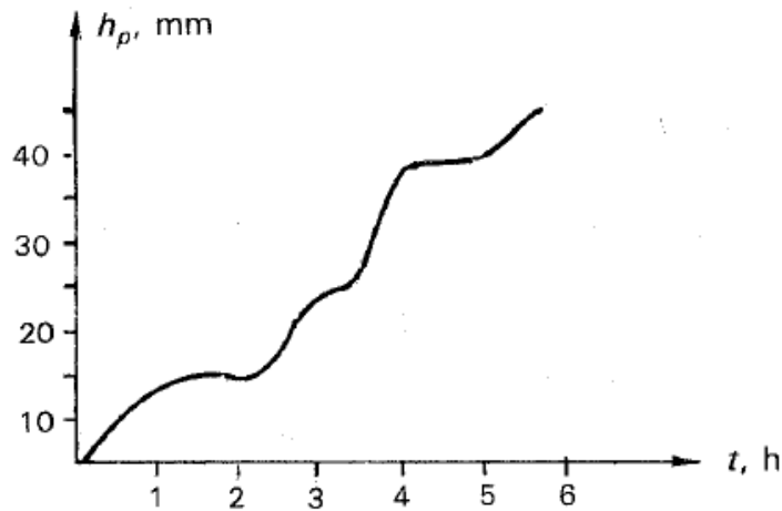
Figura 2.14 Curva masa.
