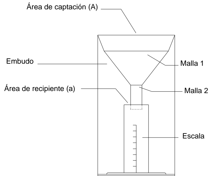
Figura 2.1 Pluviómetro. APARICIO
