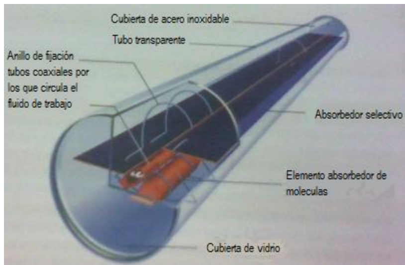
Figura 2.4 Sección de un tubo de vacío de flujo directo.
