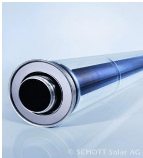
Figura 2.3 Tubo de vacío Schott.
