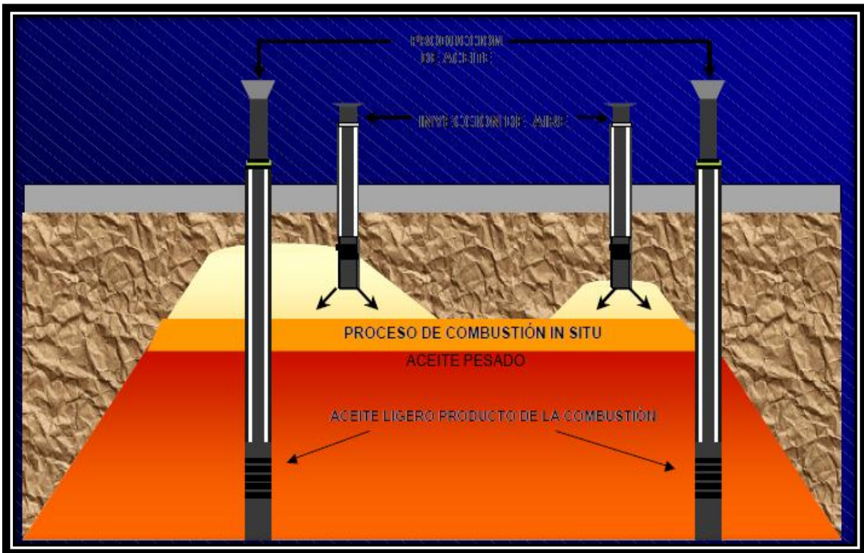
Figura 3.9 Proceso de Recuperación mejorada, inyección de aire.
