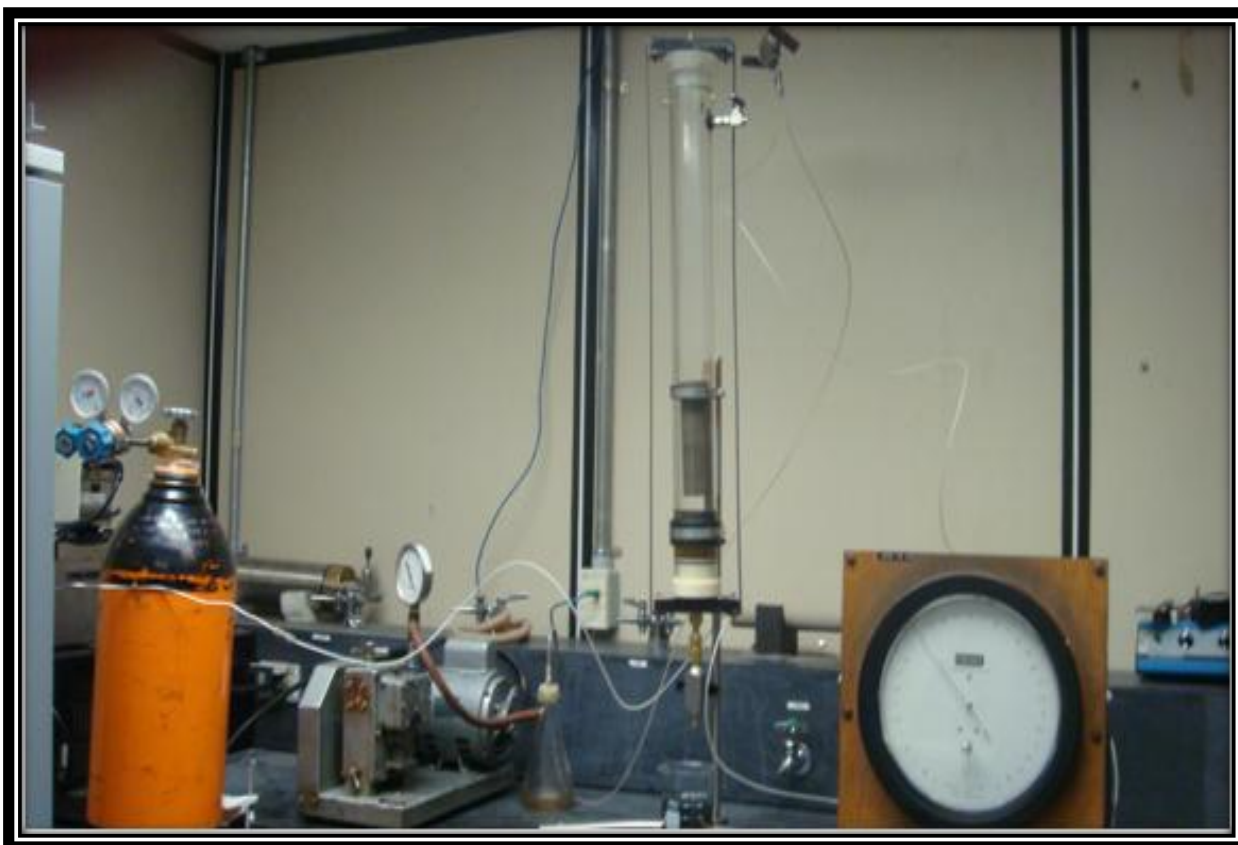
Figura 5.19 Sistema experimental para el desplazamiento con N 2 .
