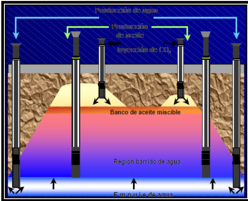
Figura 3.8 Proceso de Recuperación mejorada, doble desplazamiento.
