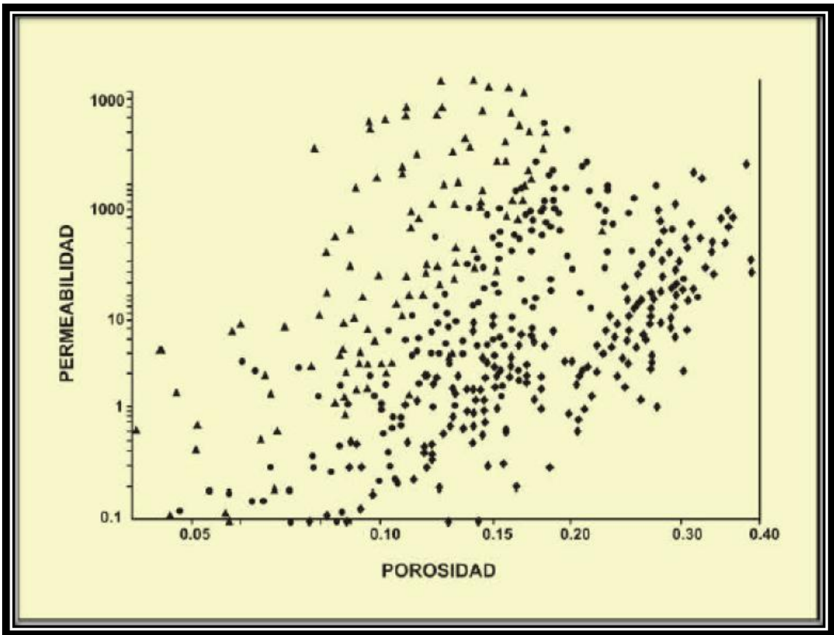
Figura 3.6 Comportamiento de la Relación de Permeabilidad-Porosidad para Carbonatos 5 .
