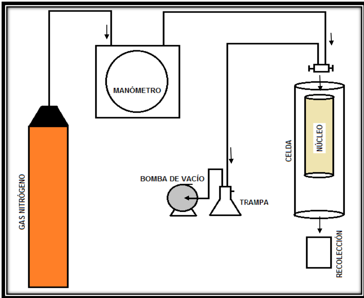
Figura 5.4 Diagrama esquemático del sistema experimental.
