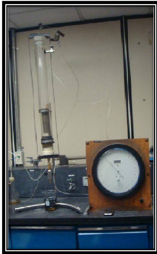
Figura 5.16 Sistema experimental para el experimento # 3.
