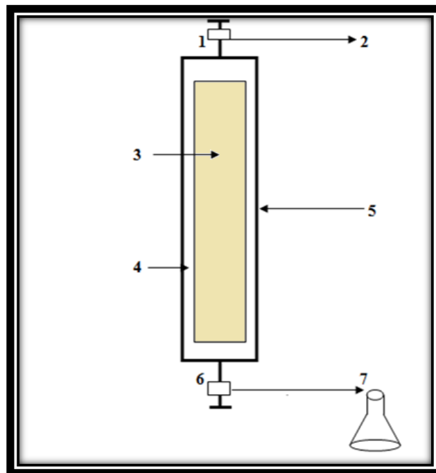
Figura 5.1 Esquema de la celda experimental.
