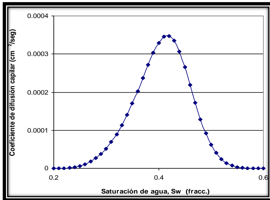
Figura 4.2 Comportamiento del coeficiente de difusión capilar en función de la saturación y modelando la presión capilar usando el modelo de Abbas Firoozabadi 6 .
