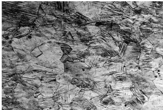
Figura 1.2. Micrografía del Acero inoxidable 316L [12].
