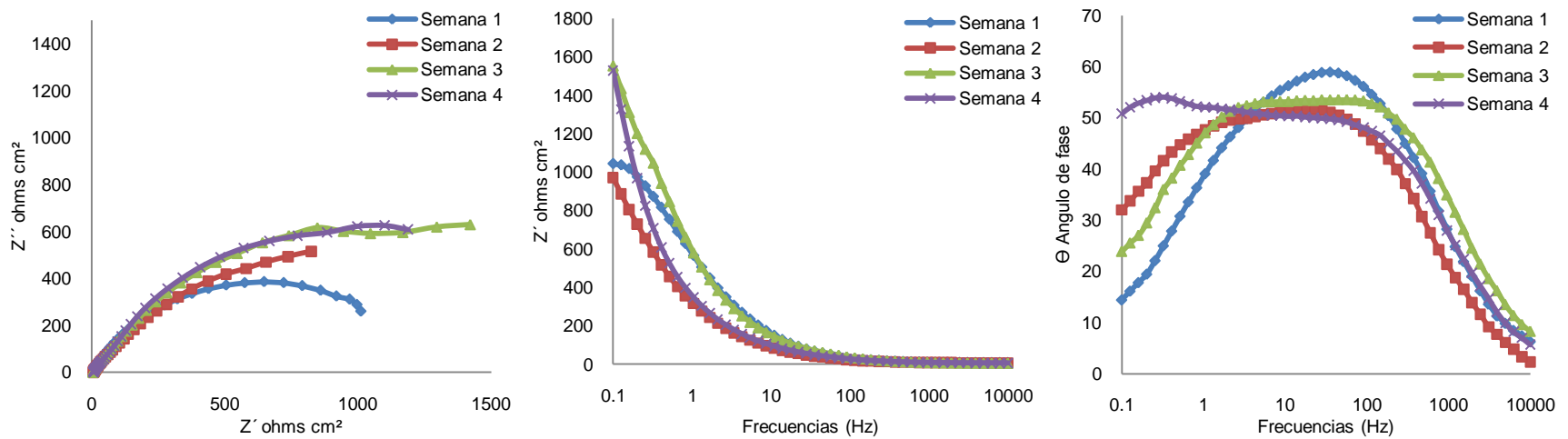
Figura 3.15. Diagrama de Nyquist y Bode de la aleación Ti-6Al-4V en solución Ringer B a 37°C en condiciones estáticas.
