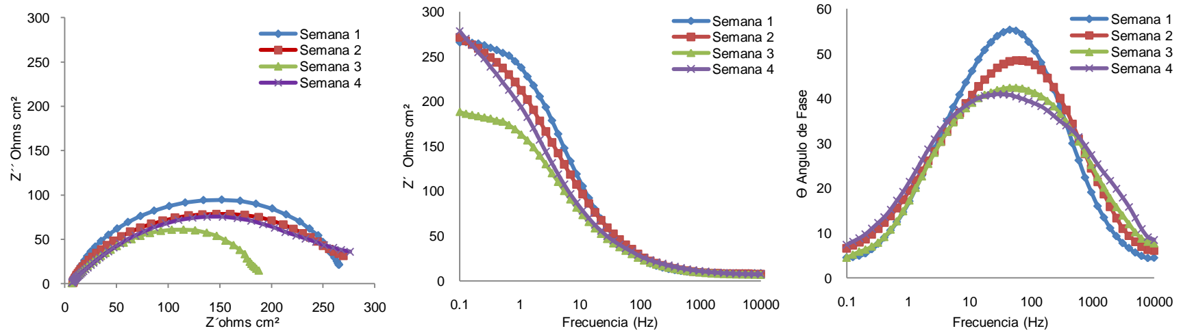
Figura 3.4. Diagrama de Nyquist y Bode de la aleación Co-Cr-Mo en solución Tyrode a 37°C en condiciones estáticas.
