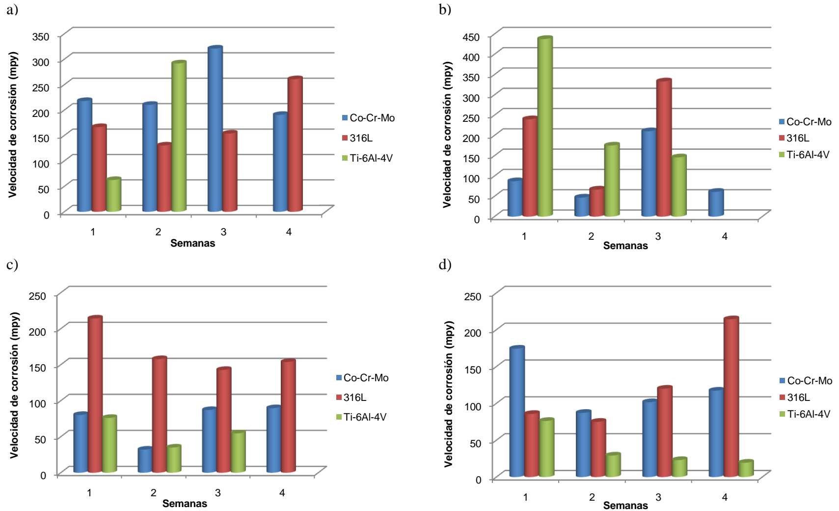
Figura. 3.16. Gráficas de Velocidad de corrosión (mpy) en función del tiempo para las aleaciones Co-Cr-Mo, acero 316L y Ti-6Al-4V, en las diferentes soluciones; a) Tyrode , b) Isotónica, c) Ringer A y d) Ringer B
