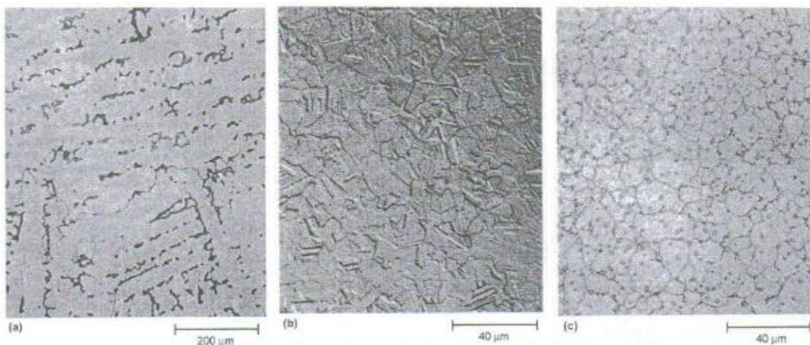
Figura 1.4. Microestructuras de aleaciones Co-Cr-Mo. (a) Modelo de revestimiento con carburos secundarios y tamaño de grano grande (ASTM tamaño 7.5) (b) Alta resistencia de grano fino forjado con refuerzo de nitrógeno (c) Isostáticamente trabajado en caliente a partir de polvo prensado [21].
