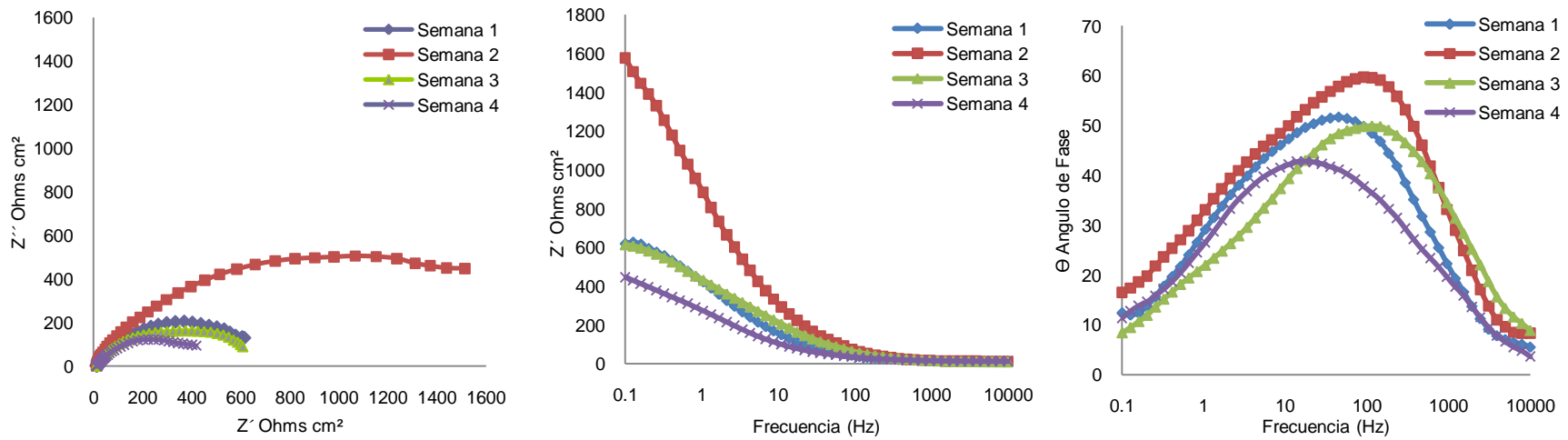
Figura 3.7. Diagrama de Nyquist y Bode de la aleación Co-Cr-Mo en solución Isotónica a 37°C en condiciones estáticas.
