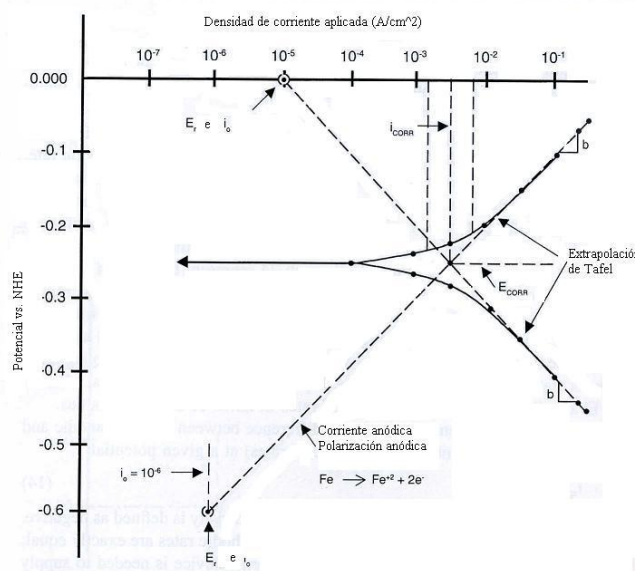
Figura I-1: Extrapolación de Tafel para predecir velocidades de corrosión [25].
