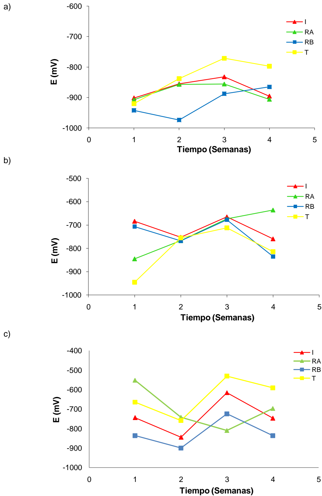
Figura 3.2. Diagramas de OCP, a) Co-Cr-Mo, b) 316L y c) Ti-6Al-4V en las diferentes soluciones Isotónica, Ringer A, Ringer B y Tyrode a 37°C en condiciones estáticas
