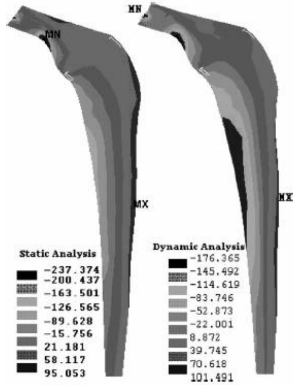
Figura 1.7. Comparación de las tensiones de tracción axiales máximas y mínimas en una prótesis de cadera en condiciones estática y dinámica [23].
