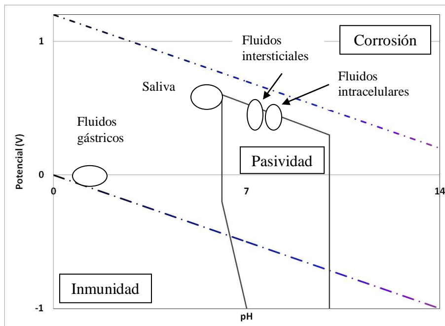
Figura 1.3. Diagrama de Pourbaix para el Cromo, destacando las zonas con diferentes fluidos corporales [15].
