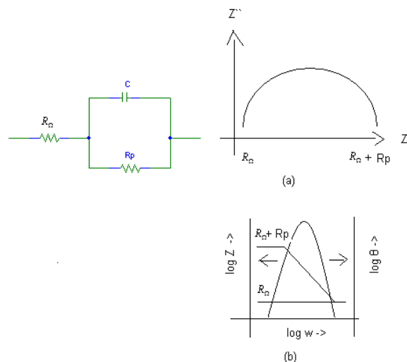
Figura 1-2: Gráficos obtenidos a partir del circuito mostrado que simula un electrodo que es corroído: (a)Gráfico de Nyquist; (b)Gráfico de Bode; ambos esquemáticos [27].
