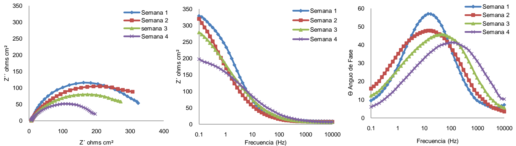
Figura 3.5. Diagrama de Nyquist y Bode del acero inoxidable 316L en solución Tyrode a 37°C en condiciones estáticas.
