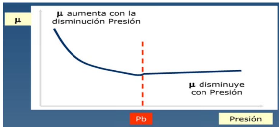
Fig. 2.8.4 Gráfica del Comportamiento de la Viscosidad.
