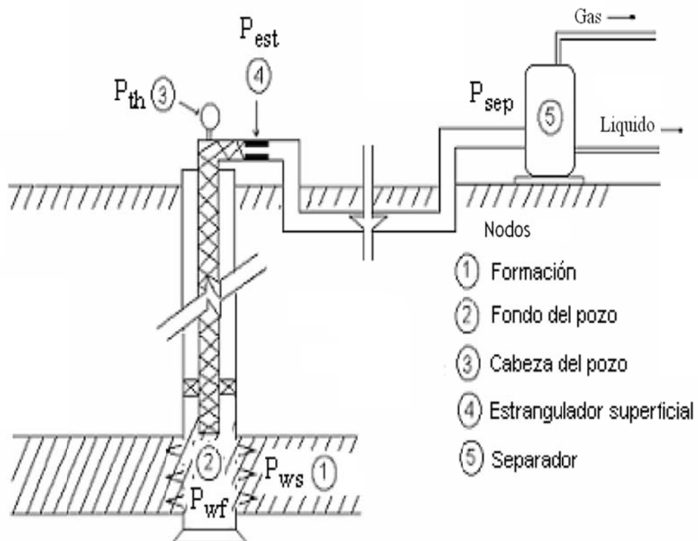
Fig. 3.3.1 Sistema Integral de Producción.
