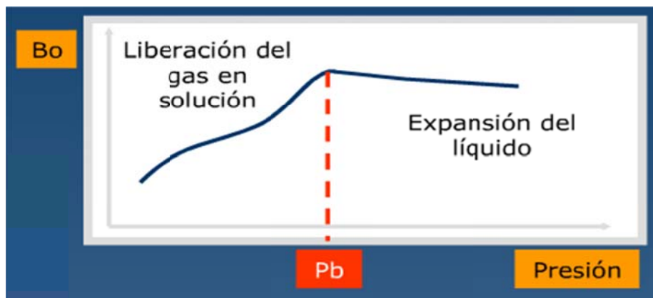
Fig. 2.8.3 Gráfica Factor de Volumen de Aceite.
