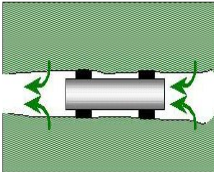
Fig. 3.8.1 Terminación en agujero abierto.
