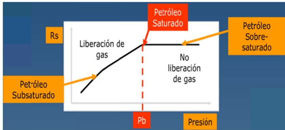
Fig. 2.8.2 Gráfica Relación de Solubilidad.
