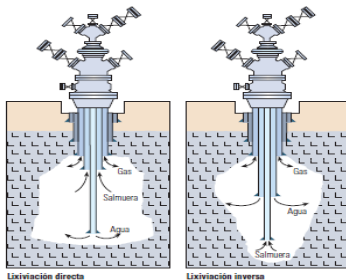
Fig. 4.15 Procesos de lixiviación (Schlumberger 2003).
