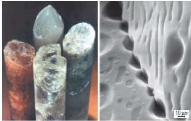
Fig. 4.14 Núcleos salinos ( izquierda ) y fotomicrografía ( derecha ) (Schlumberger 2003).
