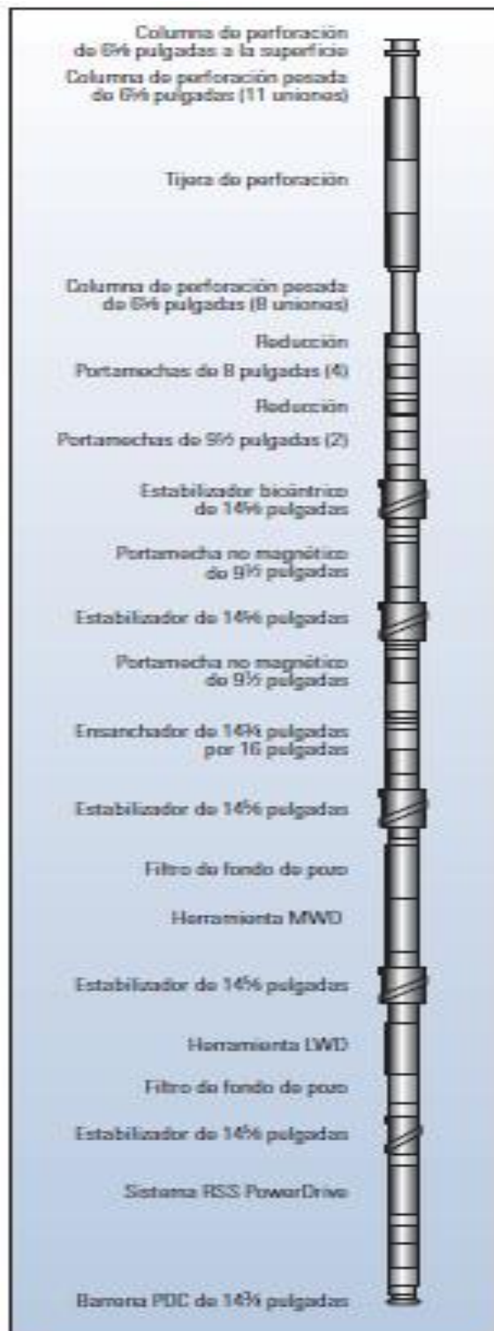
Fig. 4.8 BHA construido especialmente para una operación determinada en el Golfo de México (Schlumberger, 2008).
