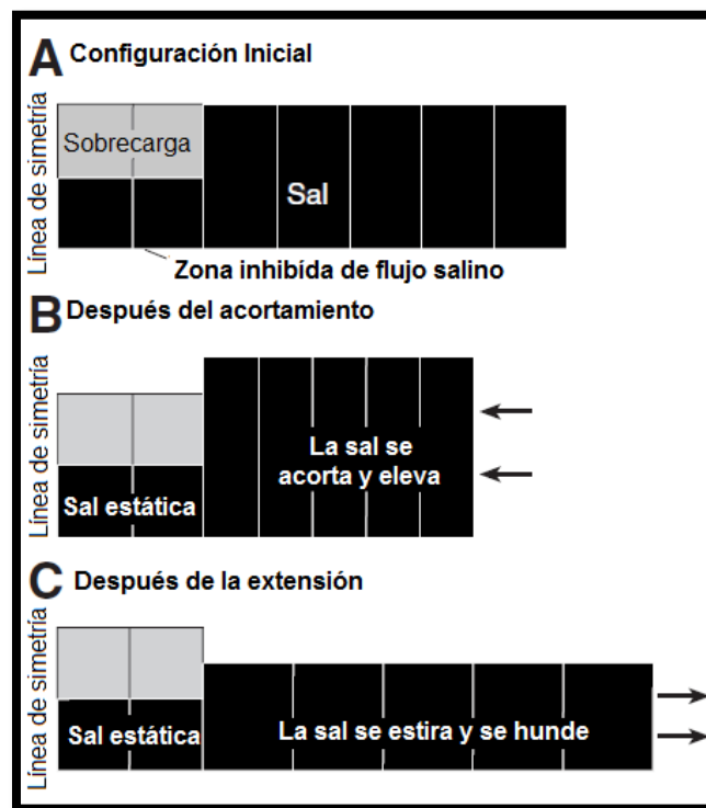
Fig. 2.38 Diagrama esquemático que explica cómo afecta el acortamiento y la extensión a una minicuenca (Hudec, 1995).
