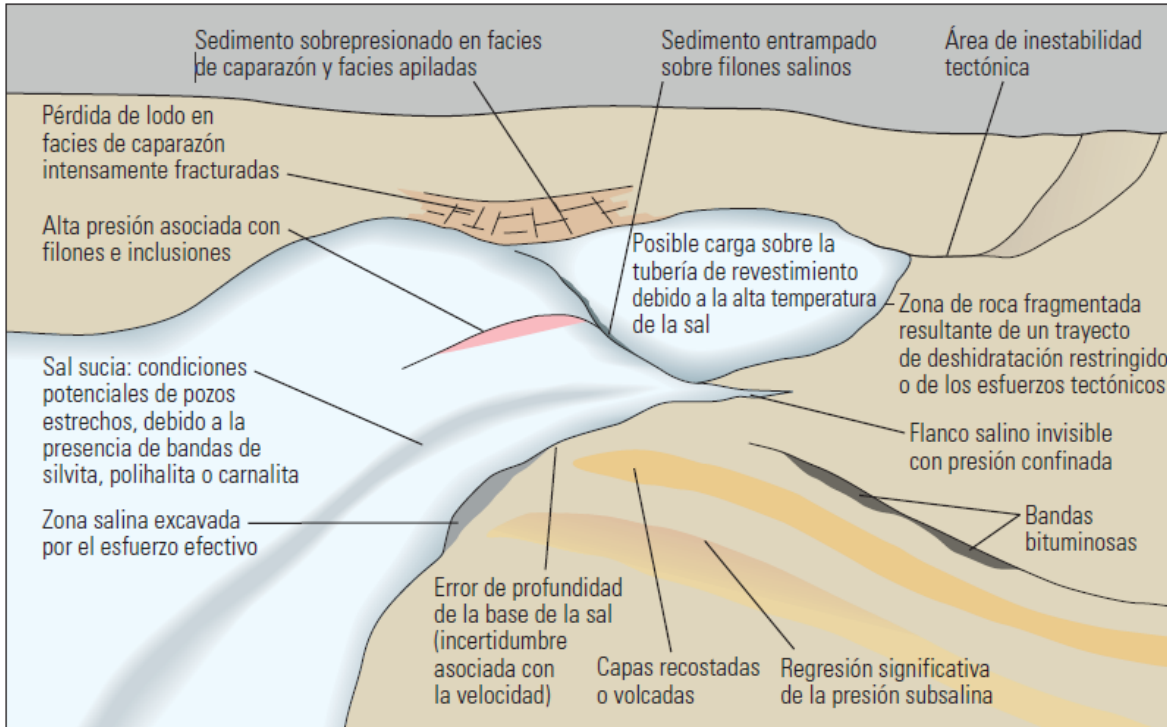
Fig.4.1 Riesgos potenciales de perforación en la sal y sus adyacencias (Schlumberger, 2008).
