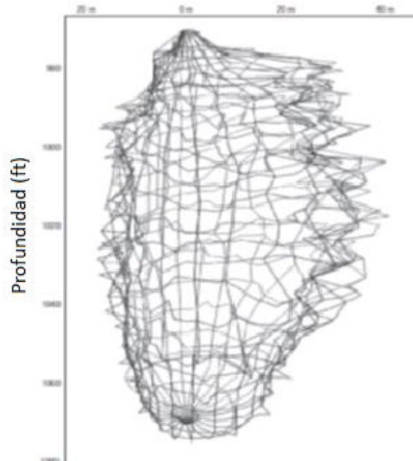
Fig. 4.16 Forma de una caverna delineada por las mediciones de un calibrador tipo sonar (Schlumberger 2003).
