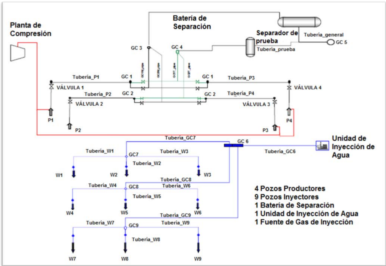
Figura III-4 Red de tuberías superficiales integral aplicado en el modelo de simulación de flujo (VIP). 3
