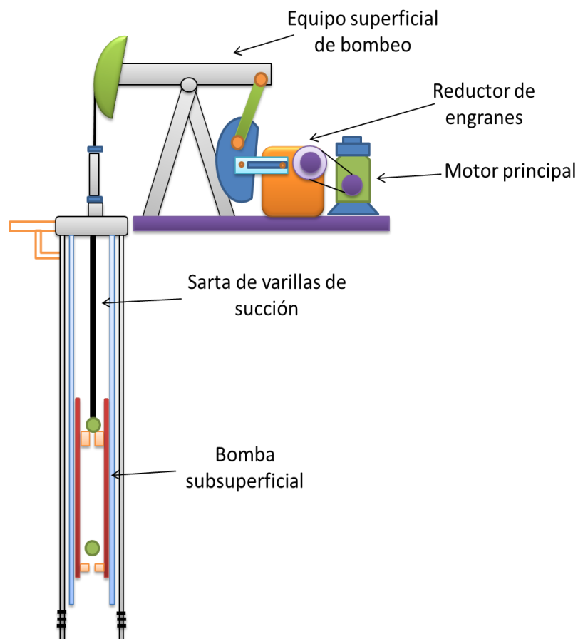
Fig. 1.3. Diagrama de un pozo con Bombeo mecánico. 5
