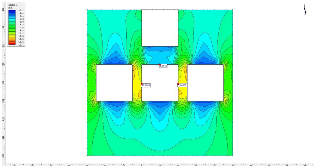
Figura 5.3 Estado de esfuerzos con un pilar de cabeza de 10m, en este caso los esfuerzos en los pilares son de 13.5 Mpa.
