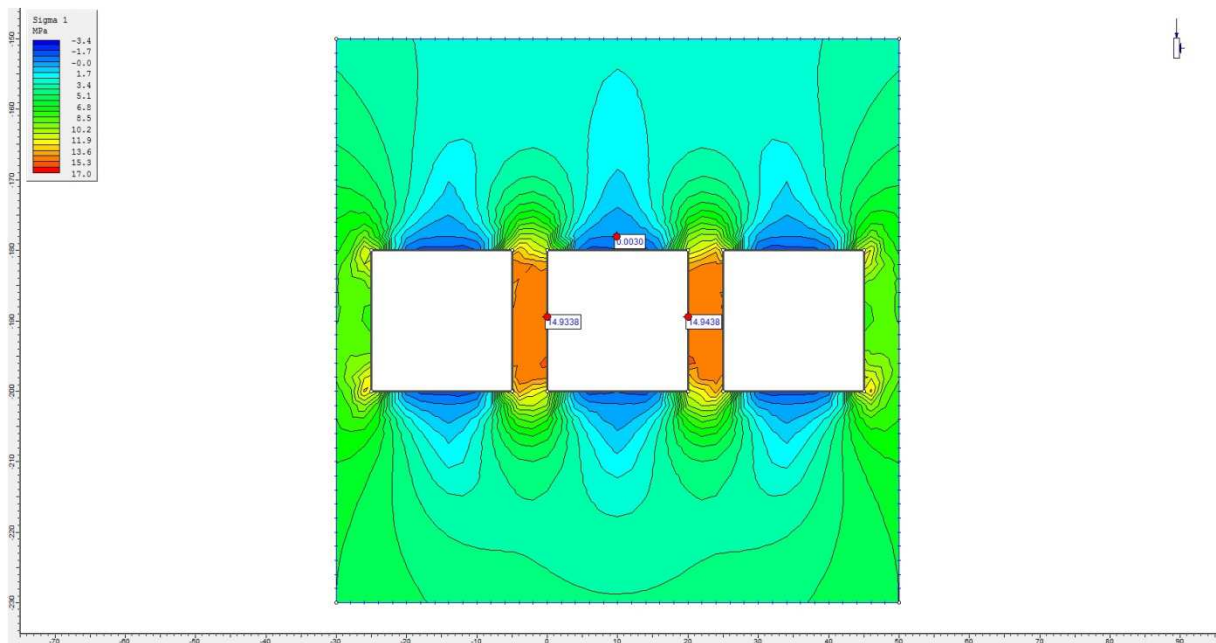
Figura 5.2 Estado de esfuerzos para un grupo de paneles con pilar intermedio de 5m.
