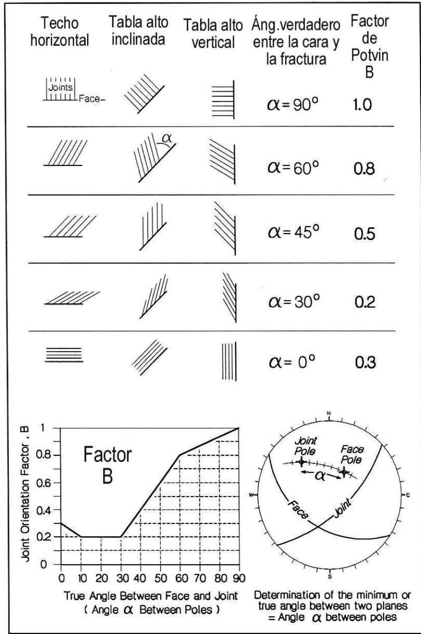
Figura 6.4 factor de ajuste B del método de Mathews.
