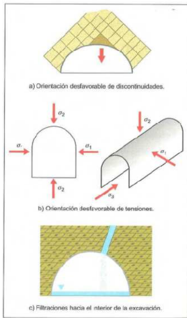
Figura 5.5 Condiciones naturales de inestabilidad en excavaciones de túneles en roca.
