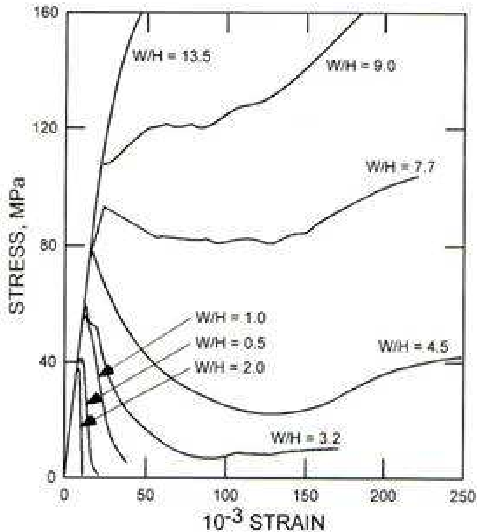
Figura 6.11 Grafica de relación de esfuerzo entre resistencia para varias relaciones de esbeltez.
