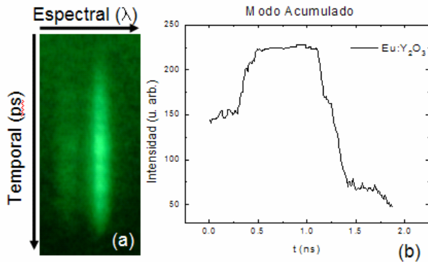
Figura 3 10 (a) Fotografía de un tren de pulsos tomada de la emisión de una muestra de \text{Eu:Y}_2\text{O}_3 con una cámara ultrarrápida y (b) Perfil de desintometría de este tren de pulsos
