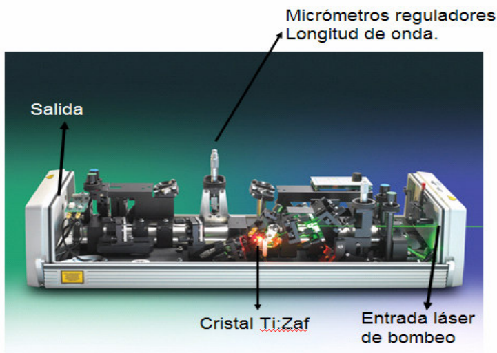
Figura 2 5 Vista interna del láser de Titanio Zafiro
