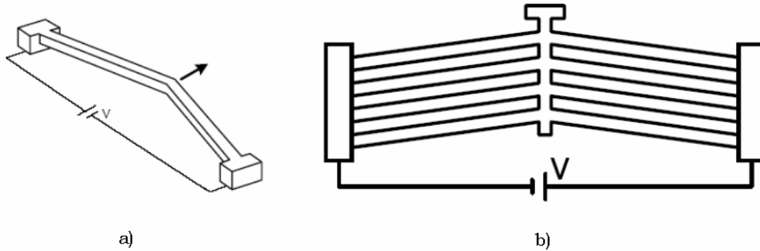
Fig. 4.10 Actuador electro-térmico tipo Chevrón . a) configuración básica, b) arreglo de actuadores.
