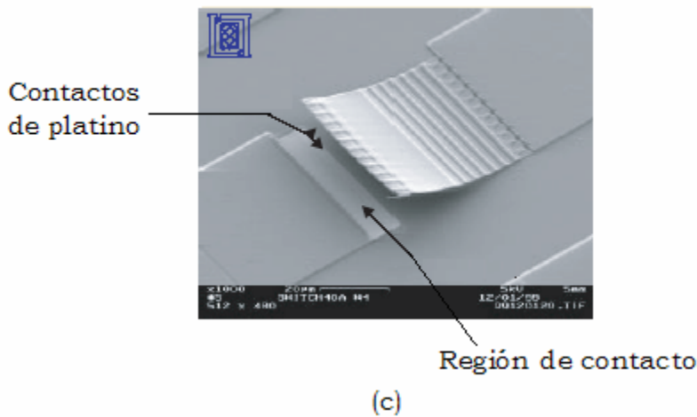
Fig. 2.36 Interruptor serie en línea de los laboratorios Lincoln: a) contacto metal-metal, b) contacto capacitivo y c) Micrografía de escaneo electrónico del interruptor [11].
