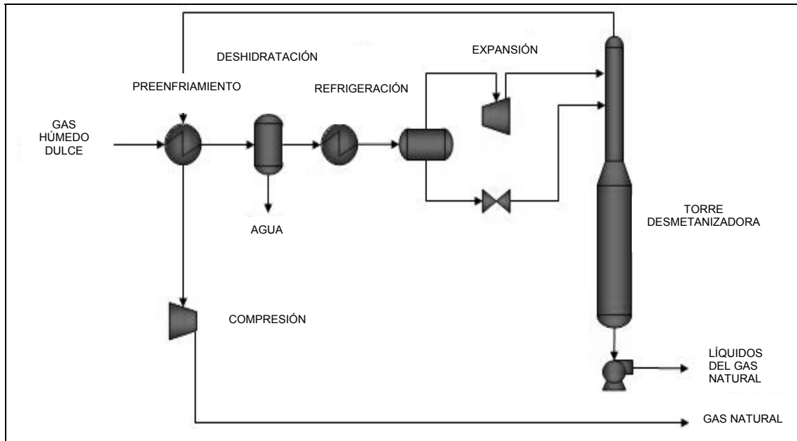
Figura 1.2 Proceso de separación criogénico
