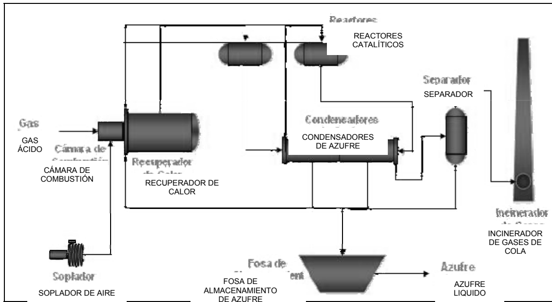
Figura 1.1 Recuperación de azufre elemental “Proceso Claus”
