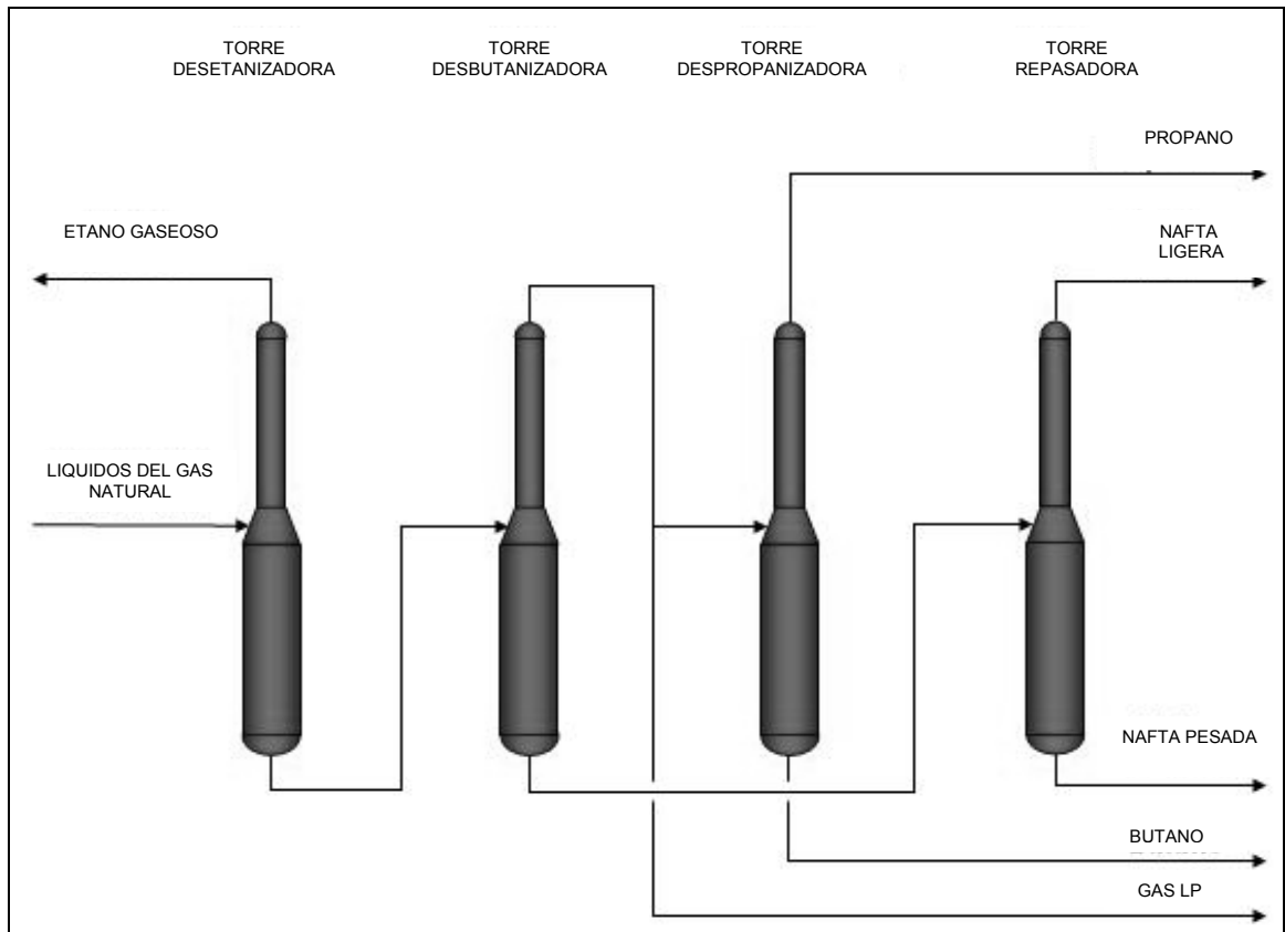
Figura 1.3 Fraccionamiento de líquidos del gas natural
