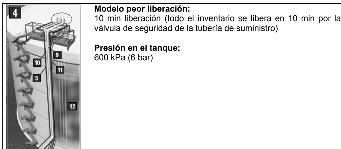
Figura 5.8 Instalación de válvulas de seguridad en la entrada a un tanque de GNL
