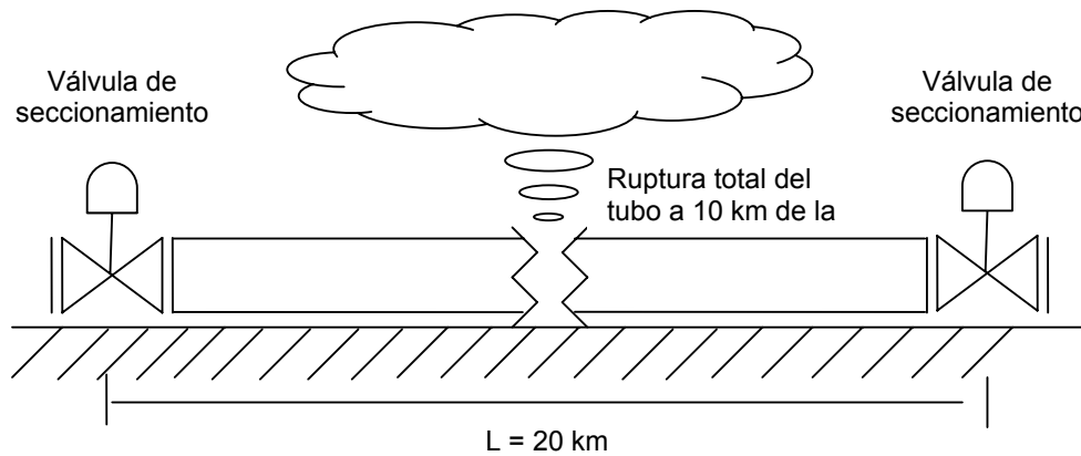
Figura 5.39 Escenario de ruptura total del gasoducto
