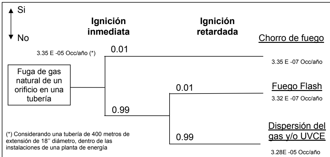
Figura 5.31 Árbol de análisis de eventos en una fuga de una tubería
