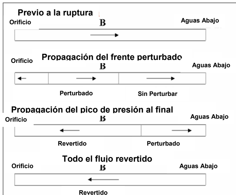
Figura 4.3 Modelo de ruptura del tubo en la parte baja
