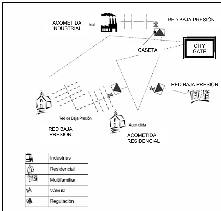
Figura 2.3 Esquema de red de distribución de gas natural
