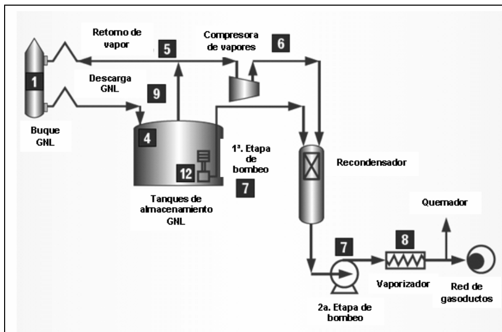
Figura 5.2 Esquema típico de una Terminal de Regasificación de GNL
