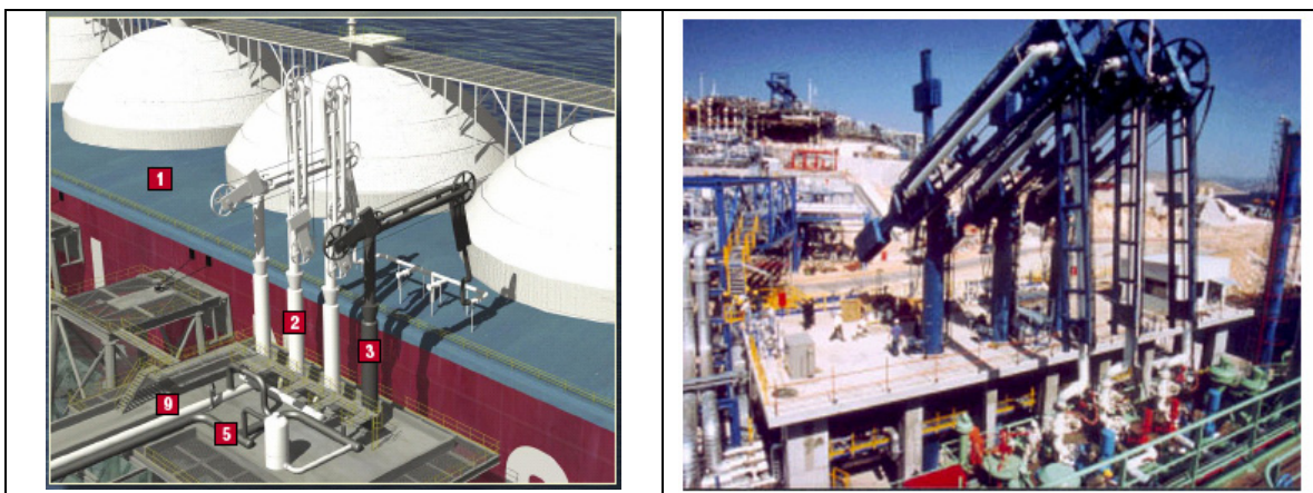
Figura 5.14 Esquema típico de los brazos de descarga (jetty)
