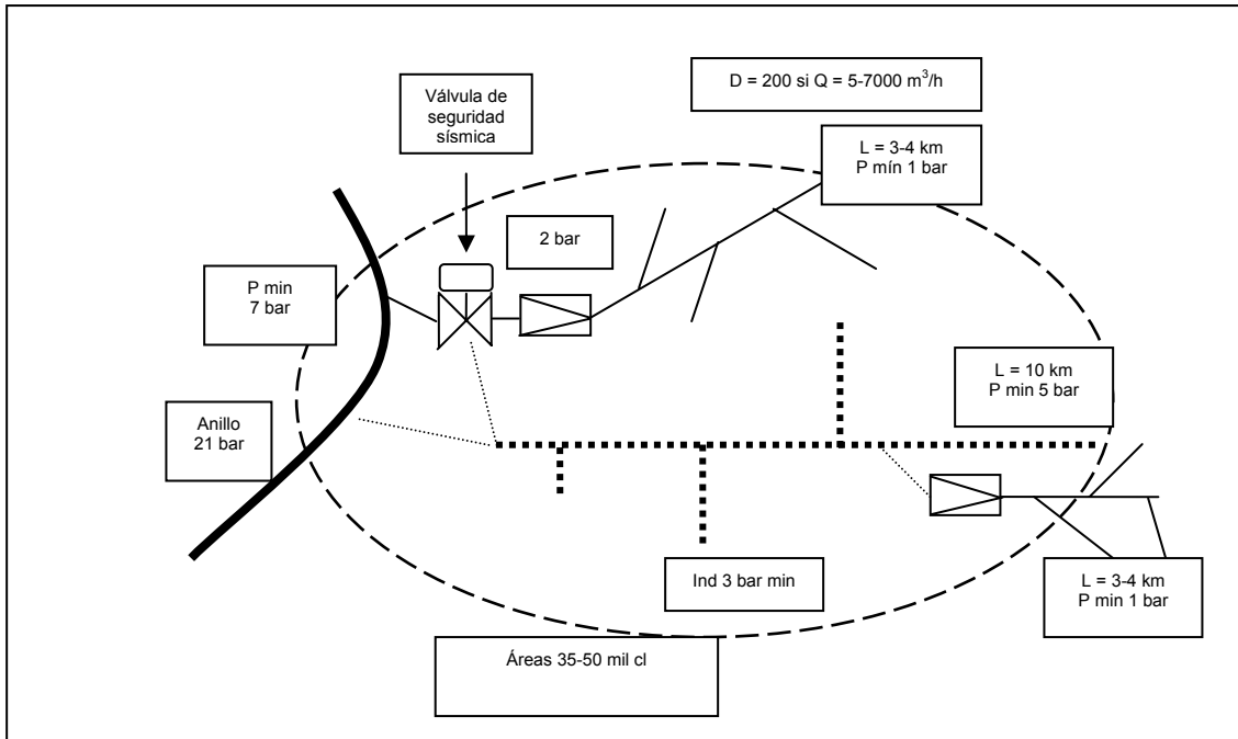
Figura 2.7 Diseño sistema Margarita
