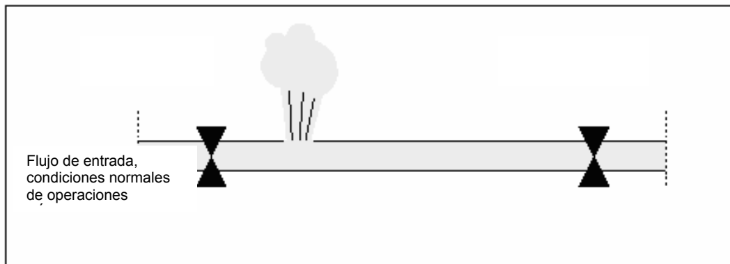
Figura 4.1 Esquema del modelo GASPIPE
