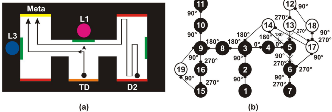
Figura V.16. (a) Rutas seguidas por el robot durante las pruebas iniciadas en las localidades TD y D2, donde el landmark L2 fue removido. (b) El mapa construido por el robot durante el experimento. Los nodos negros fueron creados durante el entrenamiento, y los blancos en las pruebas. Los arcos marcados con "X" fueron eliminados durante las pruebas.
