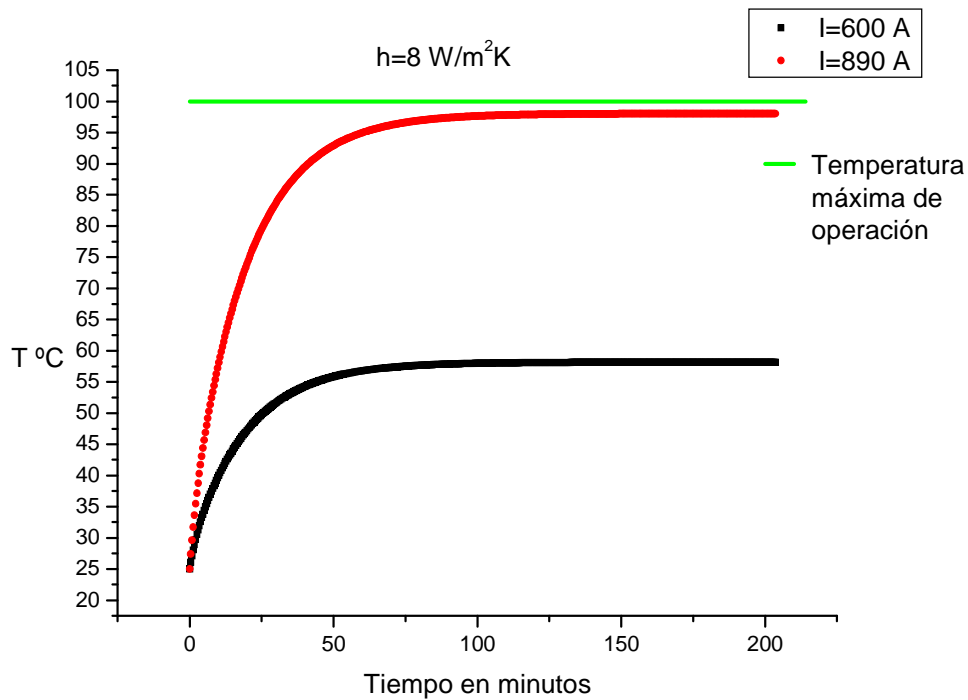
Figura 2. Comportamiento de la temperatura exterior de un cable ACSR DRAKE para distintas corrientes eléctricas.
