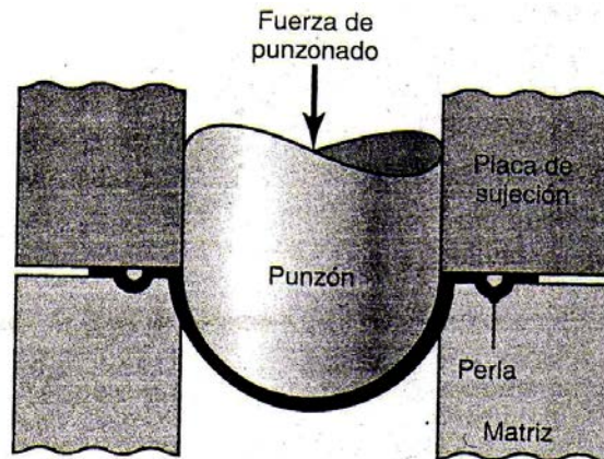
Figura 1.52 Prueba Erichsen (formado de depresión) lx .
