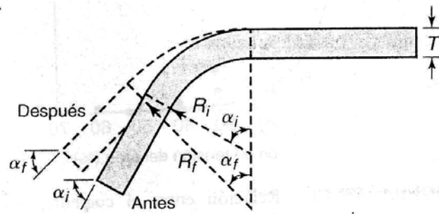
Figura 1.35. Recuperación elástica en el doblado xxvi .
