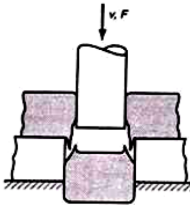
Figura 1.31 Un claro demasiado grande produce un corte menos limpio, originando rebabas más grandes xxx .
