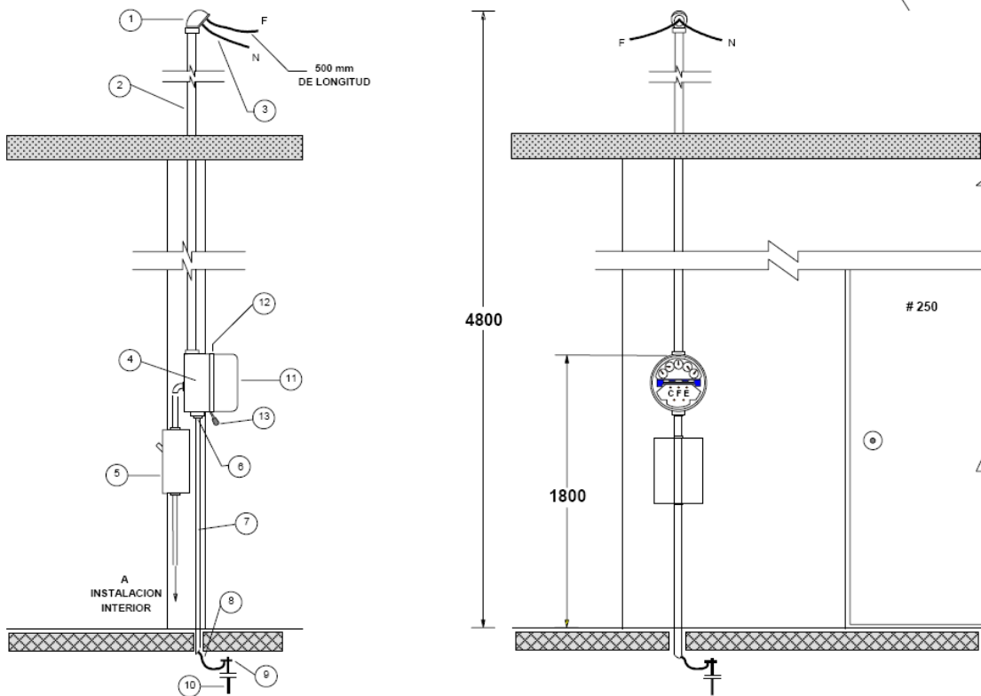
VISTA DE CONJUNTO
