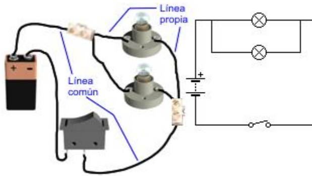
Figura 2.6 Circuito en paralelo
