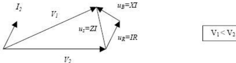
Figura 2.10 Diagrama de tensiones de un circuito capacitivo resistivo
