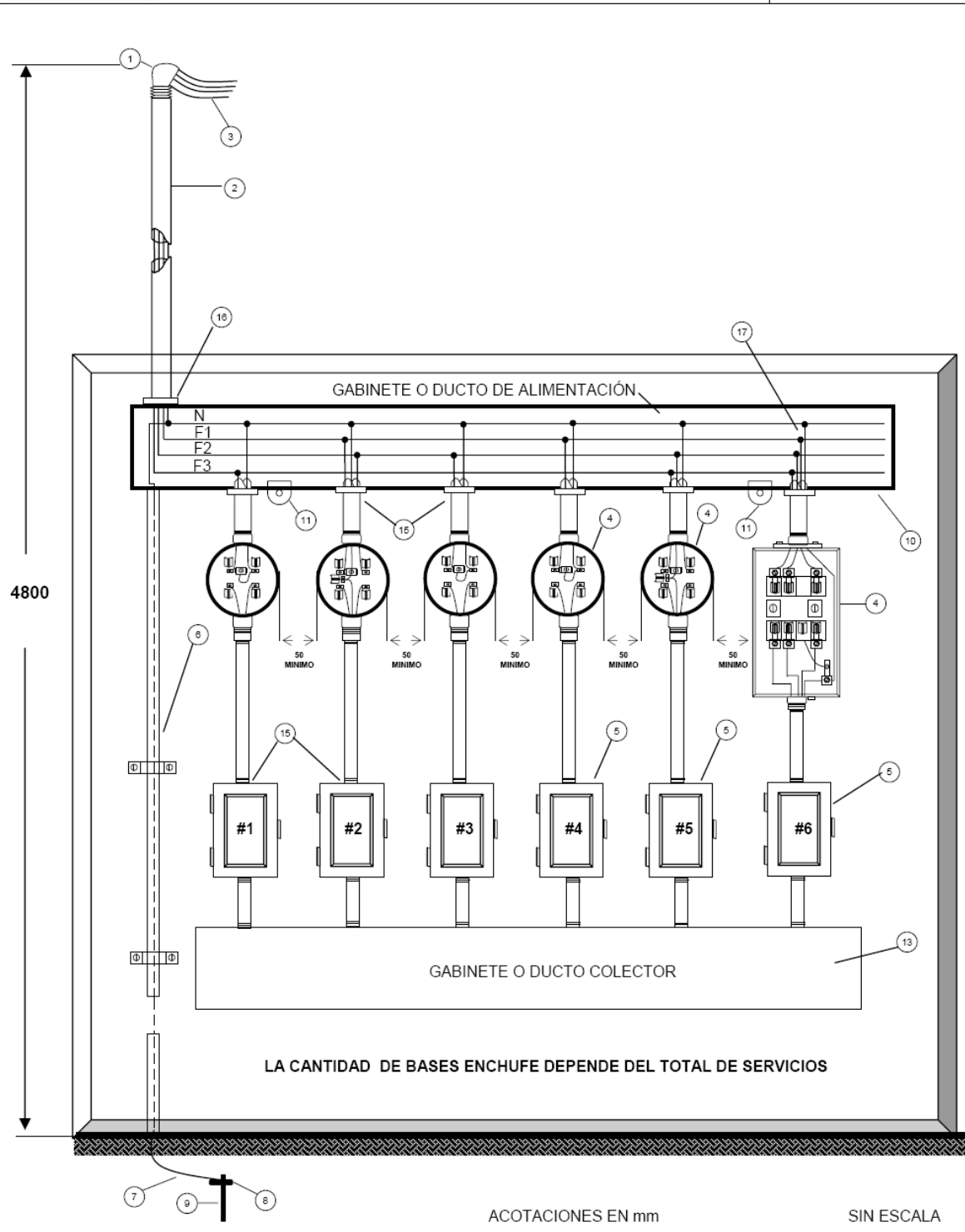
Figura 2.3.- Especificación para servicio monofásico plaza comercial. Exterior.
