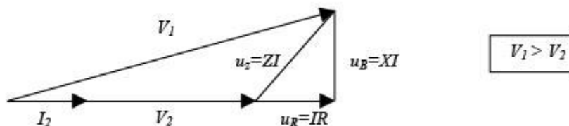
Figura. 2.8 Diagrama de tensiones de un circuito resistivo
