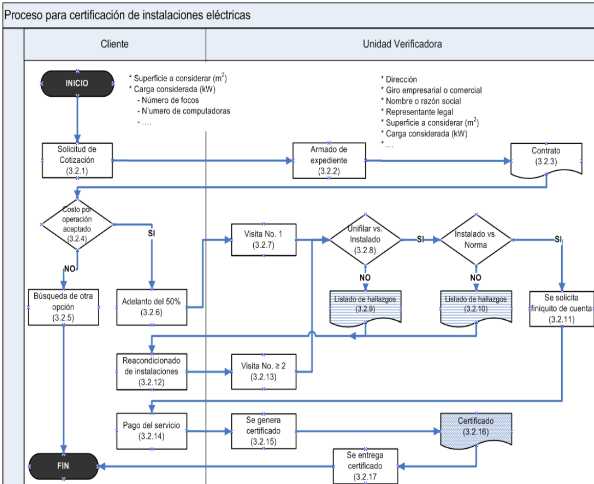
Figura 3.1 Proceso para certificación de instalaciones eléctricas.
