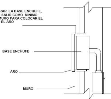
DETALLE DE EMPOTRADO DE LA BASE
