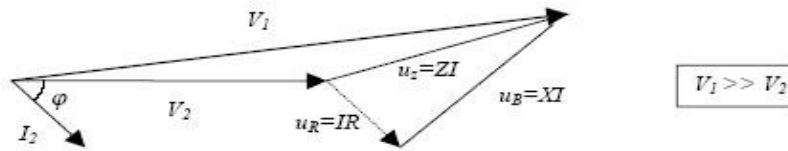
Figura. 2.9 Diagrama de tensiones de un circuito inductivo resistivo
