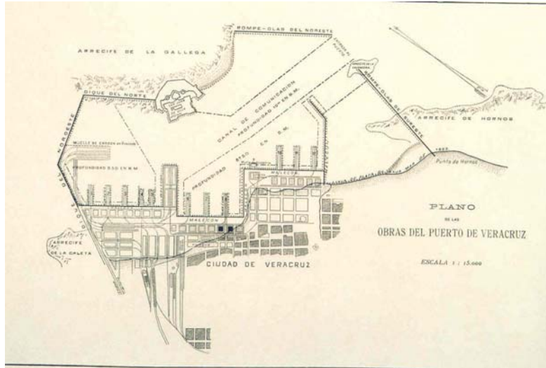
Figura 2.2 Plano de las obras del Puerto de Veracruz
