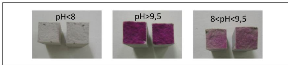
Figura 3.8. Tonalidades de la fenolftaleína en el concreto [23] .
