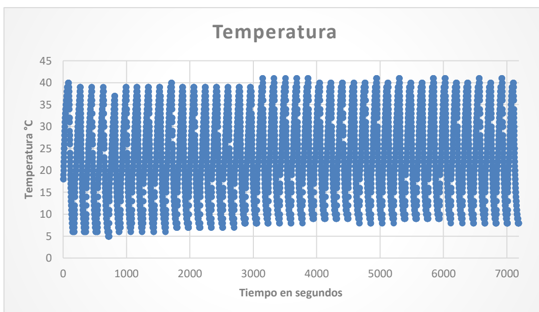
Grafica 3.1. Comportamiento de la temperatura durante los ensayos acelerados de Nitración.
