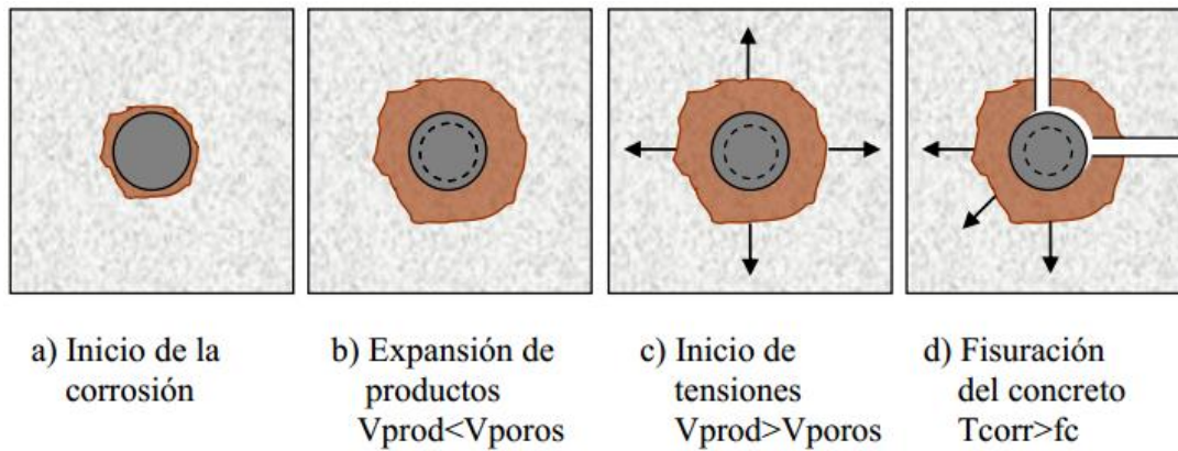
Figura 1.4. Proceso de fisuración del concreto. [25]
