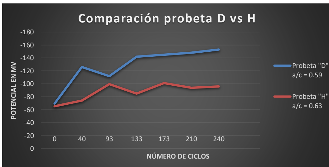
Gráfica 4.4. Probetas sometidas a humedad, temperatura y gases con diferentes relaciones a/c.
