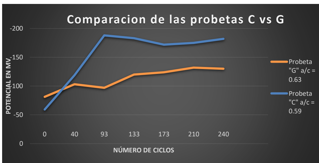
Gráfica 4.3. Comparativo de probetas con diferente relación a/c, sometidas a humedad temperatura y gases.
