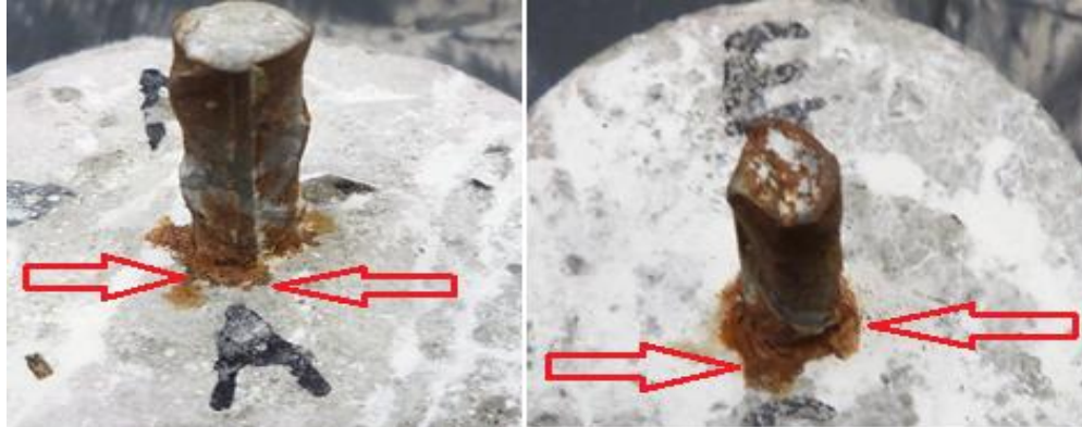
Figura 4.4. Comparación de la formación de productos de corrosión (herrumbre) entre probetas con diferente relación a/c (“A” =0.59 y “E” =0.63), expuestas en solución salina al 3.5%.
