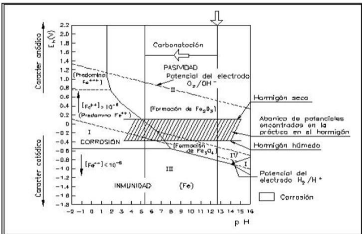
Figura 1.2. Diagrama de Pourbaix hierro-agua y condiciones reales del acero embebido en concreto. [26]
