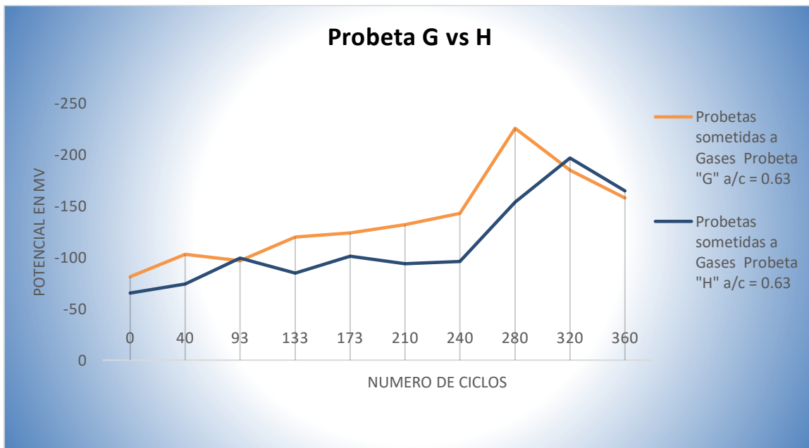
Grafica 4.6. Comparación de potenciales después de ser humectadas las probetas.
