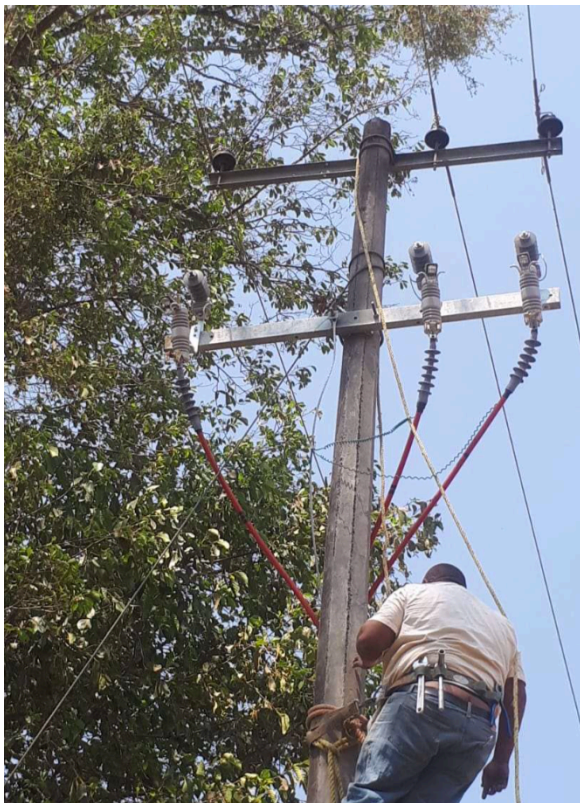
Imagen C. 47. Colocación de los accesorios para la vestimenta del poste. Aquí se hizo la conexión a la línea de distribución.
