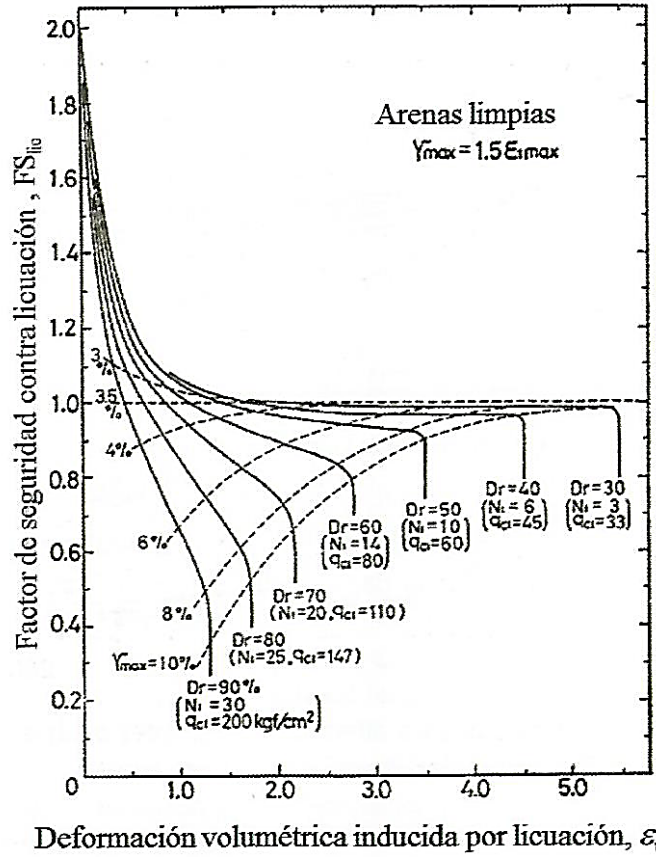
Figura 3.8. Deformación volumétrica en función del factor de seguridad (Ishihara y Yoshimine, 1992).
