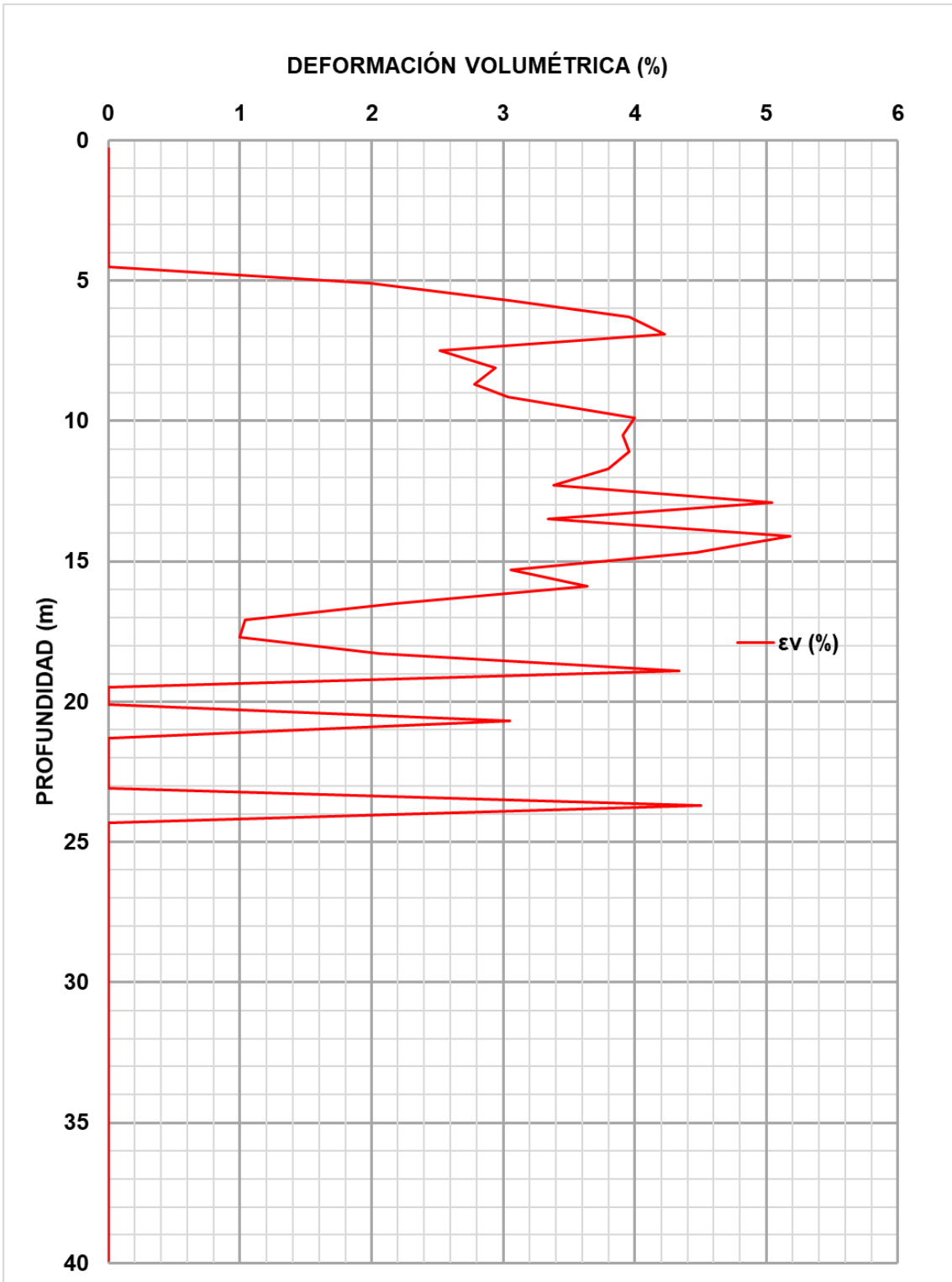
Figura 5.26. Asentamientos.
