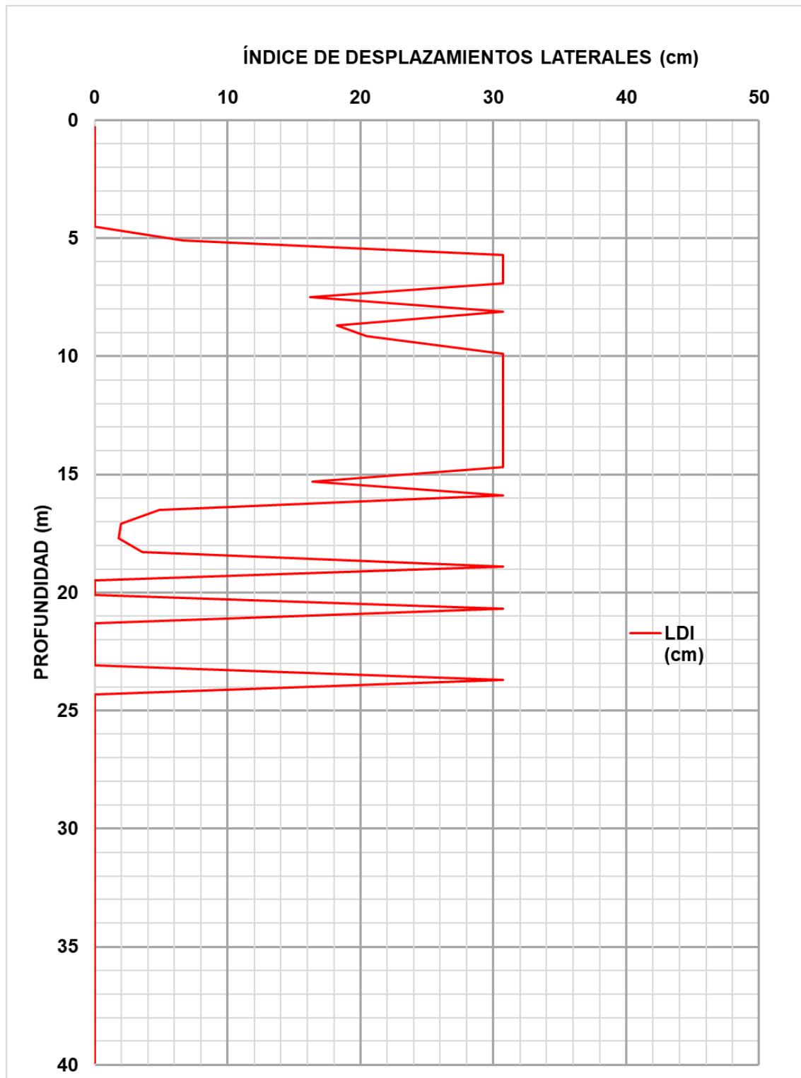
Figura 5.22. Índice de desplazamientos laterales.
