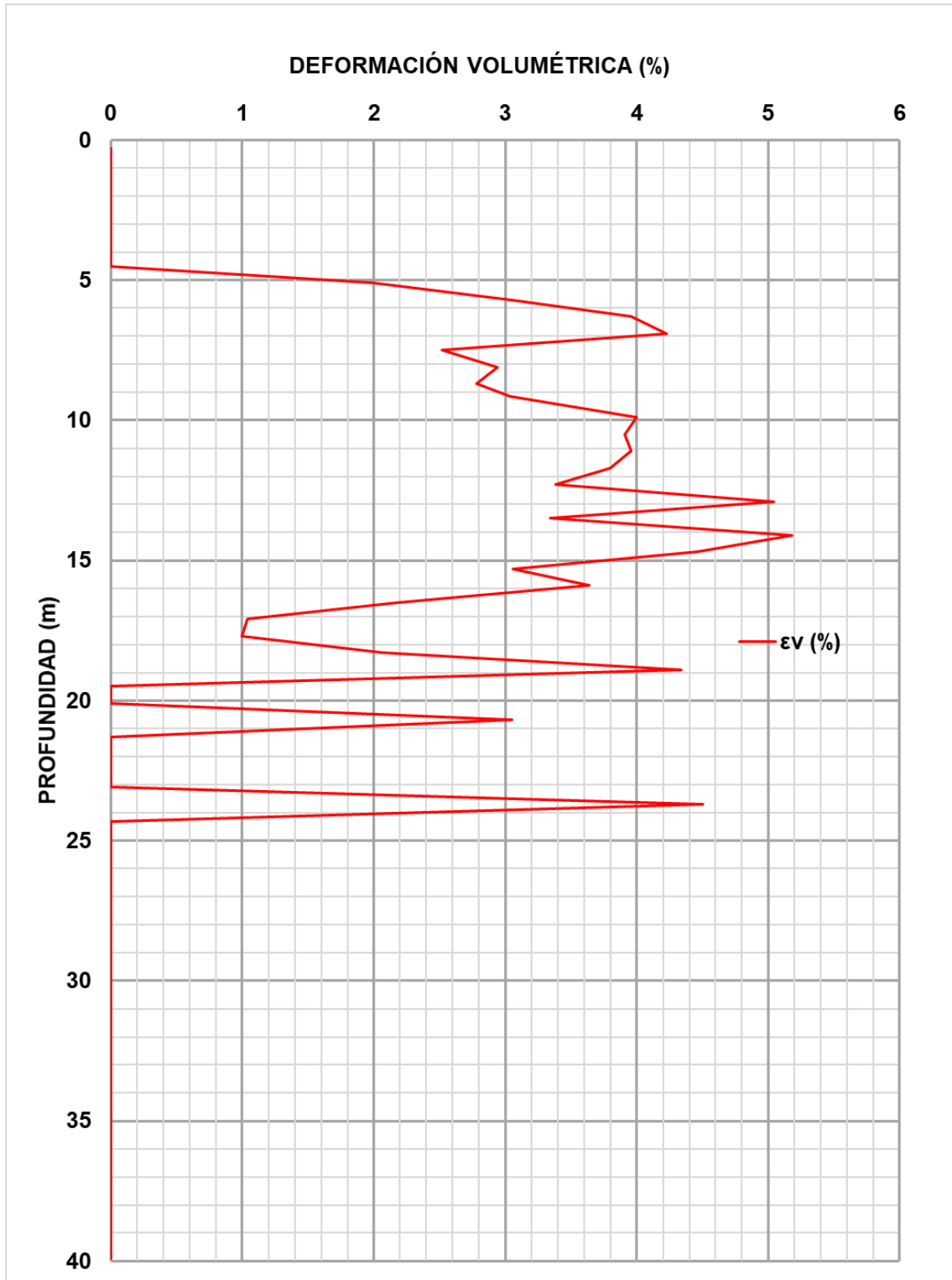
Figura 5.25. Deformación volumétrica.
