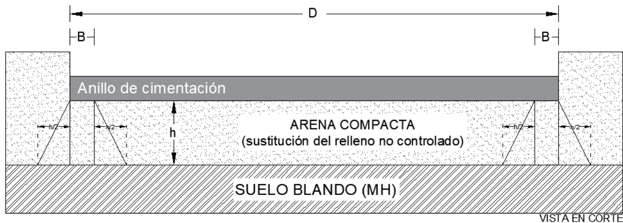
Figura 6.1 Desplante del anillo en estrato resistente y presencia de estrato débil por debajo, vista en corte.
