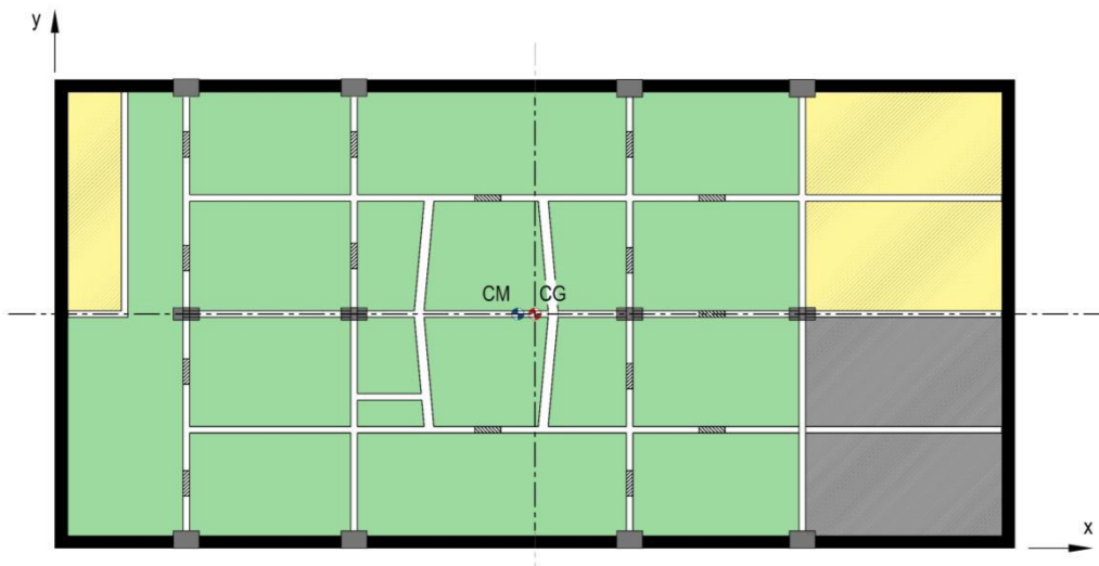
Figura 4.1 Ubicaciones del centro geométrico y de masa
