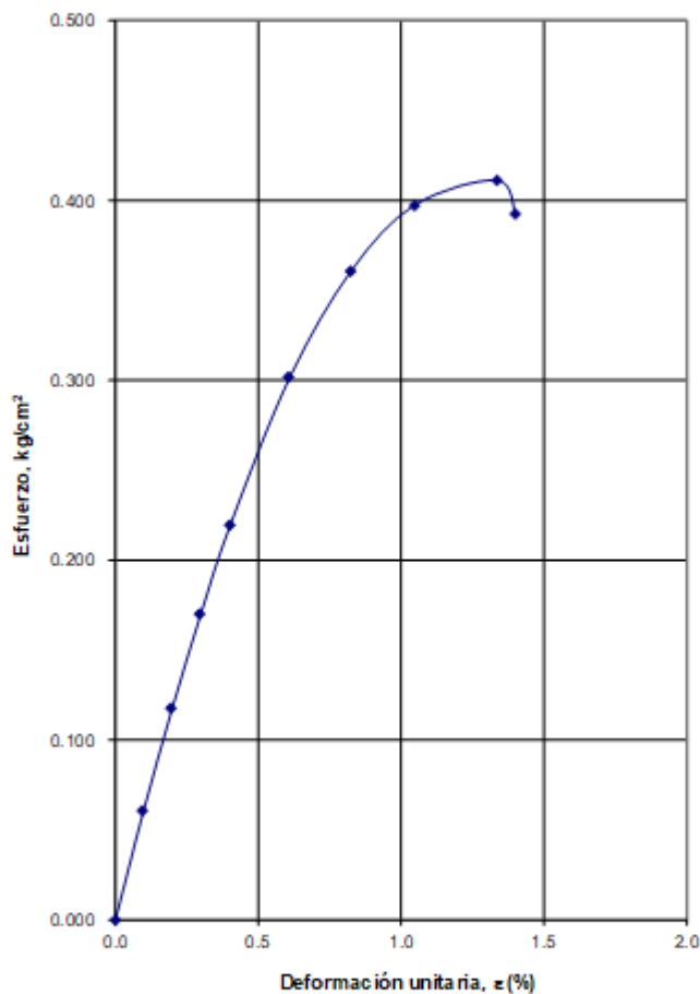
PRUEBA DE COMPRESIÓN SIMPLE q_u
