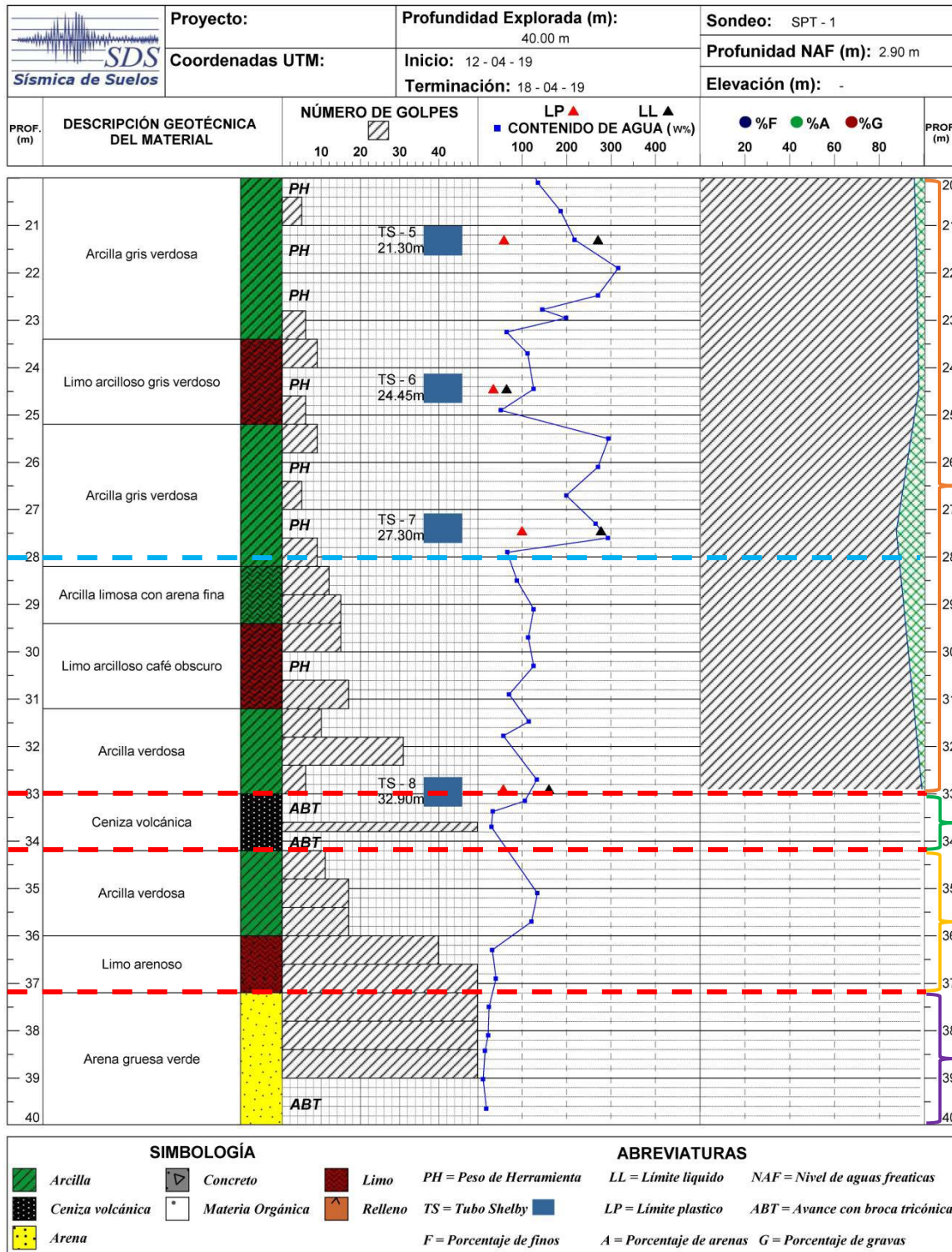
Figura 3.2. Perfil estratigráfico obtenido del SPT de 20 a 40 m
