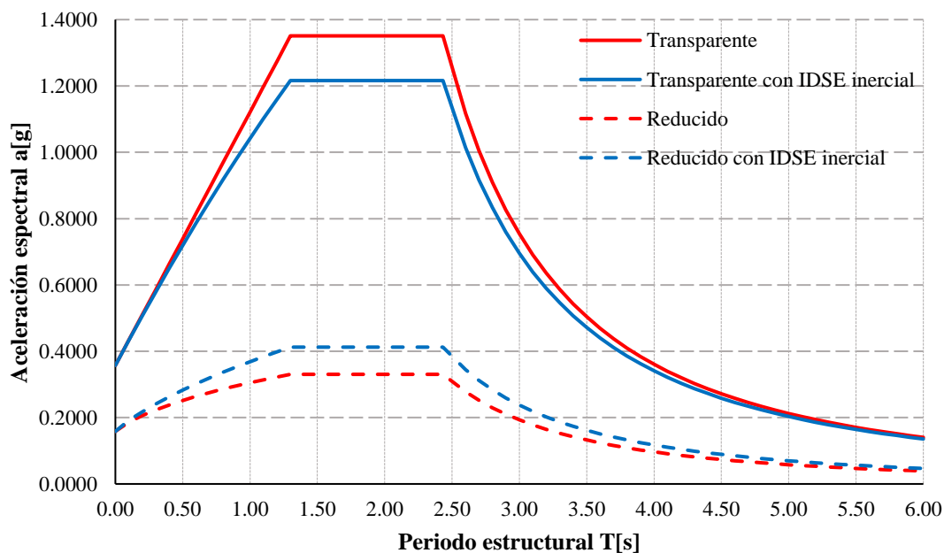
Figura 6.2 Espectros de diseño transparente y reducido de SASID y con IDSE inercial para la dirección de análisis x
