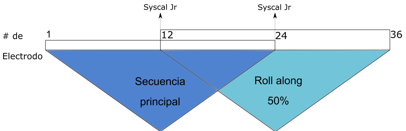
Figura 4.4: Roll along al 50 % empleado en la adquisición de los datos en los arreglos electrónicos Dipolo-Dipolo y Wenner-Schlumberger
