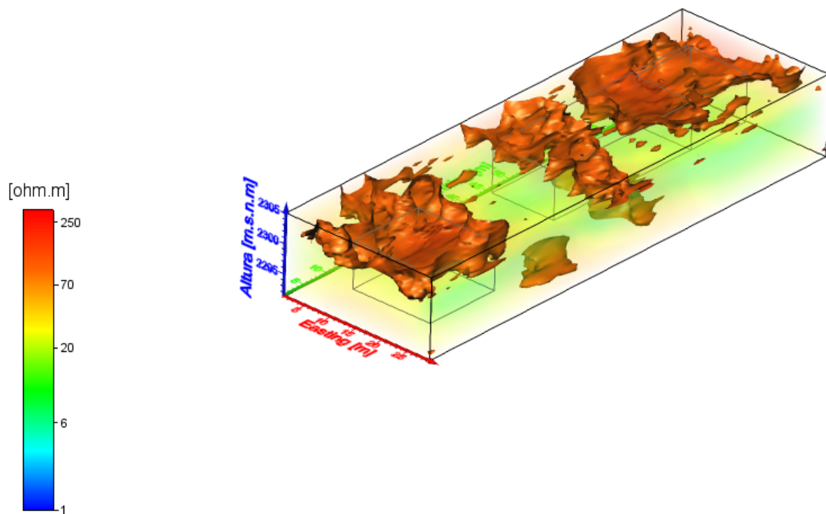
Figura 5.14: Inversión 3D, Arreglo electrónico Wenner-Schlumberger. Vista oblicua. Ver video (Es necesario contar con internet)
