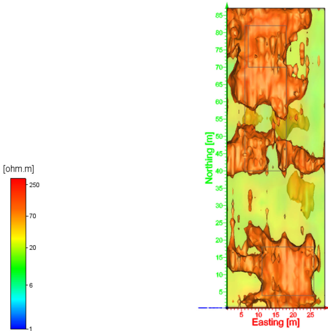
Figura 5.15: Inversión 3D, Arreglo eléctrico Wenner-Schlumberger. Vista en planta. Ver video (Es necesario contar con internet)
