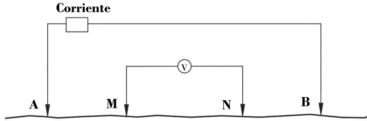
Figura 3.3: Arreglo electródico convencional con cuatro electrodos
