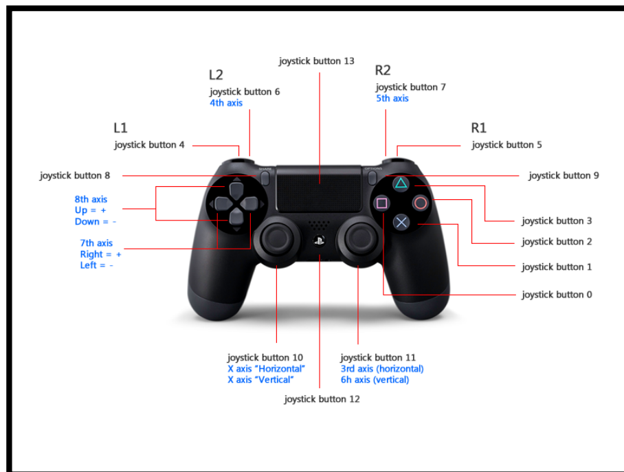
Imagen 5.98 Control de PlayStation 4 con la configuración de los botones.
