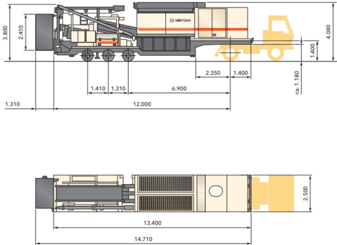
Ilustración 16 Dimensiones en metros de la KMA 220 en posición de ser transportada. Fuente Wirtgen maquinaria.
