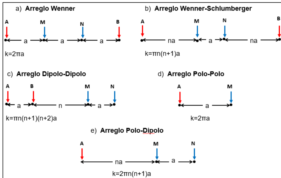
Figura 3 Esta figura muestra cuatro dispositivos electródicos más comunes con el respectivo factor geométrico (Modificado de Loke, 2004 y Milsom, 2003)
