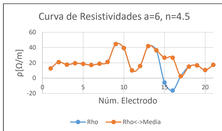
Figura 30. En azul la curva de resistividad para la Línea 1 con espaciamento entre electrodos AM = 6 y un nivel n=4.5, en naranja la curva de resistividad después de intercambiar los datos menores que cero por el valor de la media.
