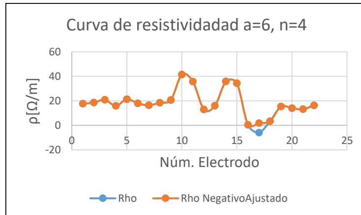
Figura 29. En azul la curva de resistividad para la Línea 1 con espaciamento entre electrodos AM = 6 y un nivel n=4; en naranja la curva de resistividad después de ajustar el dato menor que cero.
