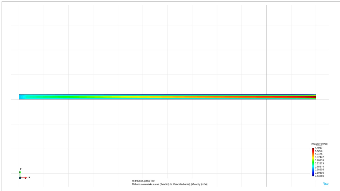
Figura 4.38c. Perfil N° 3 elaborado en IBER. Resultados correspondientes a la velocidad media presentada a lo largo del perfil, para el instante de 180 segundos en el intervalo de simulación del modelo.
