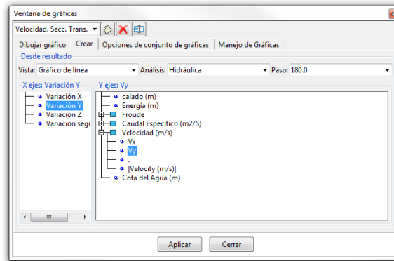
Figura 4.32a. Creación del set de gráficas para obtener la distribución de velocidad en diferentes secciones transversales del modelo.
