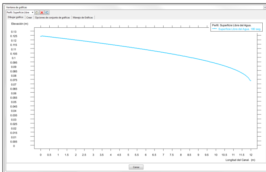
Figura 4.14a. Perfil de la superficie libre del agua. Perfil N° 1.
