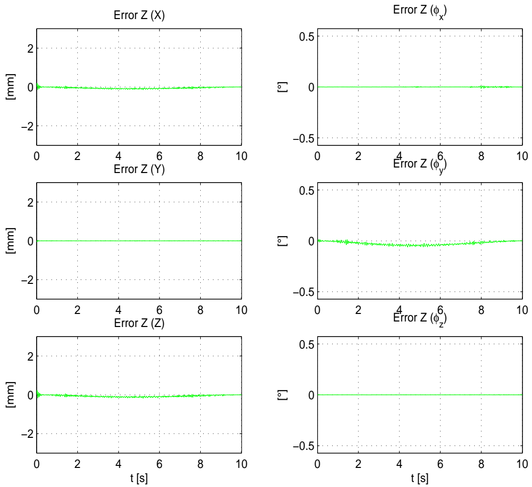
Figura 4.34: Experimento 3. Vector \mathbf{z} de error de observación ( \mathbf{x} - \hat{\mathbf{x}} ).
