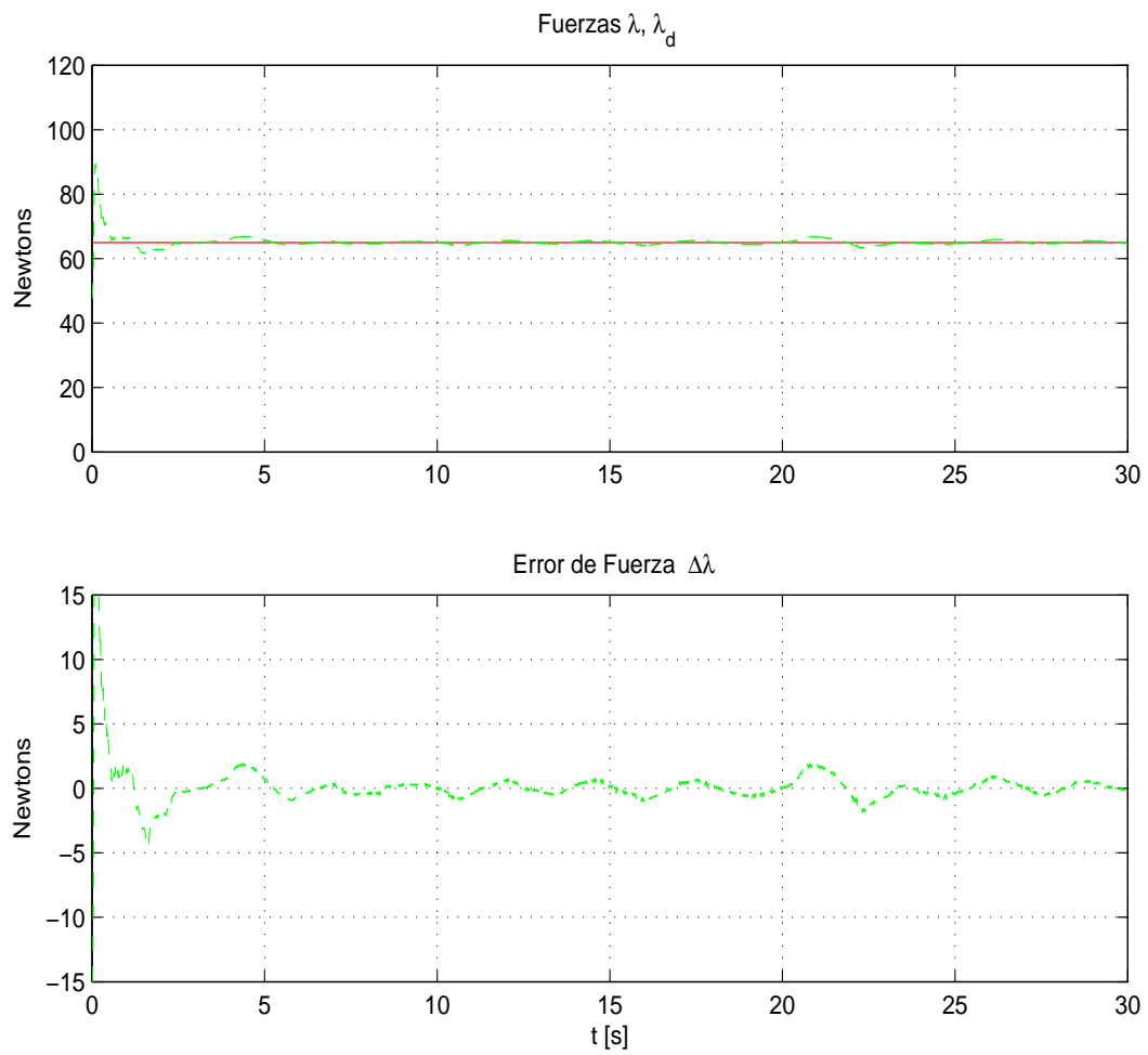
Figura 4.41: Experimento 4. Fuerza deseada \lambda_d (—) vs fuerza real \lambda (- -) y su correspondiente error de seguimiento ( \lambda - \lambda_d ).
