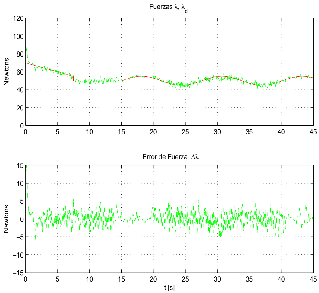
Figura 4.6: Experimento 1. Fuerza deseada \lambda_d (—) vs fuerza real \lambda (- -) y su correspondiente error de seguimiento ( \lambda - \lambda_d ).
