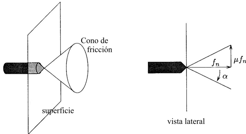
Figura 2.5: Interpretación geométrica del Modelo de fricción de Coulomb
