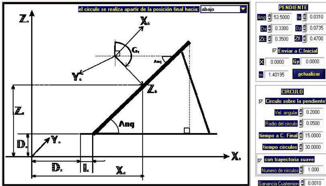
Figura B.7: Diagrama para superficie plana con parámetros
