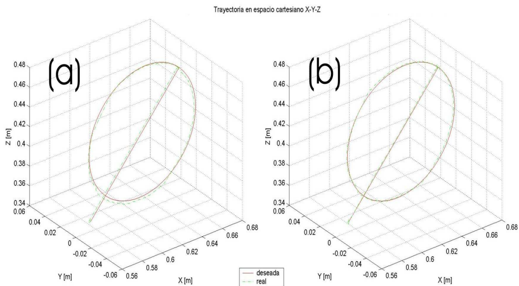
Figura 4.1: Gráficas de posición X-Z de trayectoria deseada vs real, (a) Con mediciones físicas, (b) Con mediciones calibradas.
