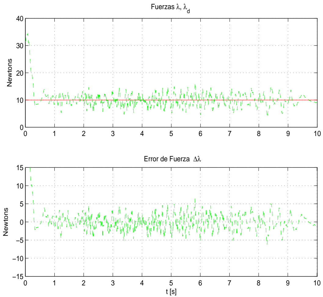
Figura 4.36: Experimento 3. Fuerza deseada \lambda_d (—) vs fuerza real \lambda (- -) y su correspondiente error de seguimiento ( \lambda - \lambda_d ).
