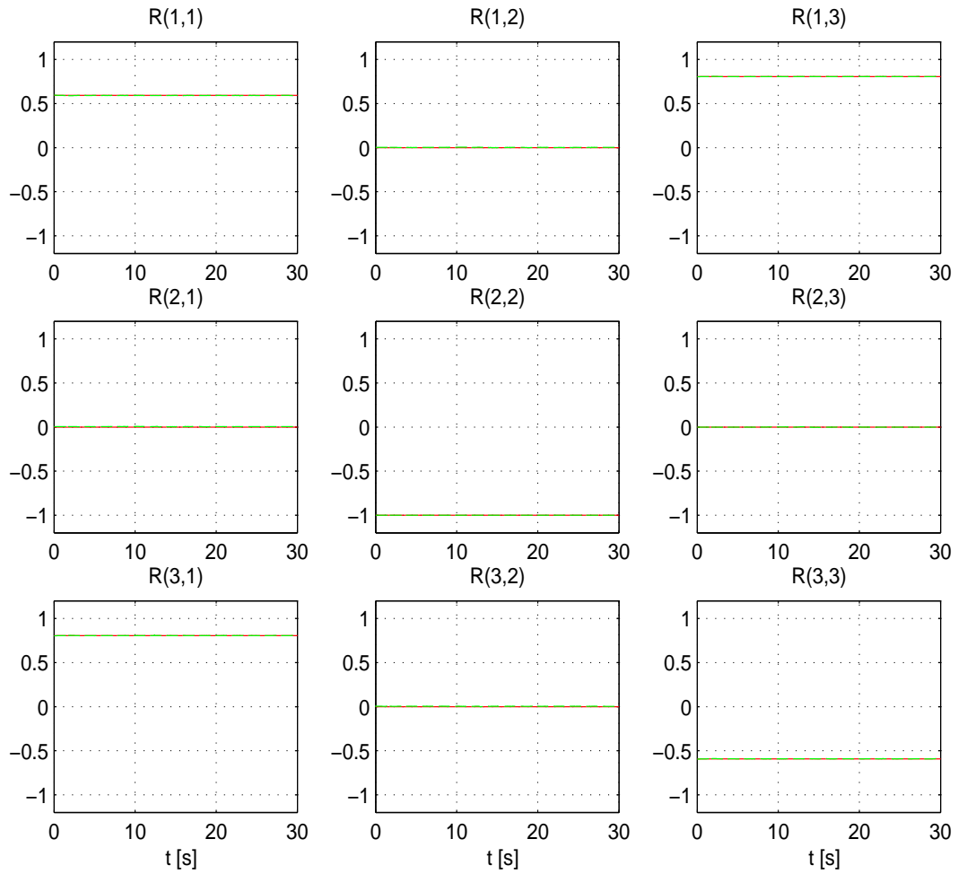
Figura 4.15: Experimento 3. Orientación deseada {}^0\mathbf{R}_d (—) vs orientación real {}^0\mathbf{R}_n (- -).
