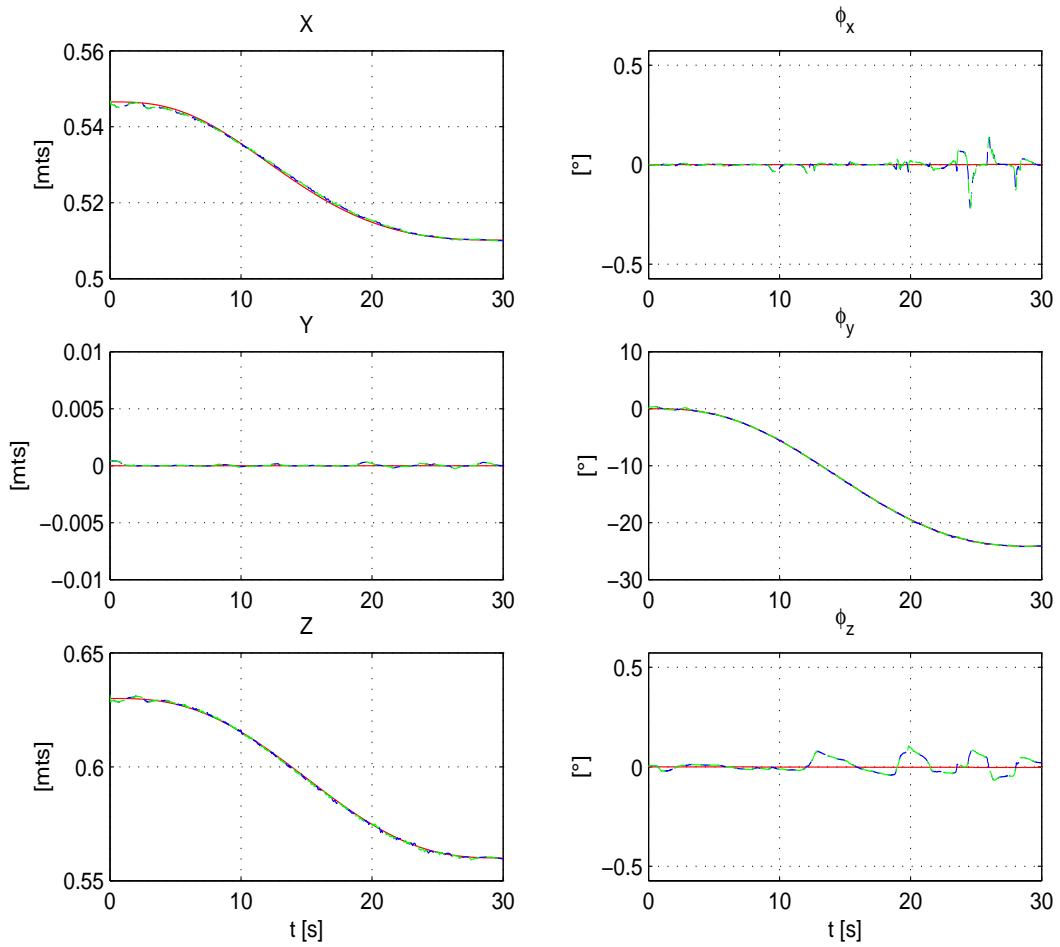
Figura 4.27: Experimento 2. Trayectoria deseada (—) vs trayectoria real (- -) vs trayectoria observada (- · -), de \mathbf{x}=[x \ y \ z \ \phi_x \ \phi_y \ \phi_z]^T .
