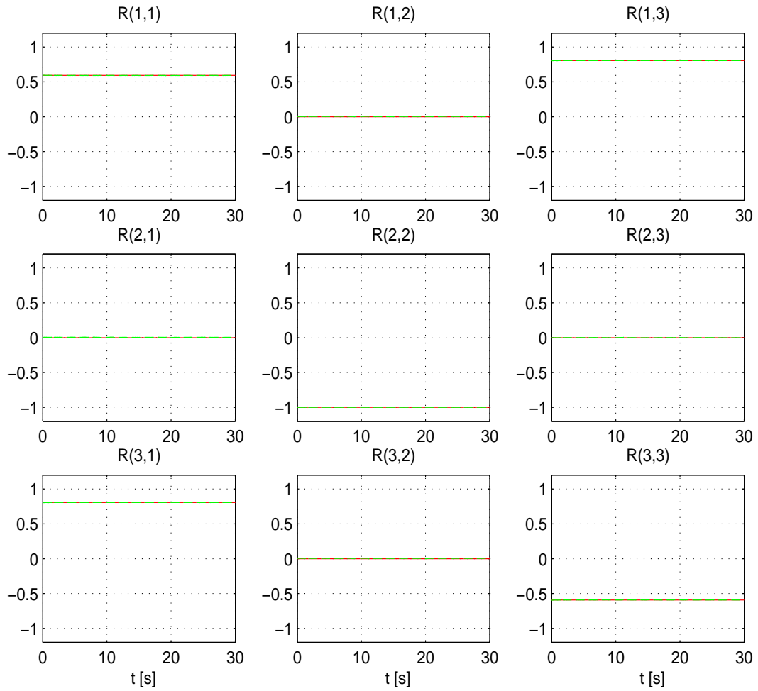
Figura 4.20: Experimento 4. Orientación deseada {}^0\mathbf{R}_d (—) vs orientación real {}^0\mathbf{R}_n (- -).
