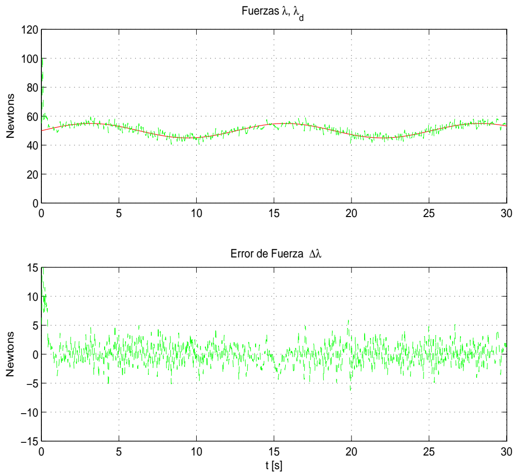
Figura 4.21: Experimento 4. Fuerza deseada \lambda_d (—) vs fuerza real \lambda (- -) y su correspondiente error de seguimiento ( \lambda - \lambda_d ).
