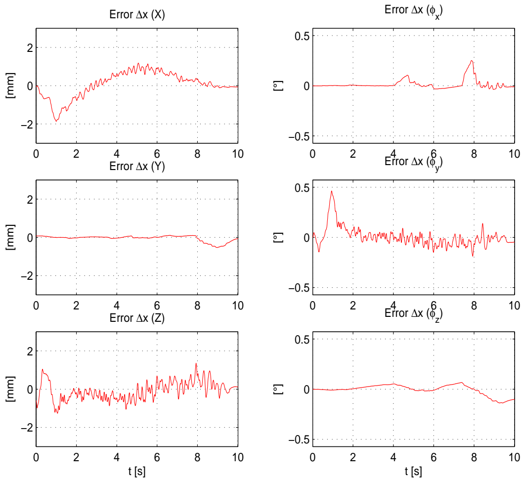
Figura 4.33: Experimento 3. Vector \Delta \mathbf{x} de error de seguimiento ( \mathbf{x} - \mathbf{x}_a ).
