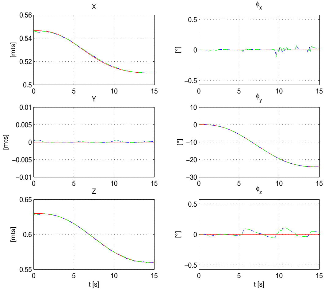
Figura 4.22: Experimento 1. Trayectoria deseada (—) vs trayectoria real (- -) vs trayectoria observada (- · -), de \mathbf{x}=[x \ y \ z \ \phi_x \ \phi_y \ \phi_z]^T .
