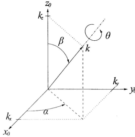
Figura 2.11: Rotación sobre un eje arbitrario
