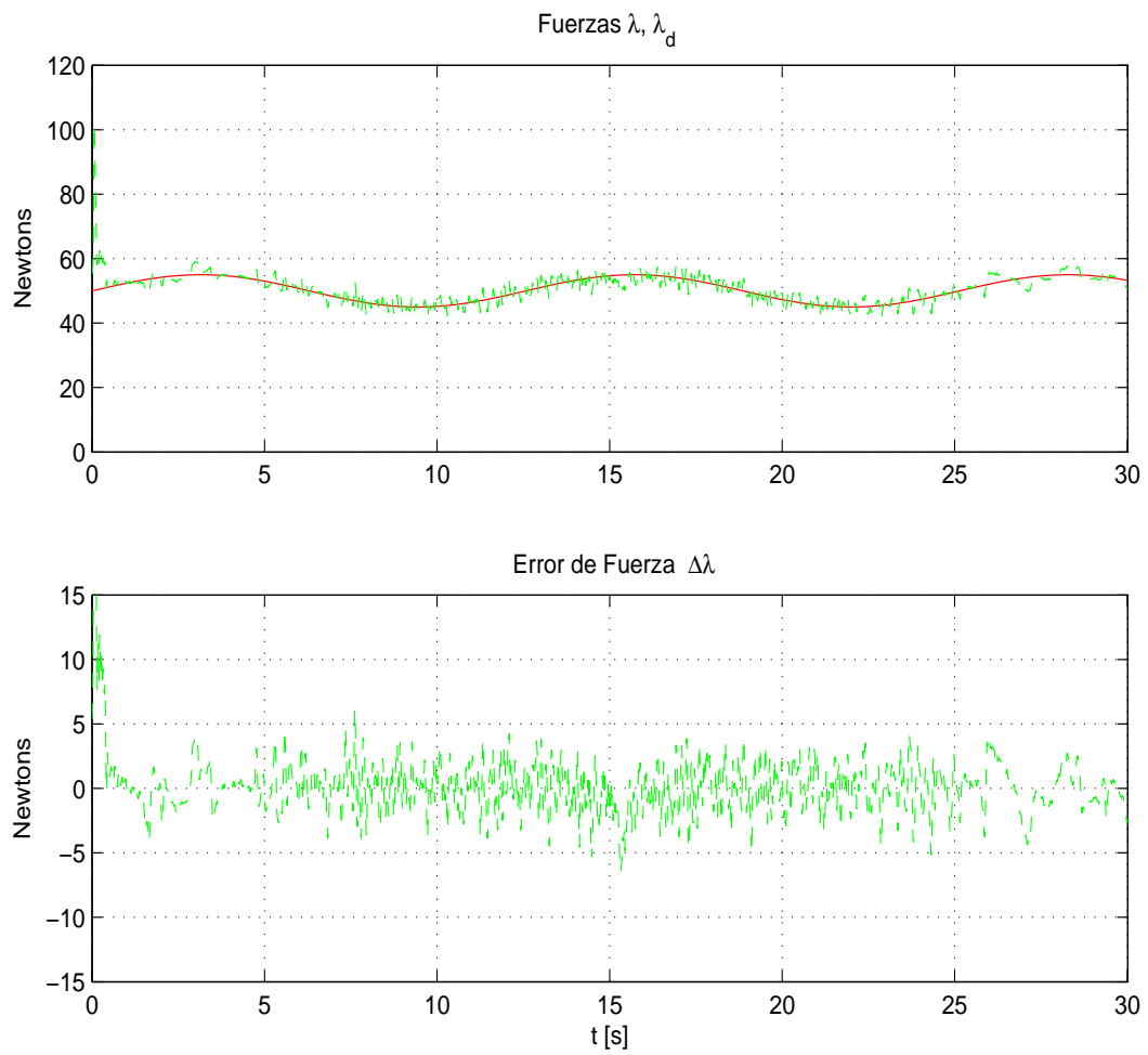
Figura 4.16: Experimento 3. Fuerza deseada \lambda_d (—) vs fuerza real \lambda (- -) y su correspondiente error de seguimiento ( \lambda - \lambda_d ).
