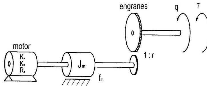
Figura 2.8: Diagrama de un motor de corriente directa.
