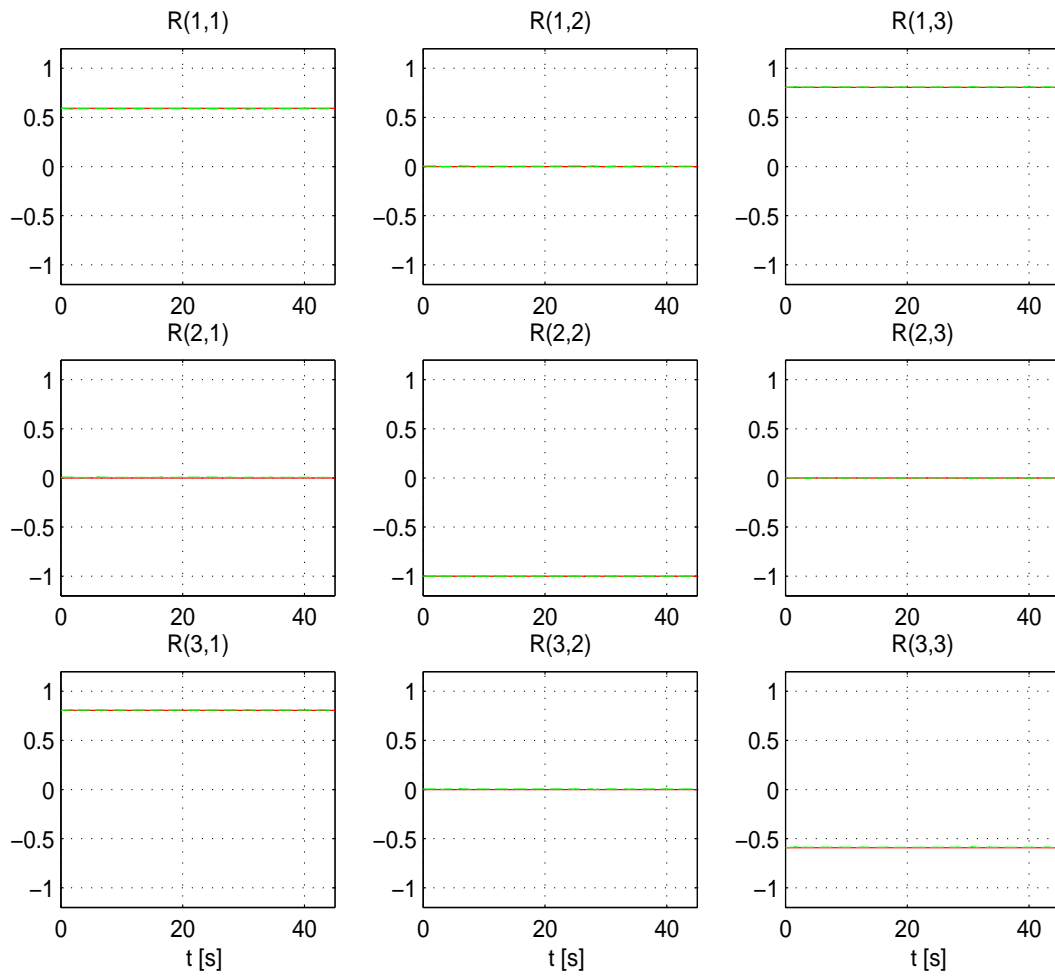
Figura 4.5: Experimento 1. Orientación deseada {}^0R_d (—) vs orientación real {}^0R_n (- -).
