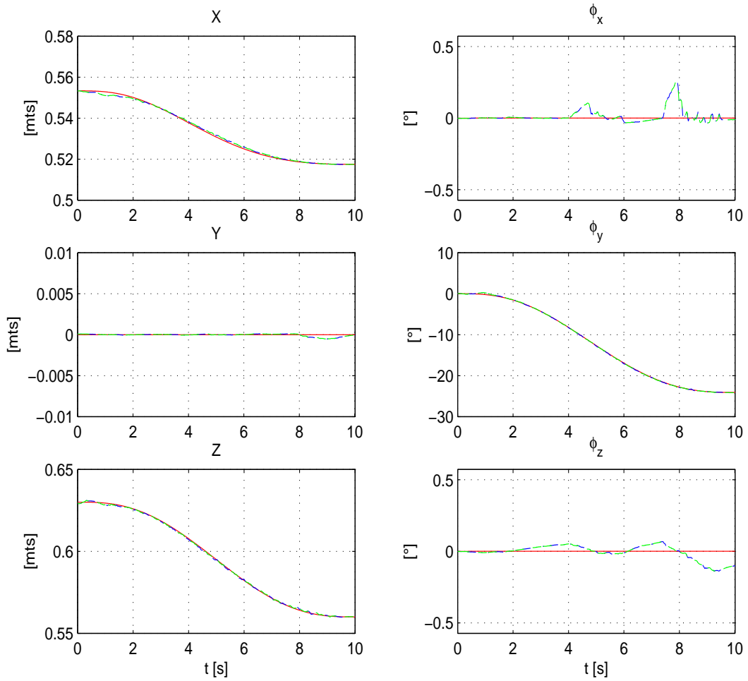
Figura 4.32: Experimento 3. Trayectoria deseada (—) vs trayectoria real (- -) vs trayectoria observada (- · -), de \mathbf{x}=[x \ y \ z \ \phi_x \ \phi_y \ \phi_z]^T .
