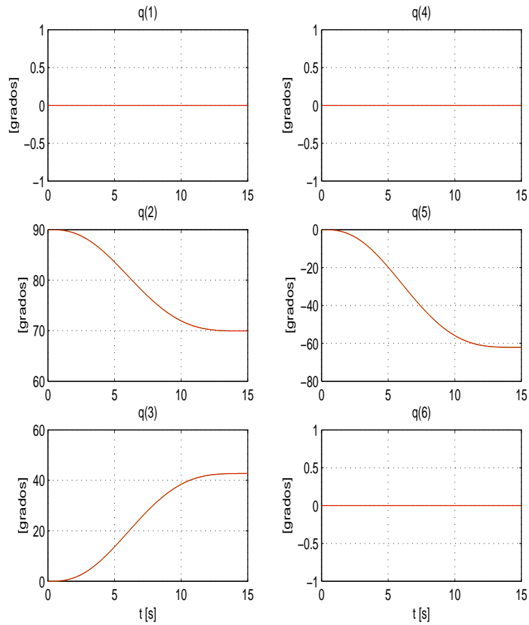
Figura B.2: Trayectoria creada por un polinomio de orden 6, para las articulaciones del Robot A465
