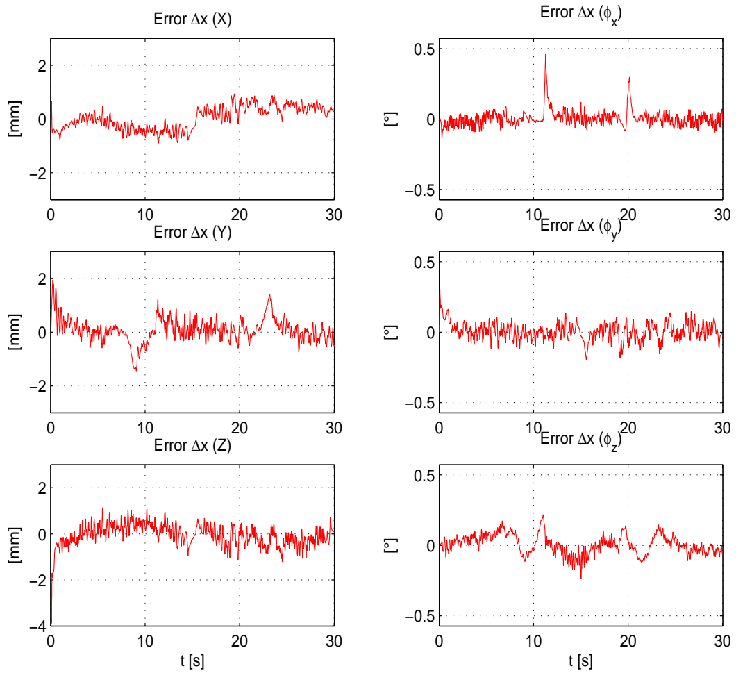
Figura 4.18: Experimento 4. Vector \Delta \mathbf{x} de error de seguimiento ( \mathbf{x} - \mathbf{x}_a ).
