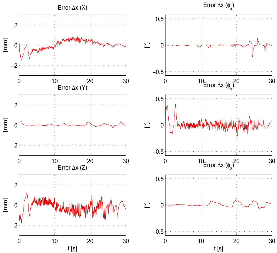
Figura 4.28: Experimento 2. Vector \Delta \mathbf{x} de error de seguimiento ( \mathbf{x} - \mathbf{x}_a ).
