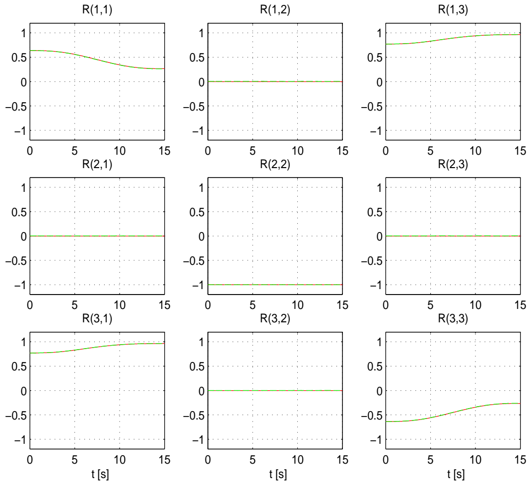
Figura 4.25: Experimento 1. Orientación deseada {}^0\mathbf{R}_d (—) vs orientación real {}^0\mathbf{R}_n (- -).
