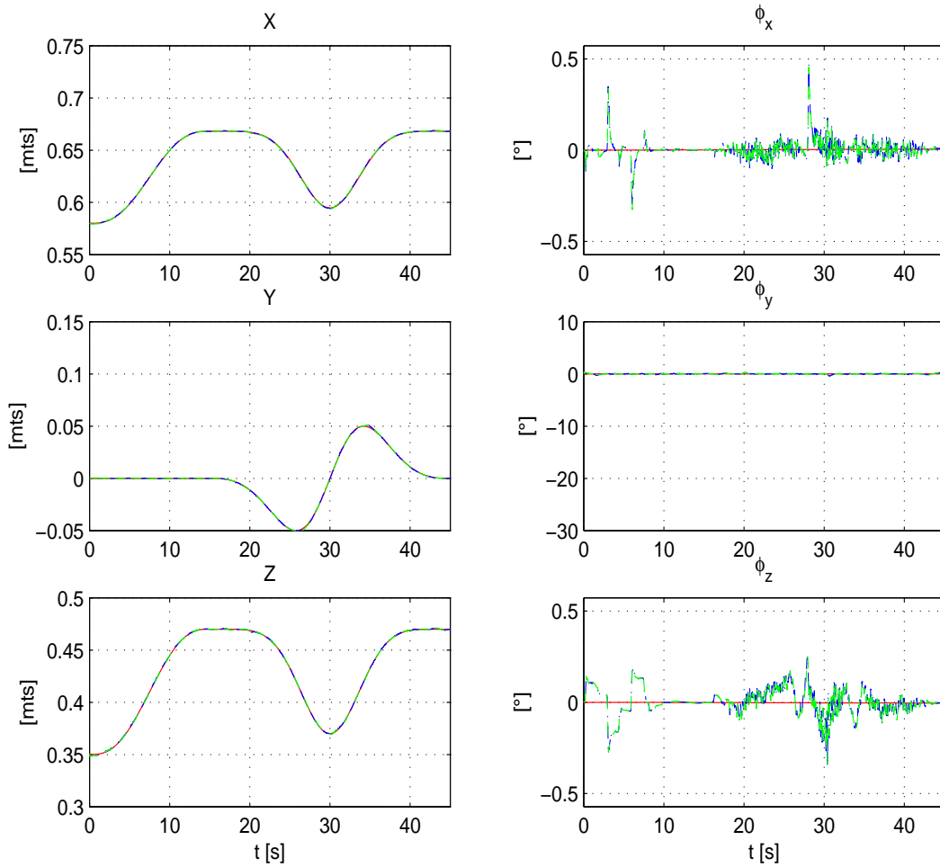
Figura 4.2: Experimento 1. Trayectoria deseada (—) vs trayectoria real (- -) vs trayectoria observada (- · -), de \mathbf{x}=[x \ y \ z \ \phi_x \ \phi_y \ \phi_z]^T .
