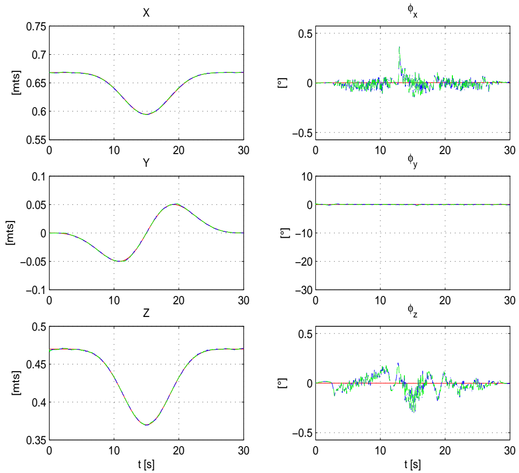
Figura 4.12: Experimento 3. Trayectoria deseada (—) vs trayectoria real (- -) vs trayectoria observada (- · -), de \mathbf{x}=[x \ y \ z \ \phi_x \ \phi_y \ \phi_z]^T .
