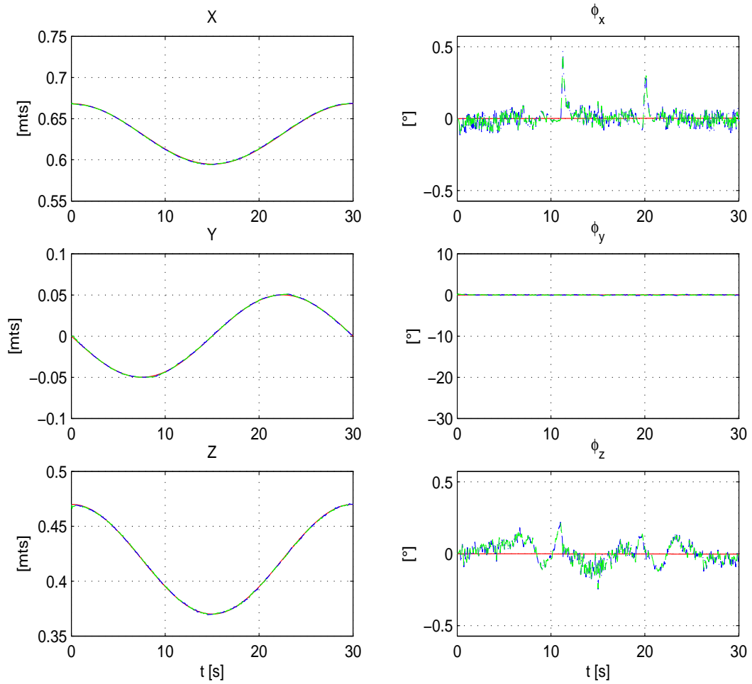
Figura 4.17: Experimento 4. Trayectoria deseada (—) vs trayectoria real (- -) vs trayectoria observada (- · -), de \mathbf{x}=[x \ y \ z \ \phi_x \ \phi_y \ \phi_z]^T .
