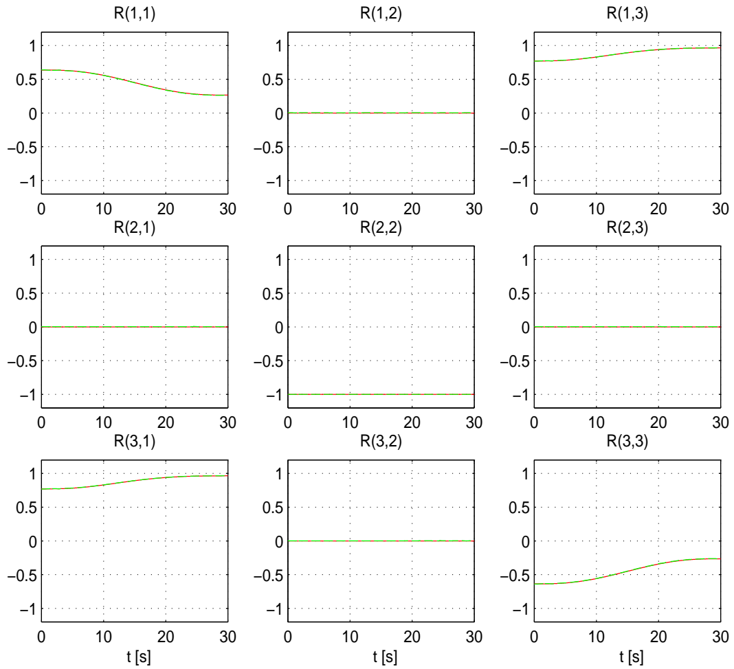
Figura 4.30: Experimento 2. Orientación deseada {}^0R_d (—) vs orientación real {}^0R_n (- -).
