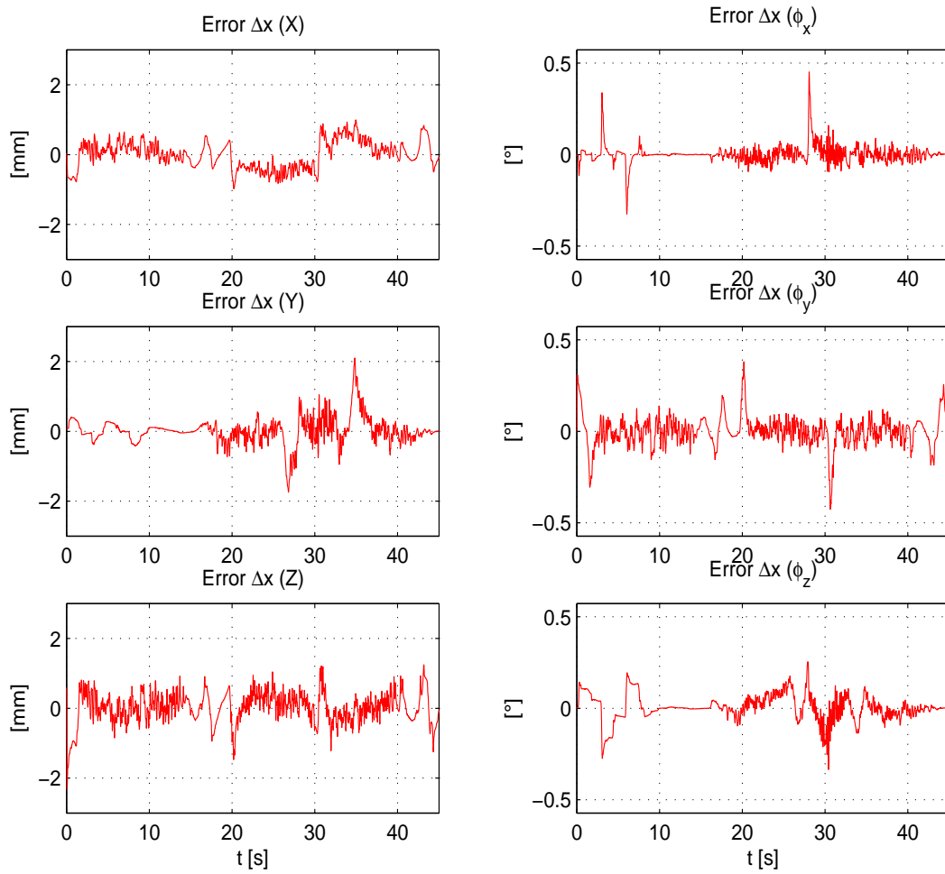
Figura 4.3: Experimento 1. Vector \Delta \mathbf{x} de error de seguimiento ( \mathbf{x} - \mathbf{x}_a ).
