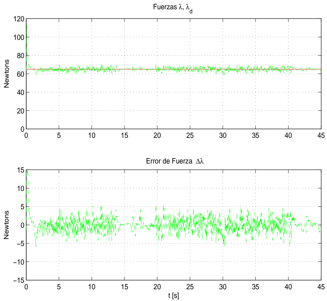
Figura 4.11: Experimento 2. Fuerza deseada \lambda_d (—) vs fuerza real \lambda (- -) y su correspondiente error de seguimiento ( \lambda - \lambda_d ).
