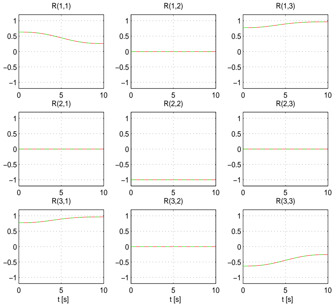
Figura 4.35: Experimento 3. Orientación deseada {}^0\mathbf{R}_d (—) vs orientación real {}^0\mathbf{R}_n (- -).
