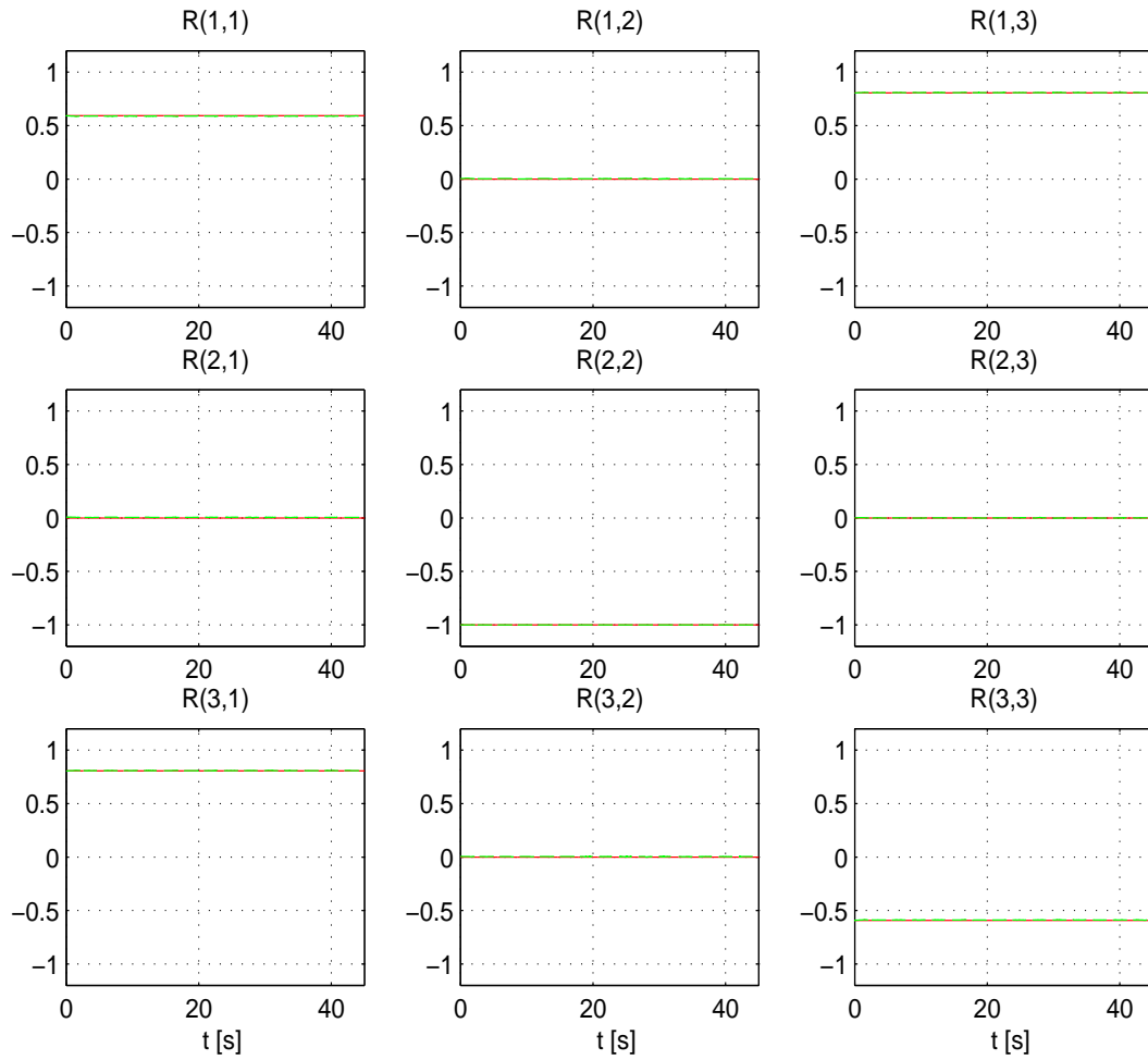
Figura 4.10: Experimento 2. Orientación deseada {}^0\mathbf{R}_d (—) vs orientación real {}^0\mathbf{R}_n (- -).
