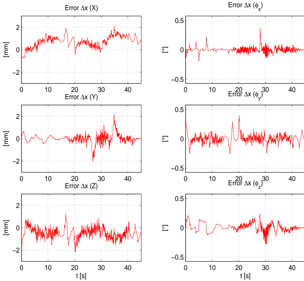
Figura 4.8: Experimento 2. Vector \Delta \mathbf{x} de error de seguimiento ( \mathbf{x} - \mathbf{x}_a ).
