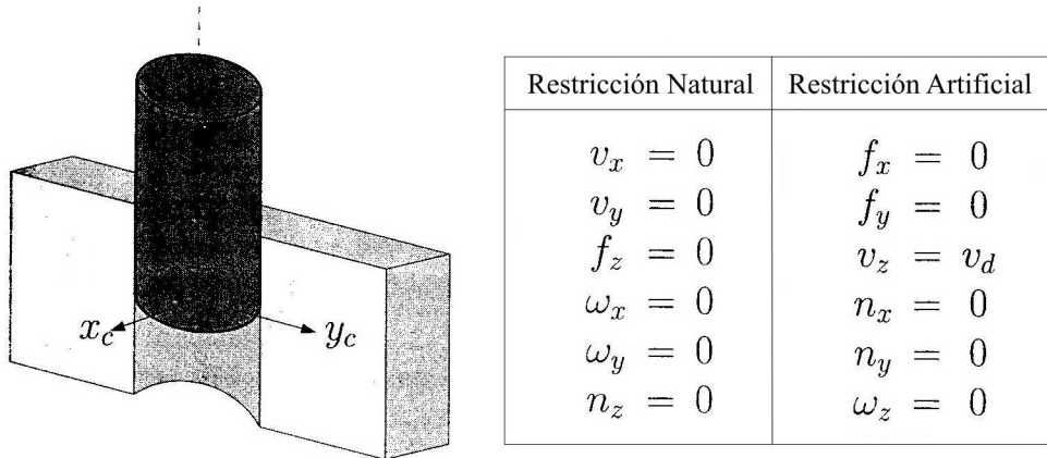
Figura 2.3: Inserción de una barra en un hoyo
