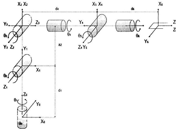
Figura 2.9: Asignación de sistemas de coordenadas del brazo manipulador CRS Robotics A465 .
