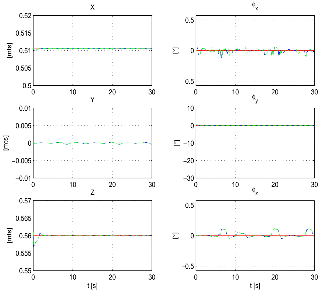
Figura 4.37: Experimento 4. Trayectoria deseada (—) vs trayectoria real (- -) vs trayectoria observada (- · -), de \mathbf{x}=[x \ y \ z \ \phi_x \ \phi_y \ \phi_z]^T .
