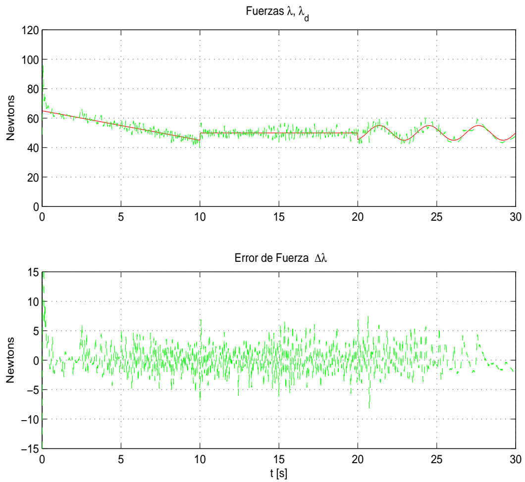
Figura 4.31: Experimento 2. Fuerza deseada \lambda_d (—) vs fuerza real \lambda (- -) y su correspondiente error de seguimiento ( \lambda - \lambda_d ).
