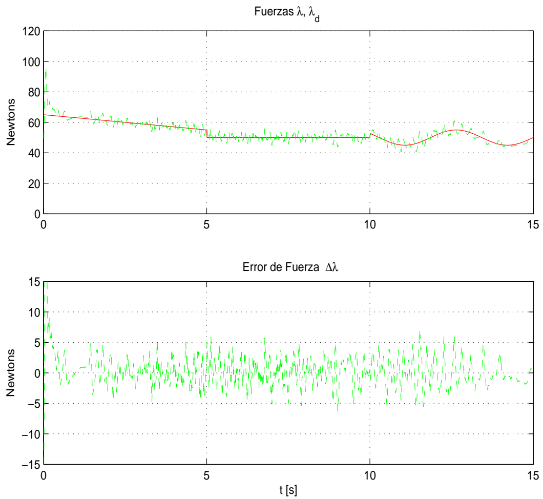
Figura 4.26: Experimento 1. Fuerza deseada \lambda_d (—) vs fuerza real \lambda (- -) y su correspondiente error de seguimiento ( \lambda - \lambda_d ).
