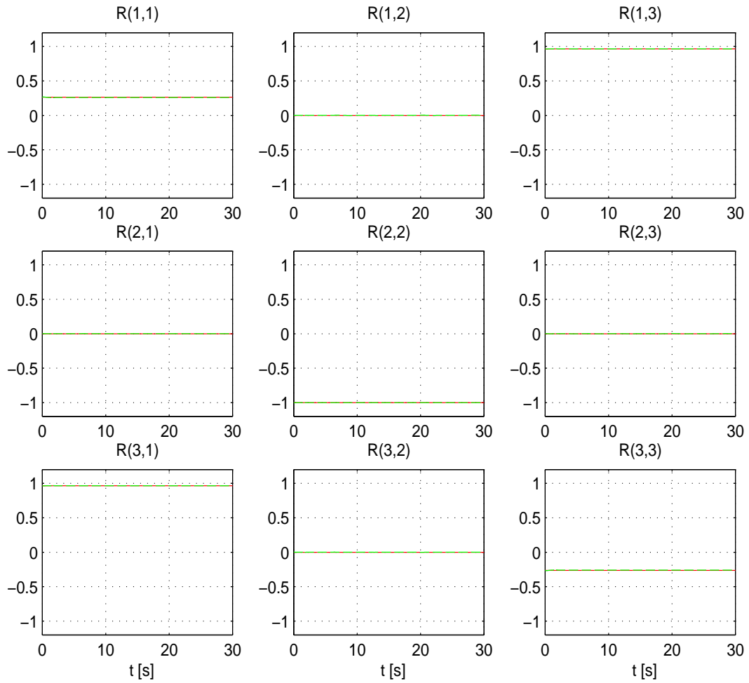
Figura 4.40: Experimento 4. Orientación deseada {}^0\mathbf{R}_d (—) vs orientación real {}^0\mathbf{R}_n (- -).
