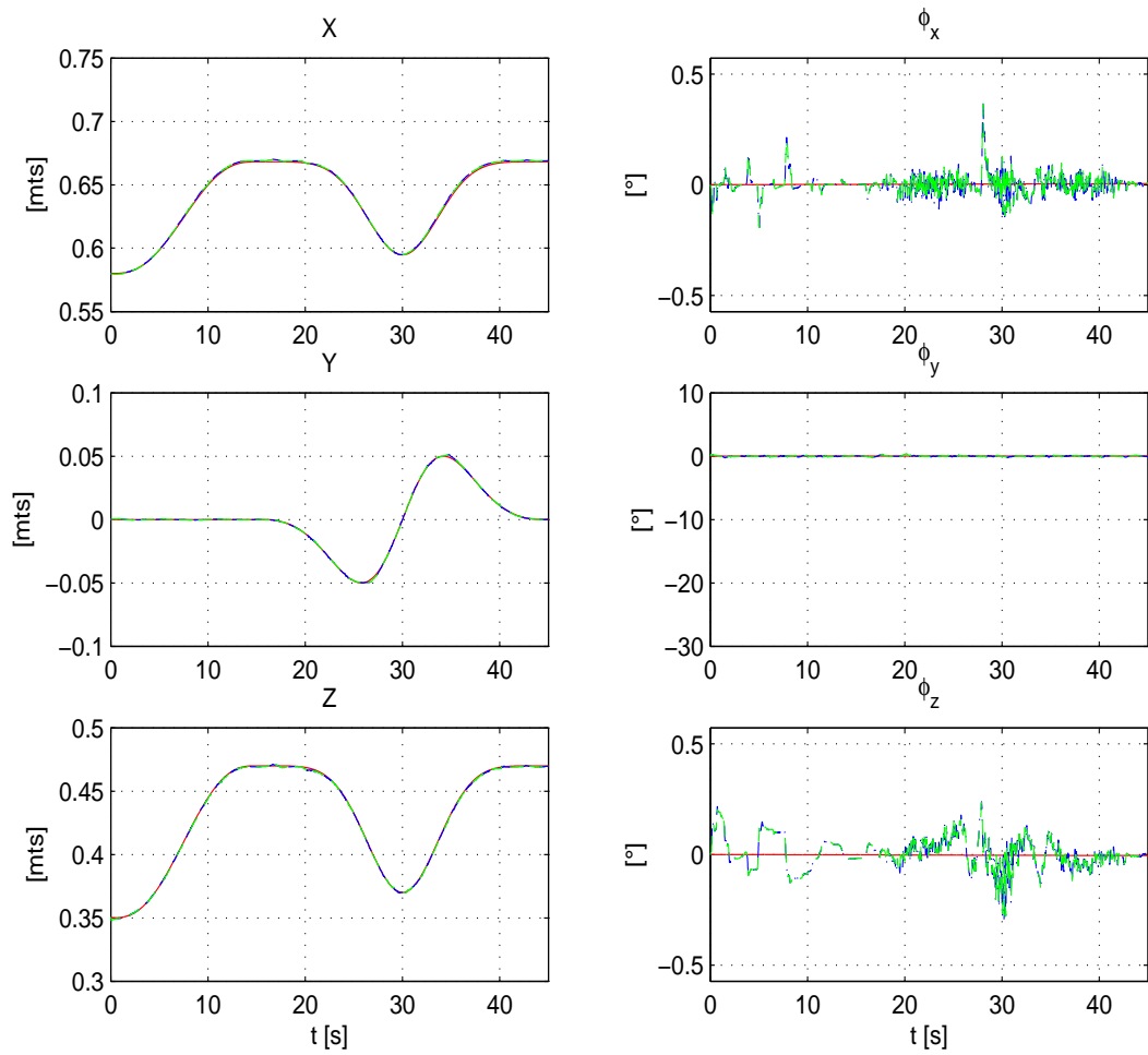
Figura 4.7: Experimento 2. Trayectoria deseada (—) vs trayectoria real (- -) vs trayectoria observada (- · -), de \mathbf{x}=[x \ y \ z \ \phi_x \ \phi_y \ \phi_z]^T .
