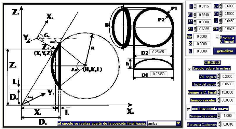
Figura B.11: Diagrama de superficie esférica con parámetros
