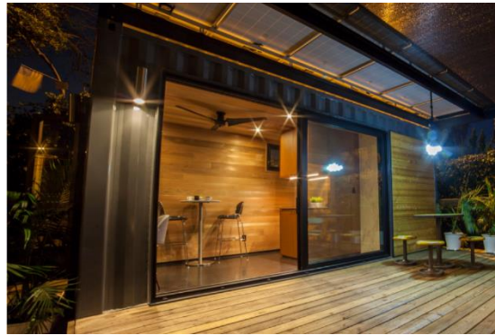
Figura 16. Vista exterior del Modelo NOS1 terminado. (New Old Stock, 2016).
