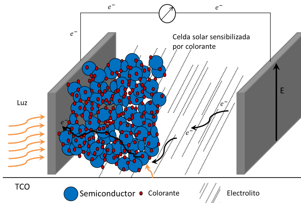
Figura 2.14 Esquema de una celda solar sensibilizada con colorante, se observan sus principales componentes como el colorante, el semiconductor, vidrios conductores y electrolito, que juntos transforman los fotones en corriente eléctrica.
