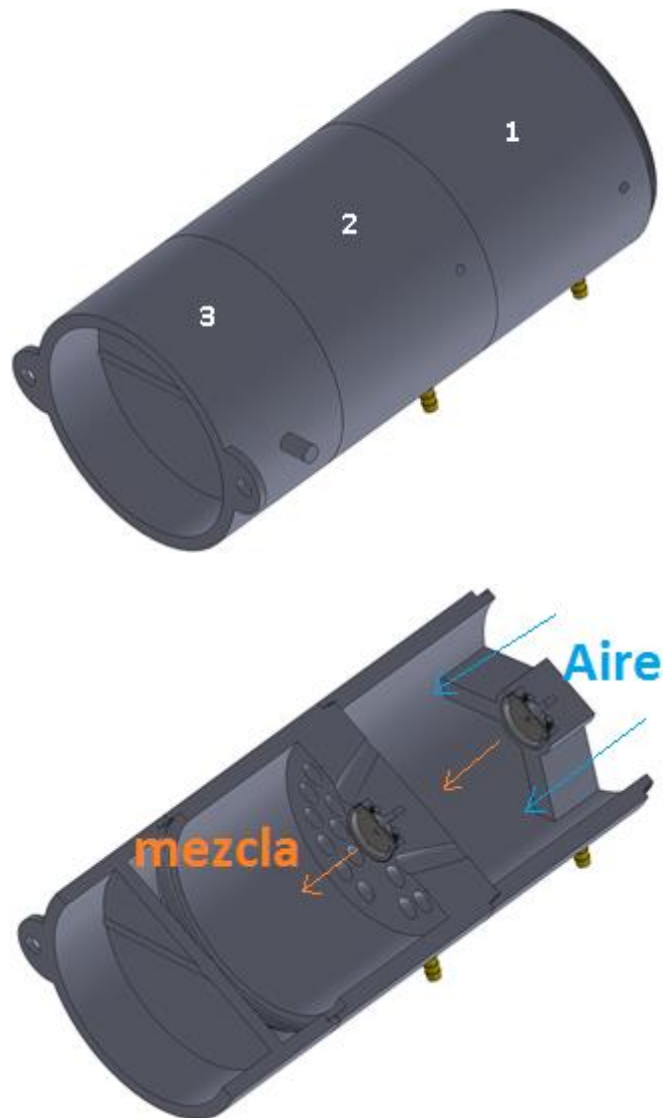
Figura 55. Tres piezas del diseño las piezas 1 y 2 sujetan un transductor ultrasónico cada uno y la pieza 3 regula la entrada de mezcla (superior), ensamble del diseño mostrado con un corte a la mitad (inferior).
