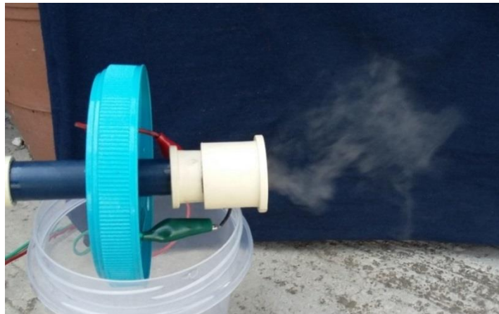
Figura 50. Funcionamiento del prototipo.
