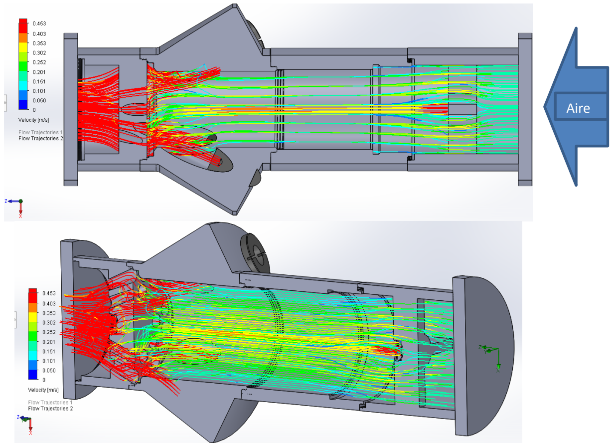
Figura 62. Simulación del ensamble del inyector con líneas.
