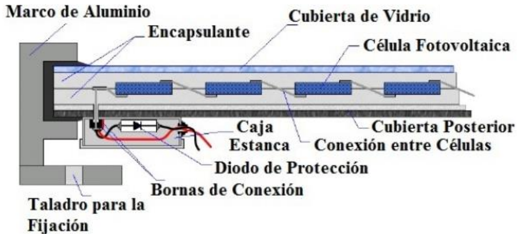
Figura 36. Estructura de un panel fotovoltaico Recuperado de: http://ingemecanica.com
