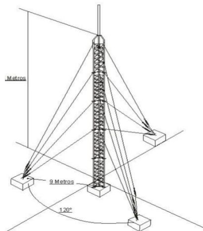
Figura 64. Diseño de la torre de comunicación. Recuperado de: Anexo III, Torres y mástiles de telecomunicaciones y radiodifusión.
