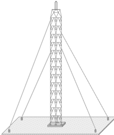
Figura 62. Diseño de una torre arriostrada.
