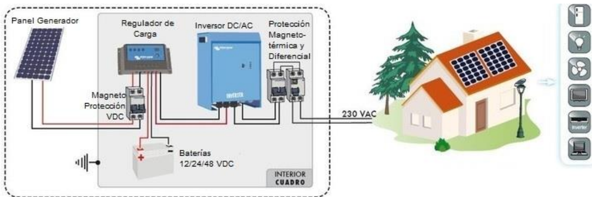
Figura 35: Kit de sistema fotovoltaico aislado. Recuperado de: http://ingemecanica.com
