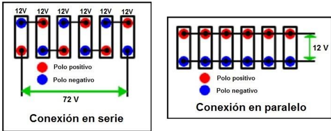
Figura 40. Diferencia entre conexión serie y conexión paralela. Recuperado de: http://ingemecanica.com
