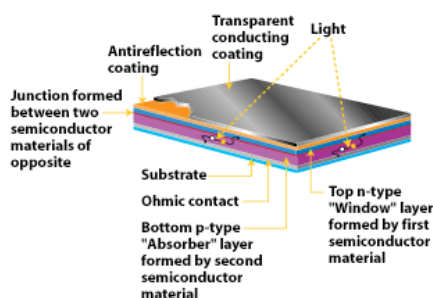
Figura 31. Capas de una celda solar Recuperado de: http://www.cenitsolar.com/fotovoltaica_esquema.php
