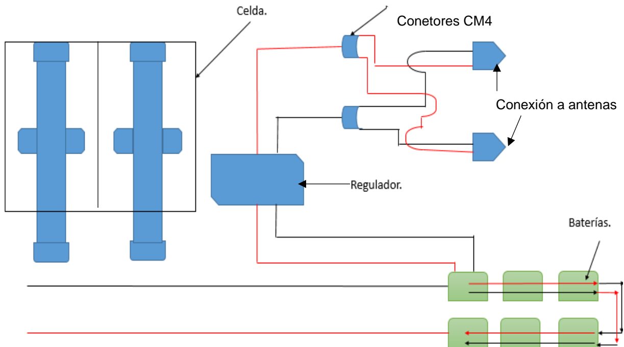
Figura 51. Arreglo del sistema de alimentación por medio de celdas fotovoltaicas. Recuperado de: Diseño propio en colaboración con Telecomunicaciones Indígenas Comunitarias.
