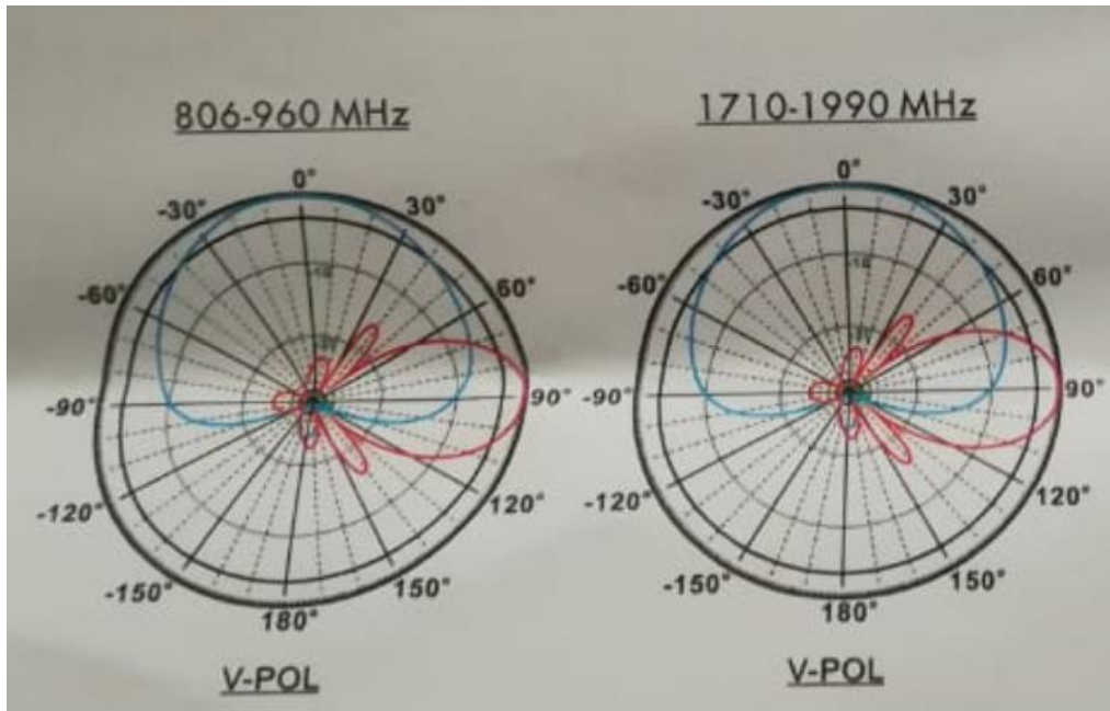
Figura 58. Diagrama de Radiación Recuperado de: Catalogo Texas Engineered, 2012.
