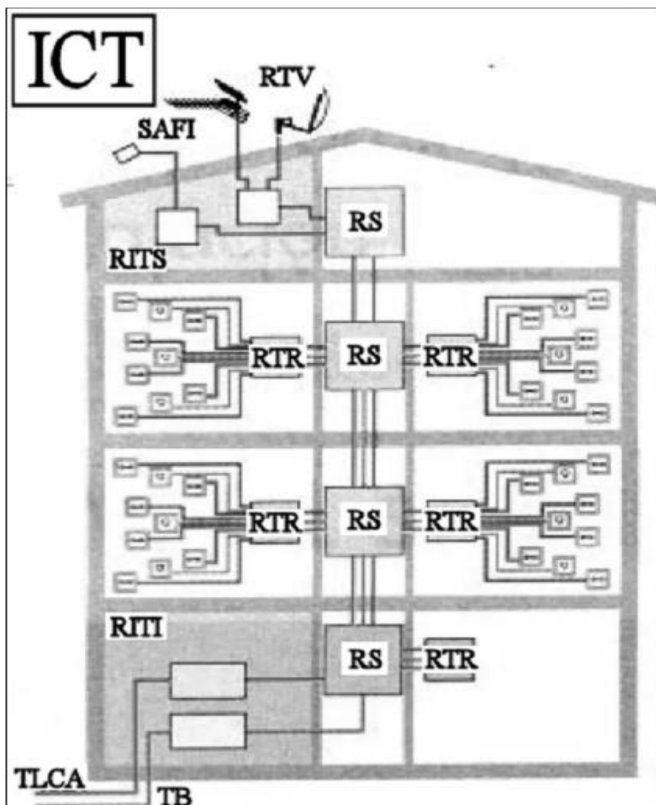
Figura 2. Diagrama de ICT y RITIS
