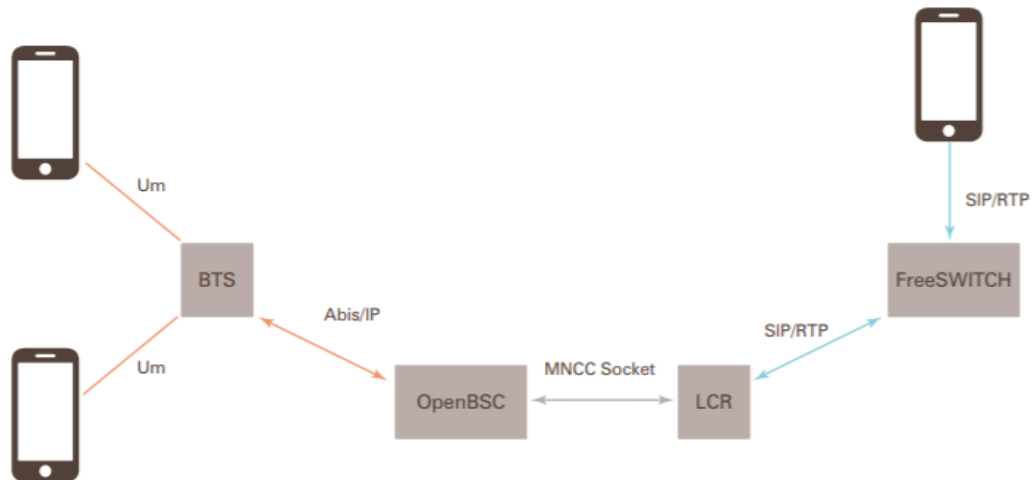
Figura 19. Cadena de tecnología de Telefonía Celular Comunitaria. Recuperado de: Manual de telefonía Celular Comunitaria (2017).
