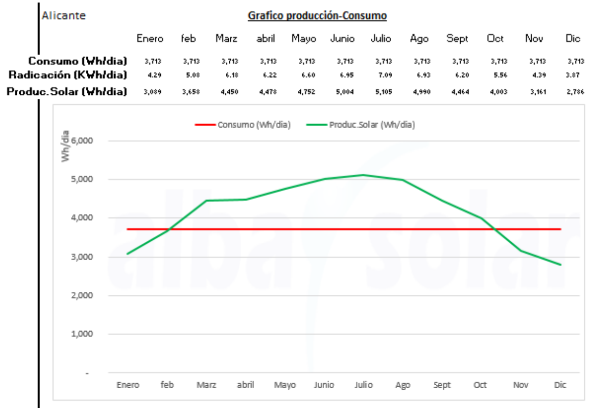
Figura 84. Gráfica de eficiencia del sistema de alimentación. Recuperado de: Creación Propia.
