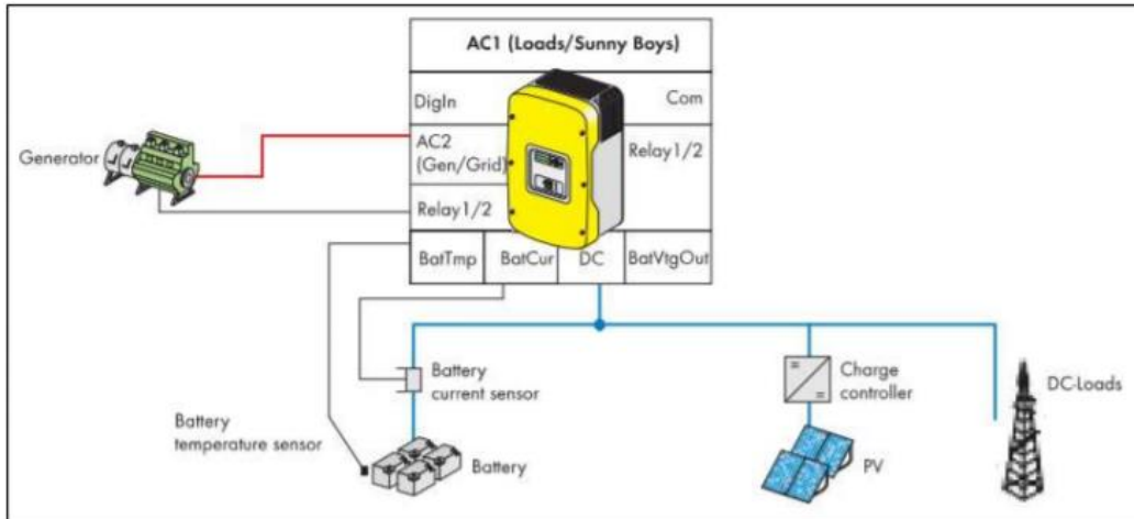
Figura 50. Esquema del circuito híbrido alimentado por diesel y celdas fotovoltaicas.
