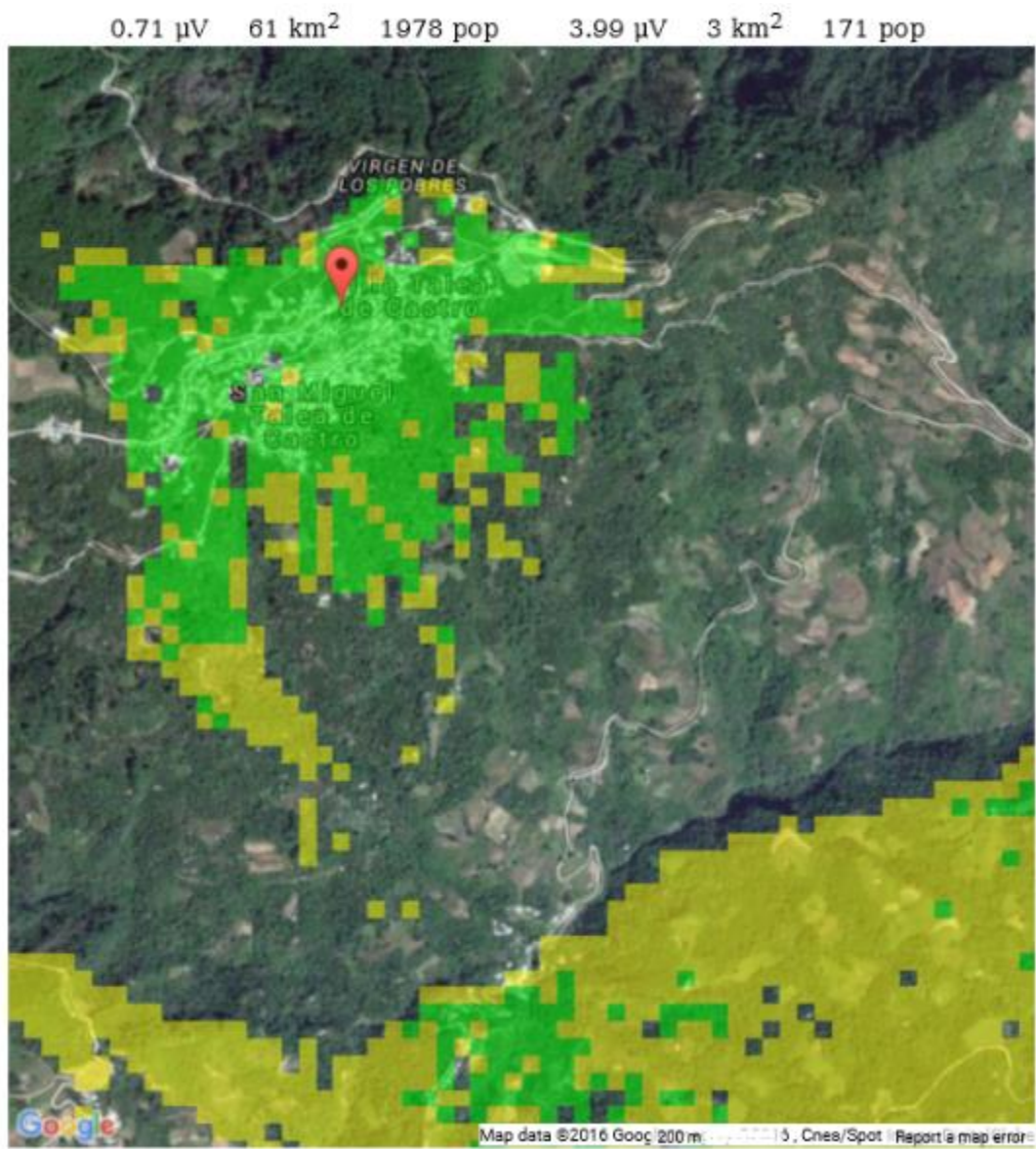
Figura 22. Mapa de Cobertura de Talea de Castro en Radio Mobile. Recuperado de: Simulación realizada en el software Radio Mobile .
