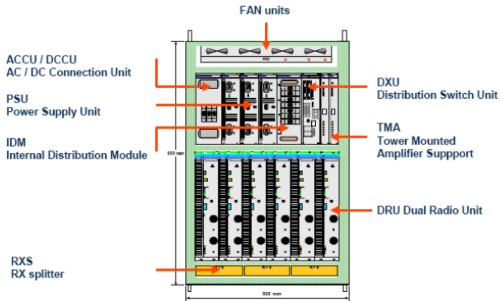
Figura 44. Cabina RBS Ericsson 2116 Recuperado de: Universidad Carlos III de Madrid. Tesis Madrid sobre sistema de alimentación fotovoltaico.
